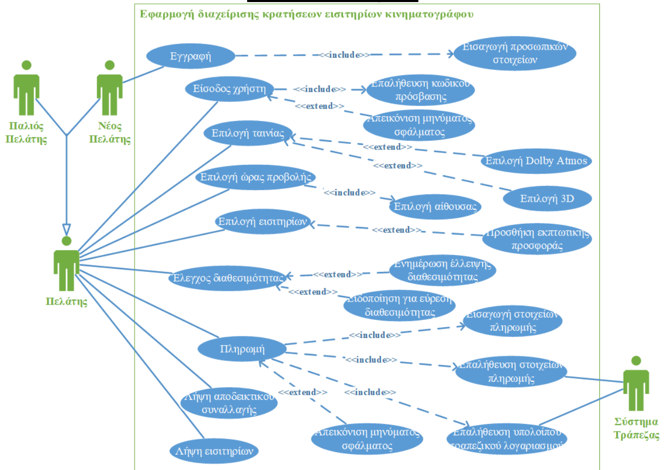
Εικόνα 5.1.1. Διάγραμμα Use case εφαρμογής διαχείρισης κρατήσεων εισιτηρίων κινηματογράφου
