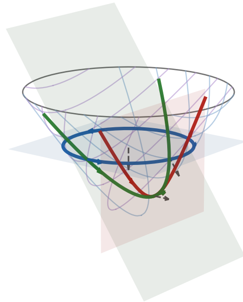
(d) 3D Cone
