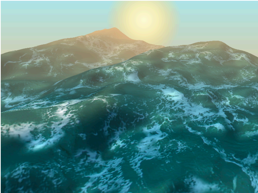
Figura 8: Resultado combinado: espectro realista por bandas, espuma aditiva sobre las crestas y niebla atmosférica que funde el borde del disco con el cielo. La malla en disco elimina las esquinas del plano y da la sensación de mar abierto.
