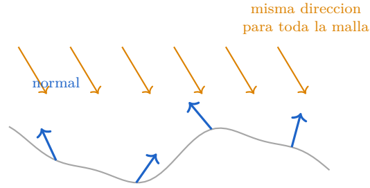
Figura 3: Luz direccional: el vector hacia la luz (naranja) es idéntico para toda la malla, como rayos de sol paralelos. La normal (azul) sí cambia en cada vértice según la inclinación local de la ola. El resultado de la iluminación difusa/especular varía de un punto a otro únicamente porque cambia la normal, no la dirección de la luz.
