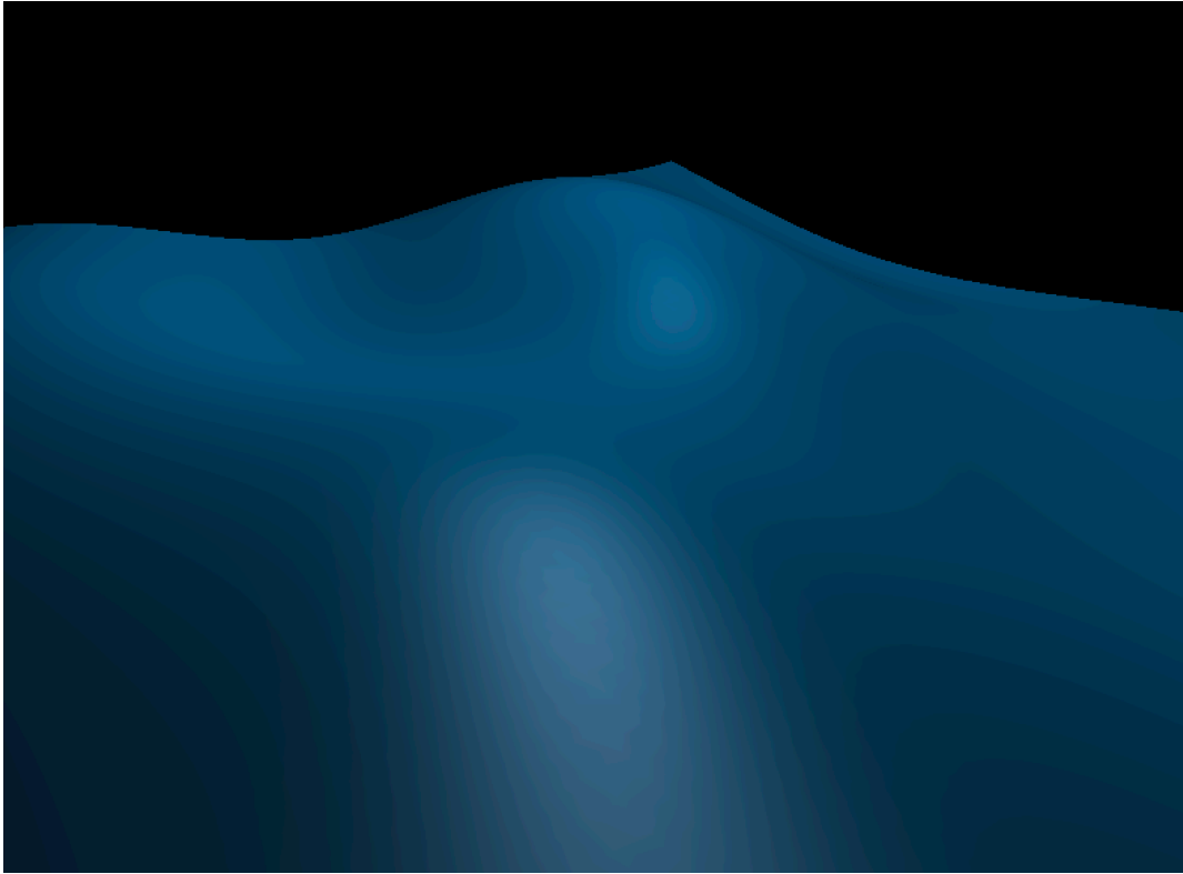
Figura 4: Océano con geometría e iluminación, sin textura (capturado desactivando temporalmente glEnable(GL_TEXTURE_2D) en Ocean::draw() ). Se distinguen dos manchas de brillo especular: una grande en el centro y otra más pequeña arriba a la derecha, cada una sobre una cresta distinta de la superficie.
