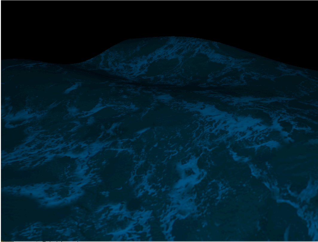
Figura 5: Océano con textura, normales e iluminación combinadas. La forma general de las olas la aporta la geometría (la malla deformada por update() ); el detalle fino de espuma y reflejos lo aporta la textura ( ocean.tga ); y el contraste entre la cresta iluminada y los valles en sombra lo aporta la iluminación , que usa las normales calculadas por computeNormals() para saber cuánta luz recibe cada punto de la superficie.
