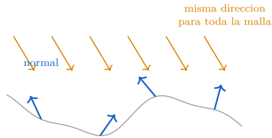
Figura 3: Luz direccional: el vector hacia la luz (naranja) es idéntico para toda la malla, como rayos de sol paralelos. La normal (azul) sí cambia en cada vértice según la inclinación local de la ola. El resultado de la iluminación difusa/especular varía de un punto a otro únicamente porque cambia la normal, no la dirección de la luz.
