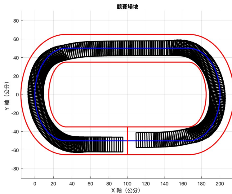
圖 57: 初始偏差為 -4cm 之車輛移動路徑模擬圖
