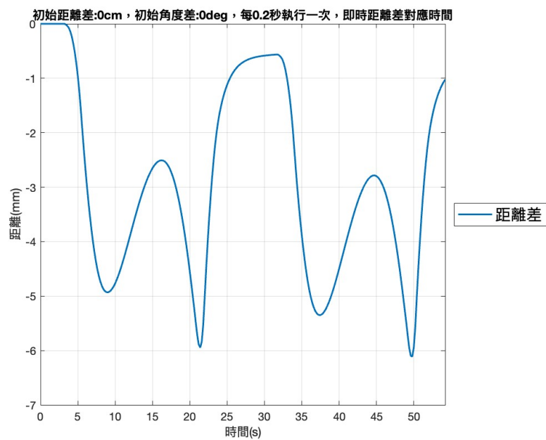
圖 42: 車輛與標線距離差對應時間圖
