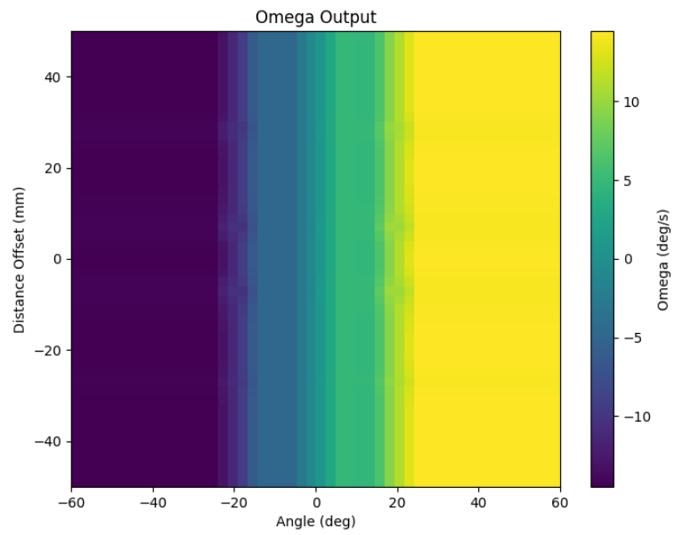
圖 24: 不同偏差角度及偏移量對應之角速度 \omega
