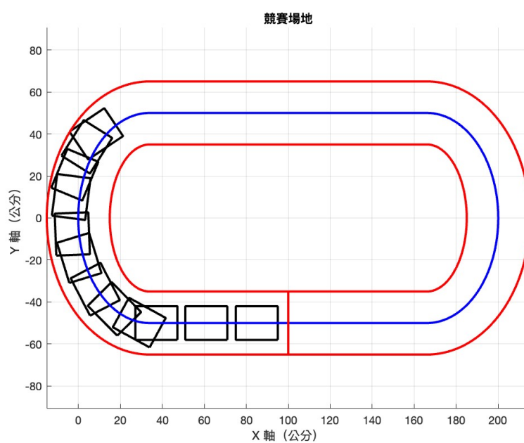
圖 46: 每 2 秒控制一次之車輛移動路徑模擬圖
