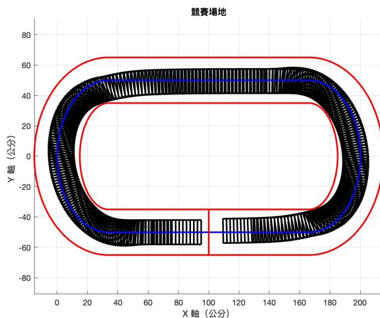
圖 38: 車輛路徑模擬圖
