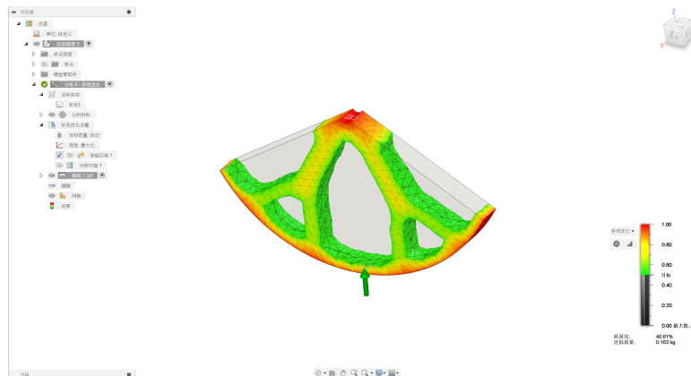
圖 61: 輪椅大輪的形狀優化 2
