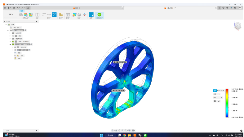
圖 64: 輪椅大輪的應力分析
