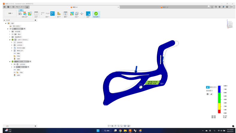
圖 67: 輪椅側板的安全係數分析
