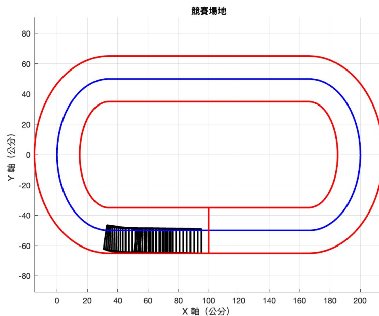
圖 59: 初始偏差為-7cm 之車輛移動路徑模擬圖
