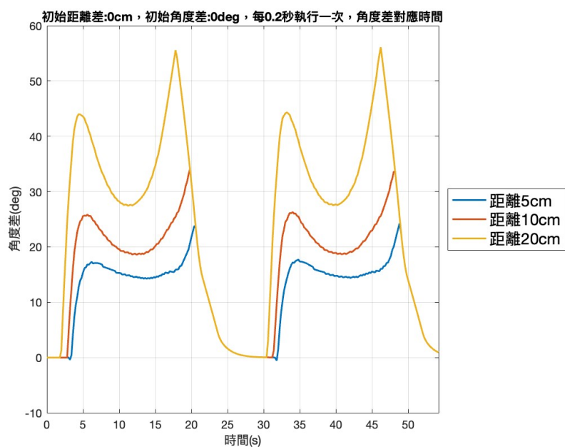
圖 44: 車輛偵測標線角度差對應時間圖
