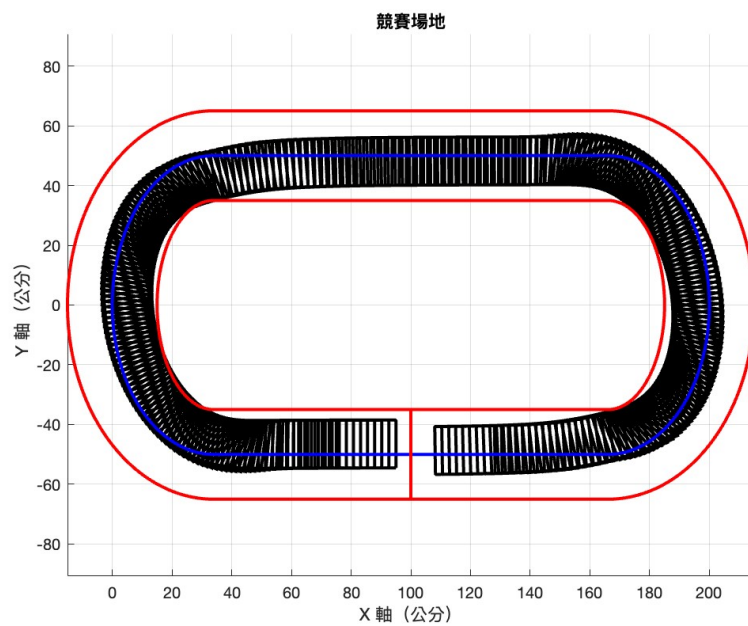
圖 55: 初始偏差為 3.5cm 之車輛移動路徑模擬圖
