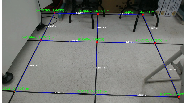
圖 27: 實際測量地板尺寸
