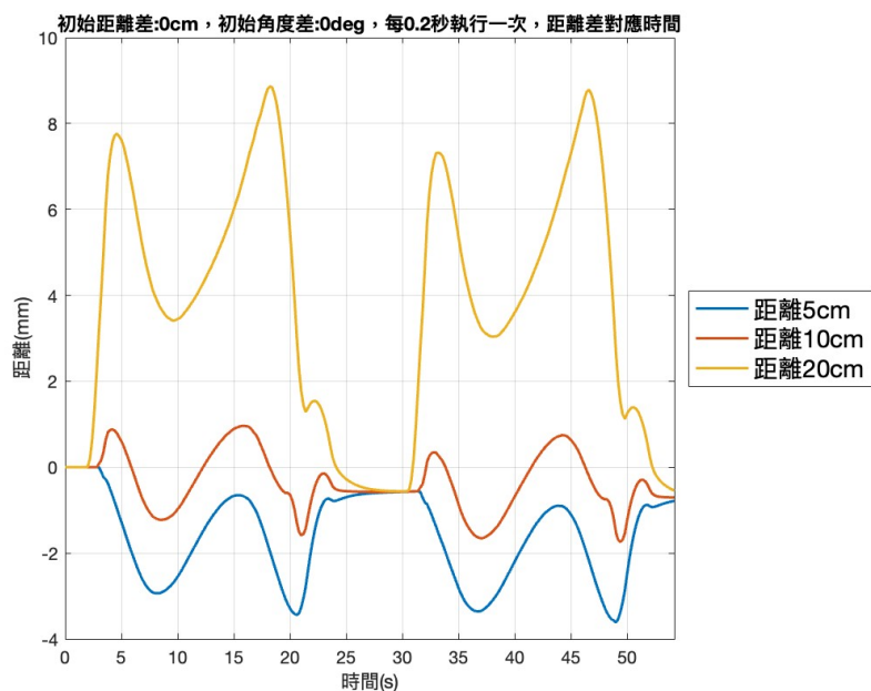
圖 43: 車輛偵測標線距離差對應時間圖
