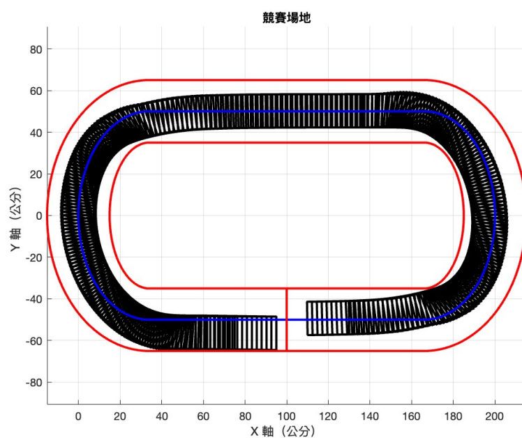
圖 58: 初始偏差為 -6.5cm 之車輛移動路徑模擬圖
