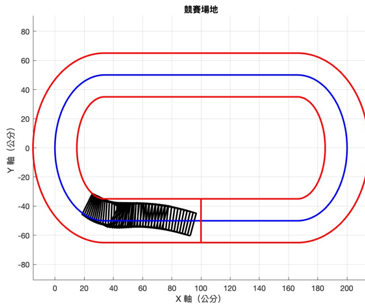
圖 48: 初始角度為 15 度之車輛移動路徑模擬圖
