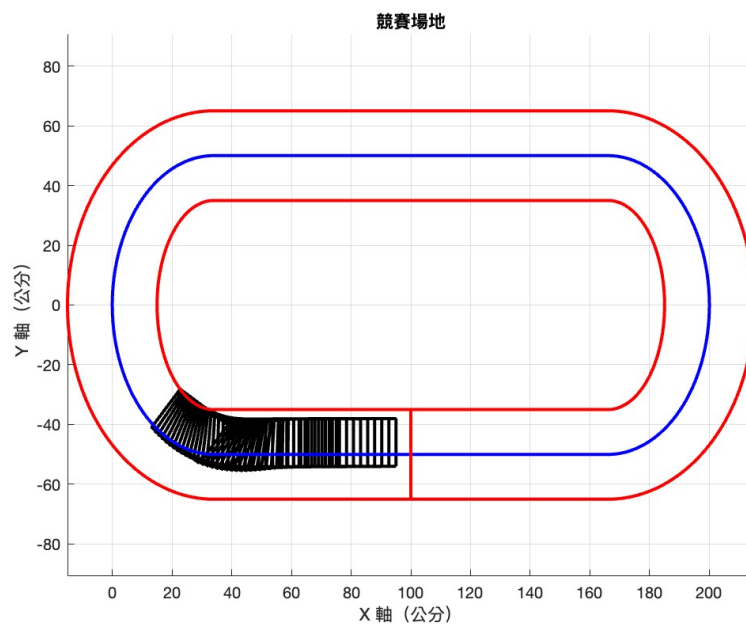
圖 54: 初始偏差為 4cm 之車輛移動路徑模擬圖
