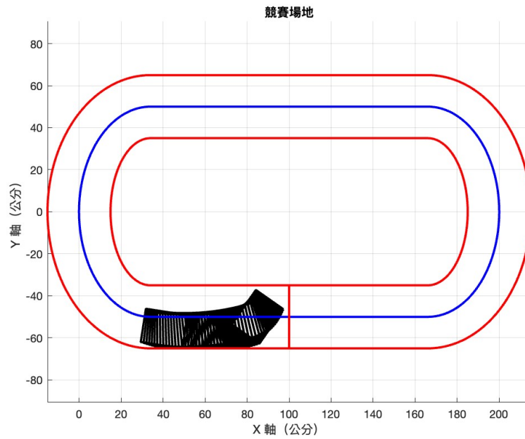
圖 53: 初始角度為-55 度之車輛移動路徑模擬圖
