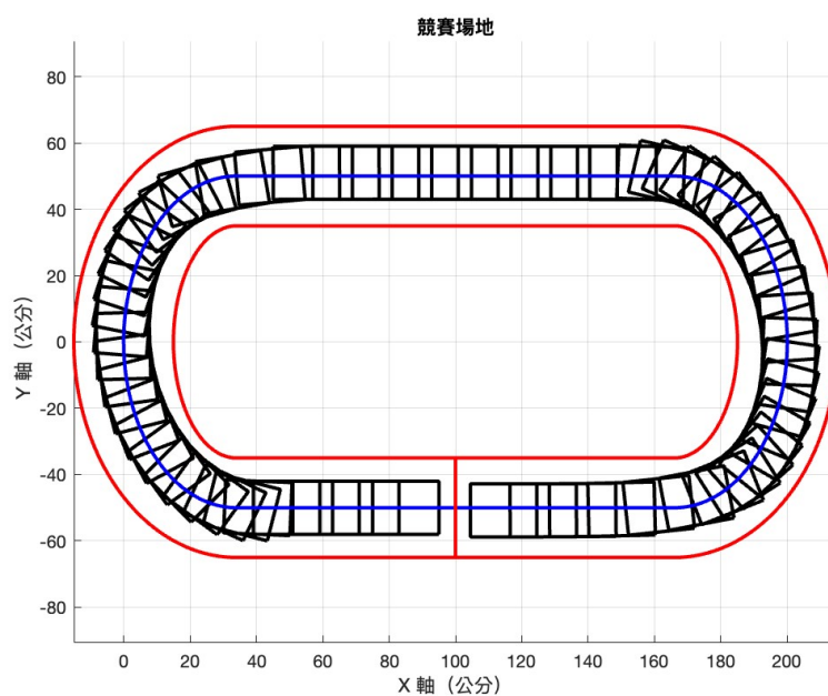
圖 45: 每 1 秒控制一次之車輛移動路徑模擬圖
