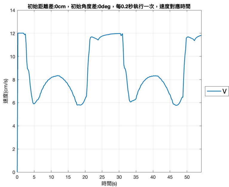
圖 39: 車輛速度對應時間圖
