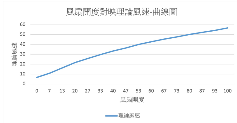
圖 71: 風扇開度對應理論風速曲線圖
