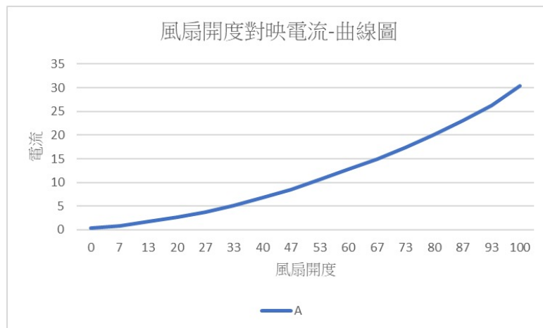
圖 72: 風扇開度對應電流曲線圖
