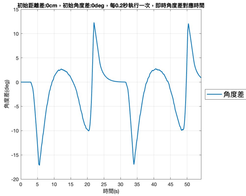
圖 41: 車輛與標線角度差對應時間圖
