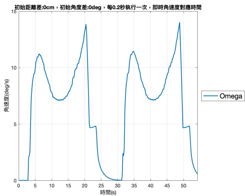
圖 40: 車輛速度對應角速度時間圖
