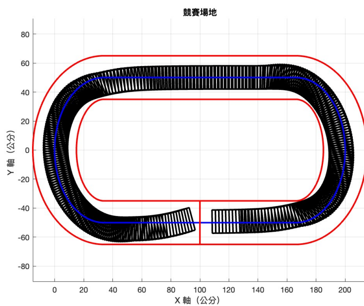
圖 54: 初始角度為-15 度之車輛移動路徑模擬圖
