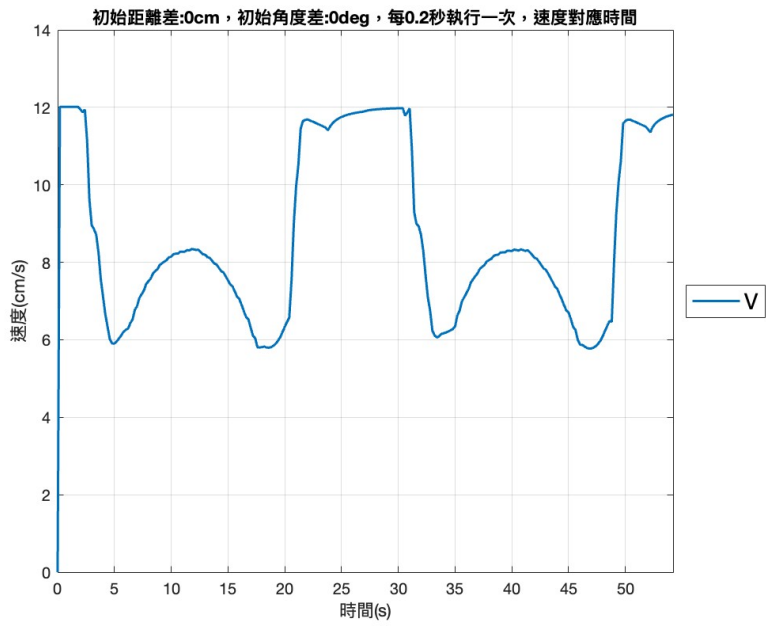
圖 43: 車輛速度對應時間圖
