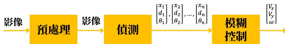
圖 8: 影像循線演算法流程圖
