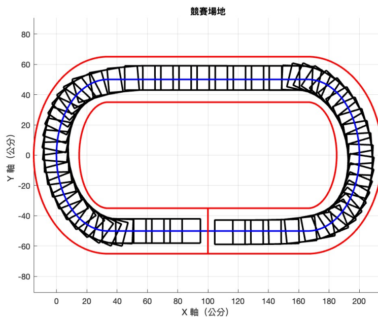
圖 49: 每 1 秒控制一次之車輛移動路徑模擬圖
