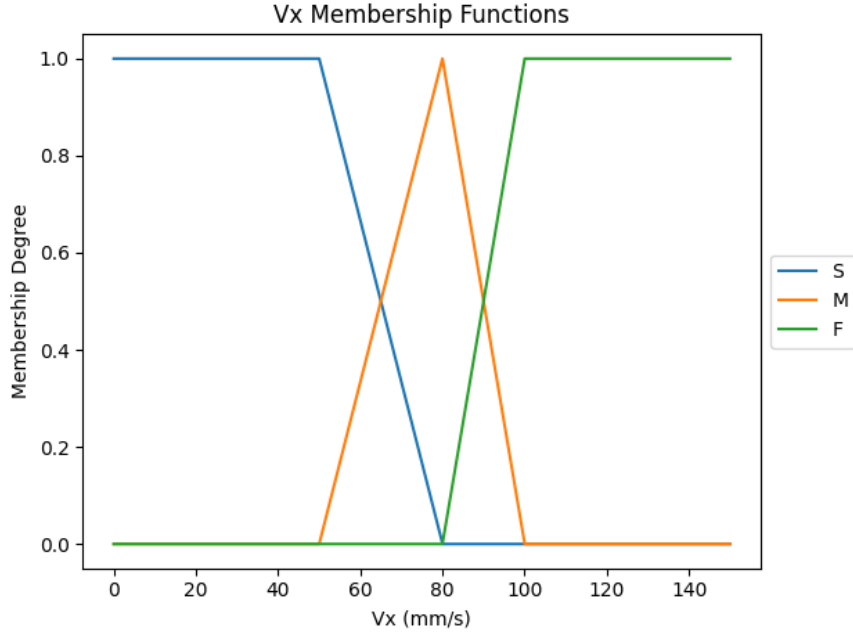
圖 21: 前進速度 V_x 隸屬函數
