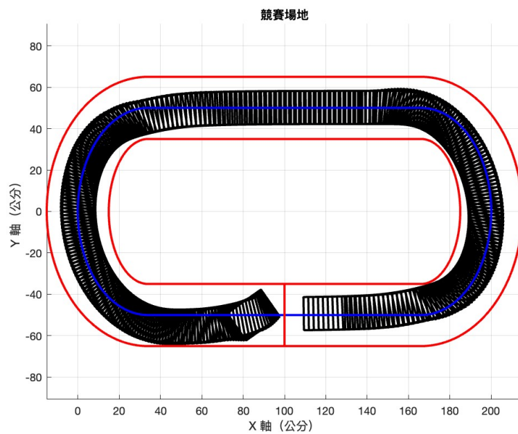
圖 55: 初始角度為-35 度之車輛移動路徑模擬圖
