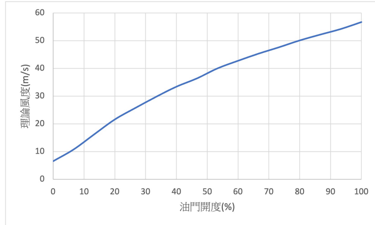
圖 76: 風扇開度對應理論風速曲線圖
