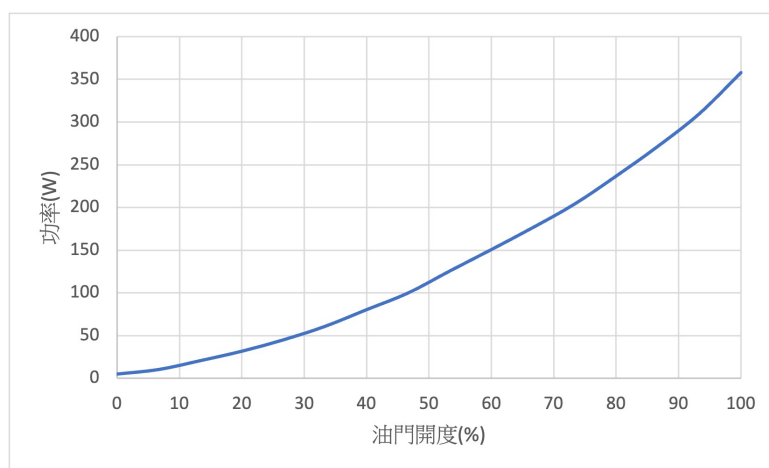
圖 78: 風扇開度對應功率曲線圖
