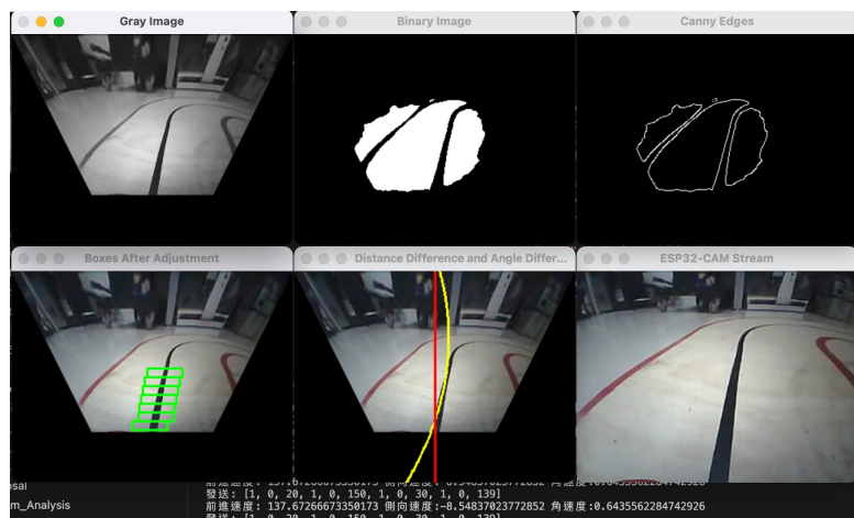
圖 39: 車輛靜止時影像處理與模糊控制之結果(出彎)
