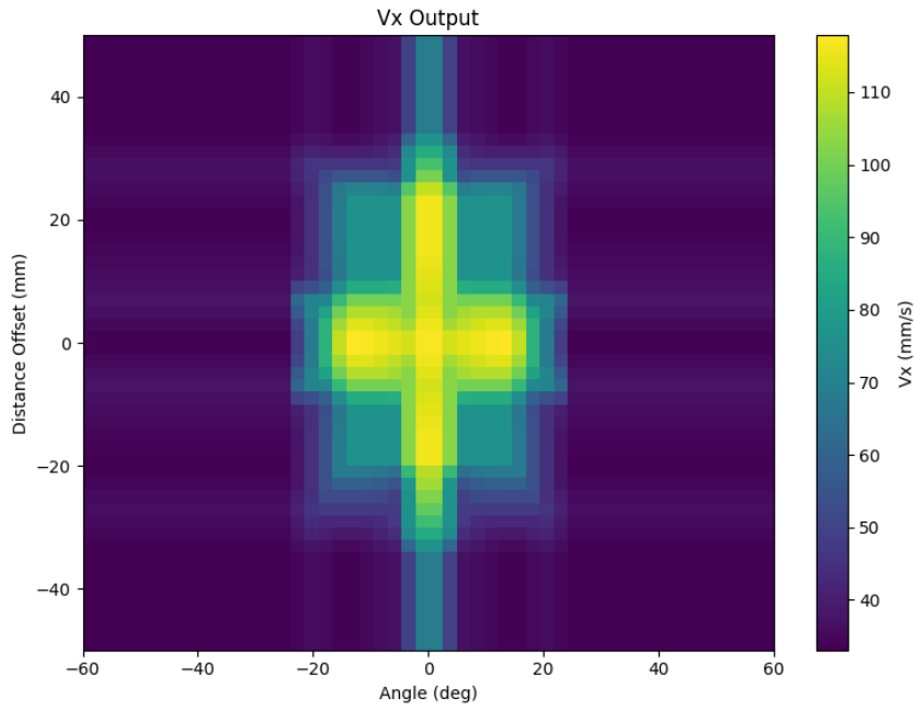
圖 24: 不同偏差角度及偏移量對應之前進速度 V_x
