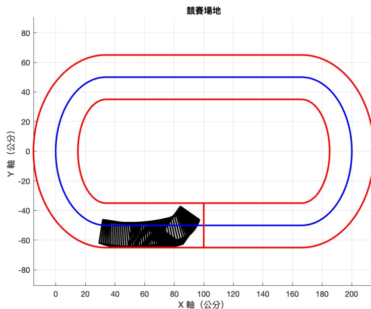
圖 57: 初始角度為-55 度之車輛移動路徑模擬圖
