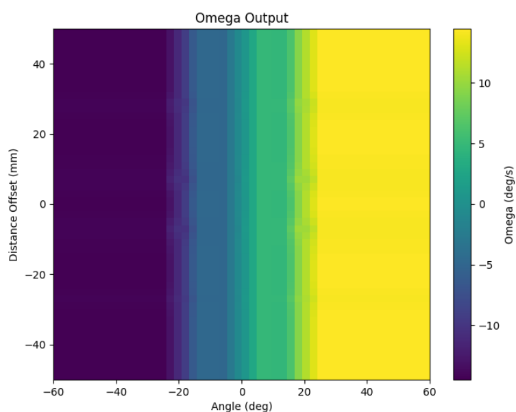
圖 25: 不同偏差角度及偏移量對應之角速度 \omega
