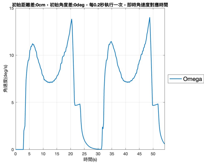
圖 44: 車輛速度對應角速度時間圖
