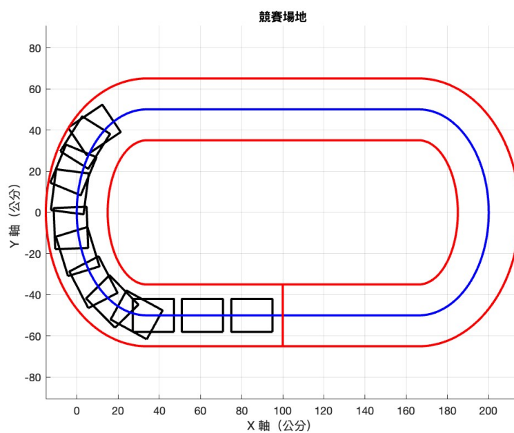
圖 50: 每 2 秒控制一次之車輛移動路徑模擬圖
