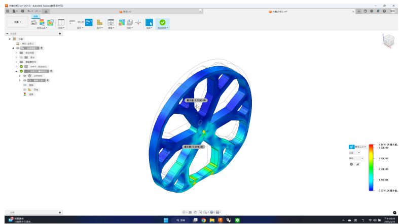
圖 68: 輪椅大輪的應力分析
