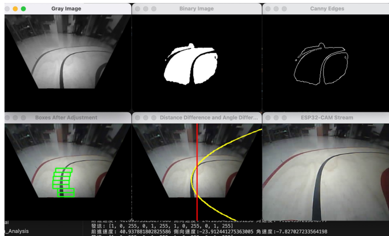
圖 38: 車輛靜止時影像處理與模糊控制之結果(入彎)
