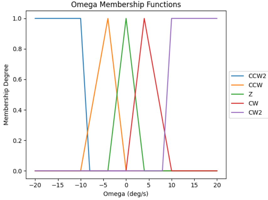
圖 23: 角速度 \omega 隸屬函數
