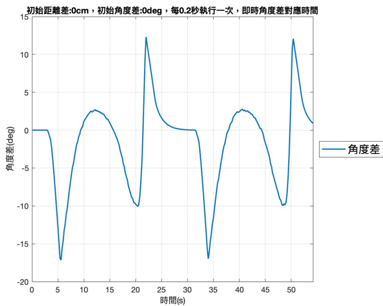
圖 45: 車輛與標線角度差對應時間圖
