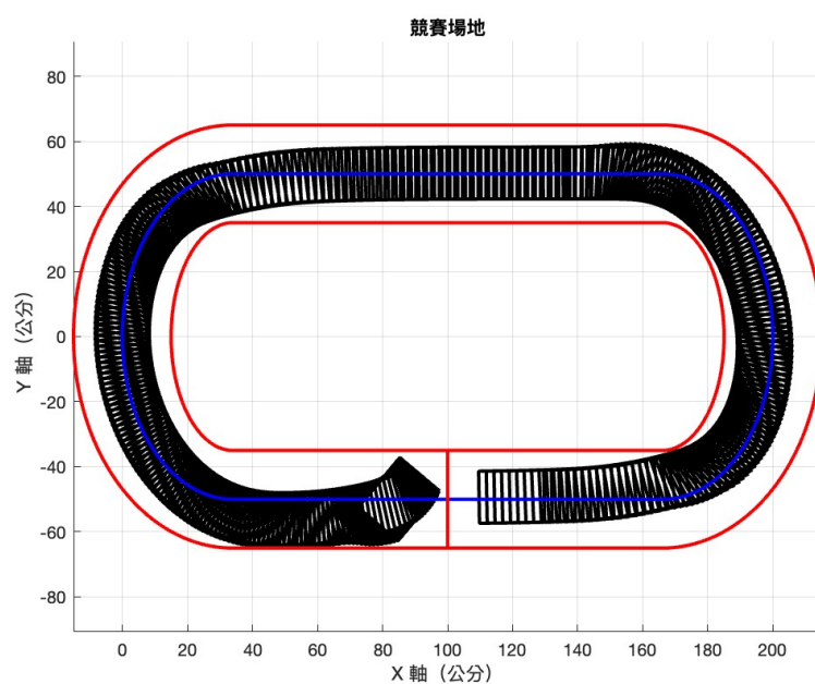
圖 56: 初始角度為-50 度之車輛移動路徑模擬圖
