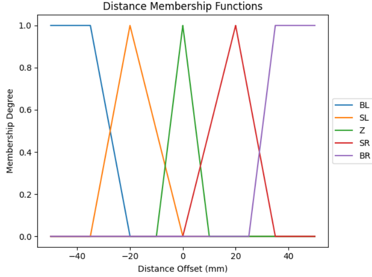
圖 20: 位置偏移量 distance(mm) 隸屬函數
