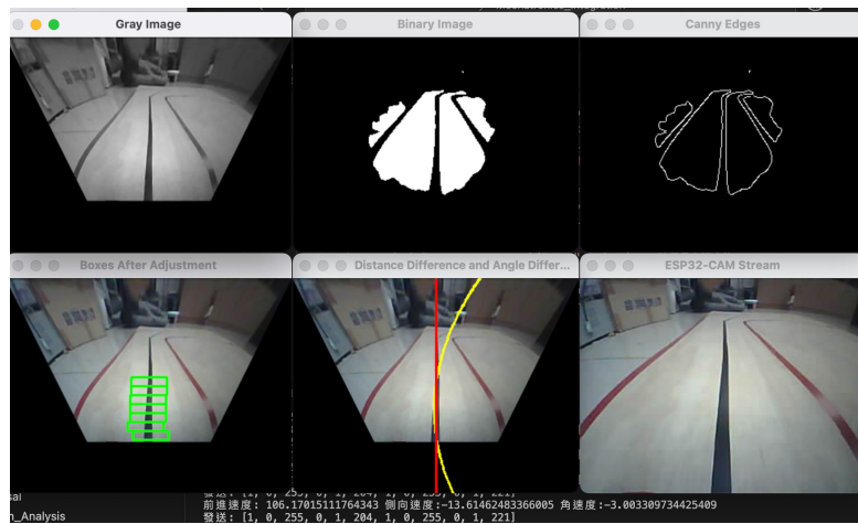
圖 37: 車輛靜止時影像處理與模糊控制之結果(直線)
