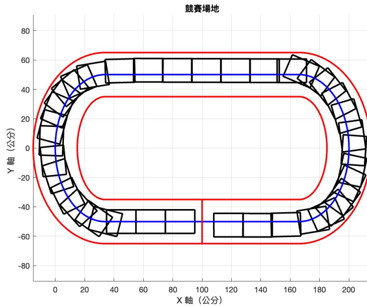
圖 51: 每 1.7 秒控制一次之車輛移動路徑模擬圖
