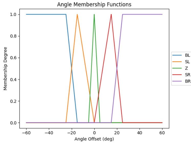
圖 19: 偏差角度 \text{angle}(\theta) 隸屬函數
