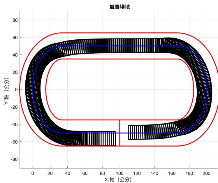
圖 62: 初始偏差為 -6.5cm 之車輛移動路徑模擬圖
