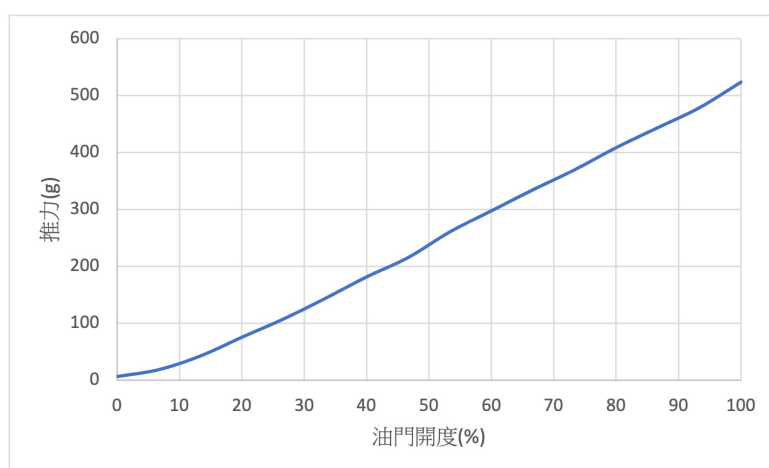
圖 79: 風扇開度對應推力曲線圖
