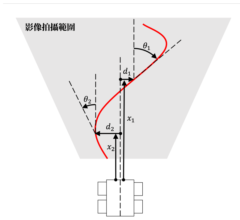
圖 18: 辨識前方偏移量和偏移角度示意圖
