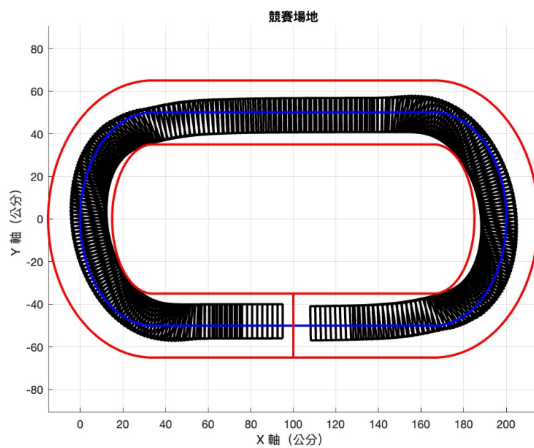
圖 60: 初始偏差為 2\text{cm} 之車輛移動路徑模擬圖
