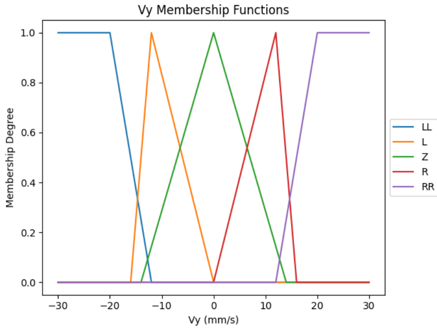
圖 22: 側向數度 V_y 隸屬函數
