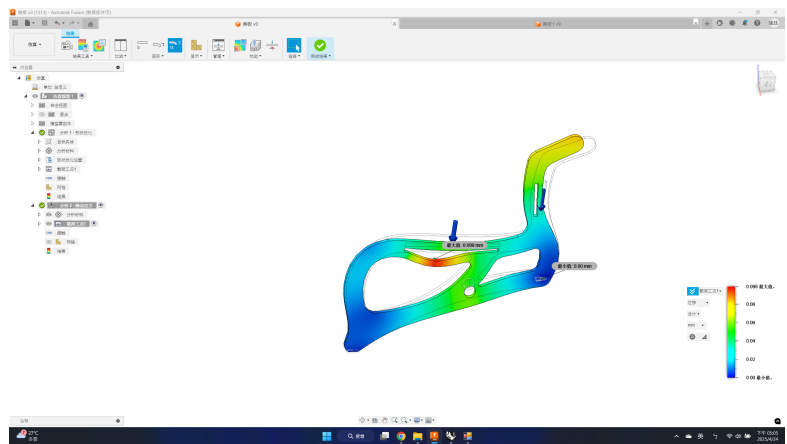
圖 70: 輪椅側板的位移分析
