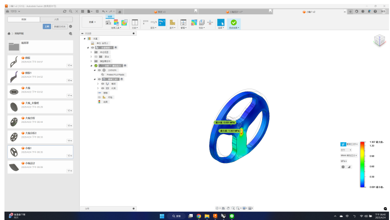
圖 73: 小輪的應力分析
