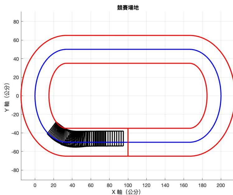
圖 58: 初始偏差為 4cm 之車輛移動路徑模擬圖
