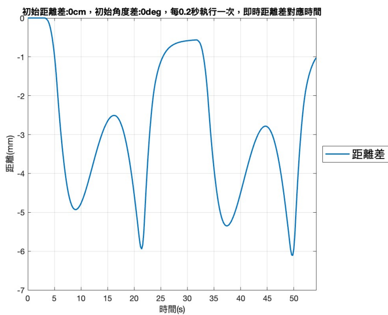
圖 46: 車輛與標線距離差對應時間圖
