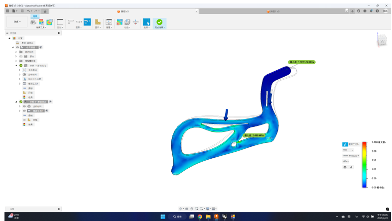
圖 69: 輪椅側板的應力分析
