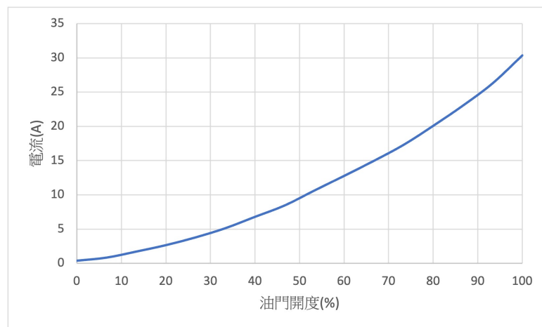
圖 77: 風扇開度對應電流曲線圖
