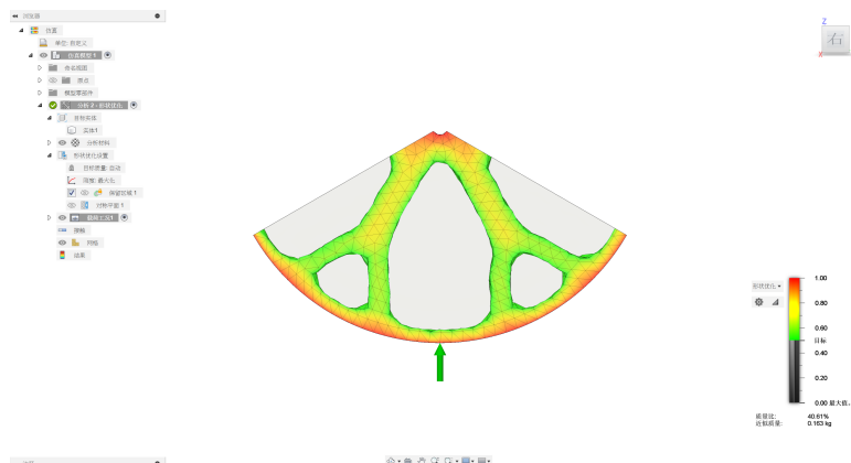
圖 64: 輪椅大輪的形狀優化 1
