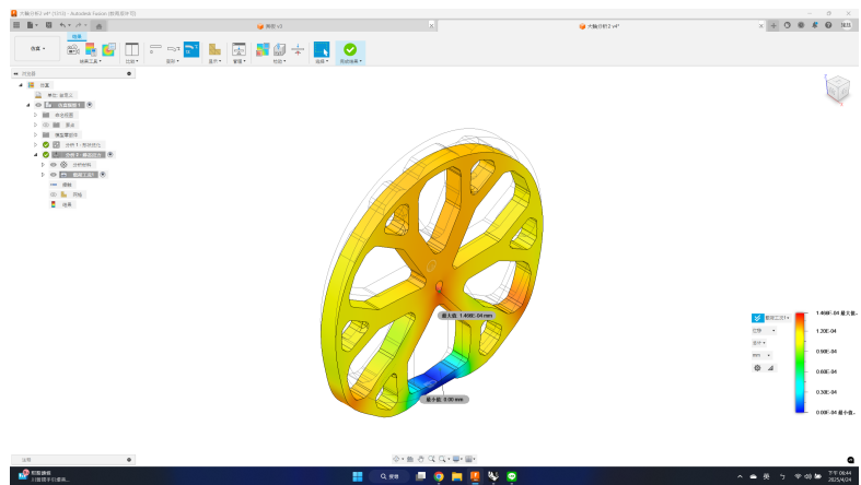
圖 67: 輪椅大輪的位移分析
