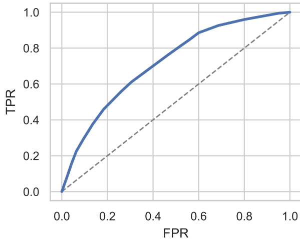
ROC (AUC=0.7168)
