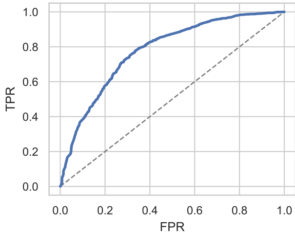
ROC (AUC=0.7779)
