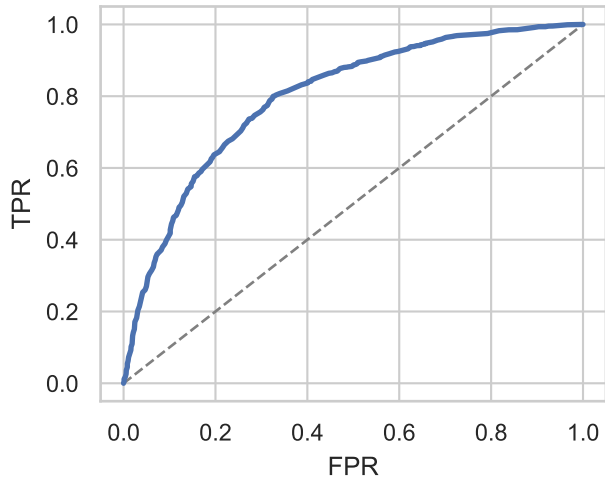
ROC (AUC=0.7980)
