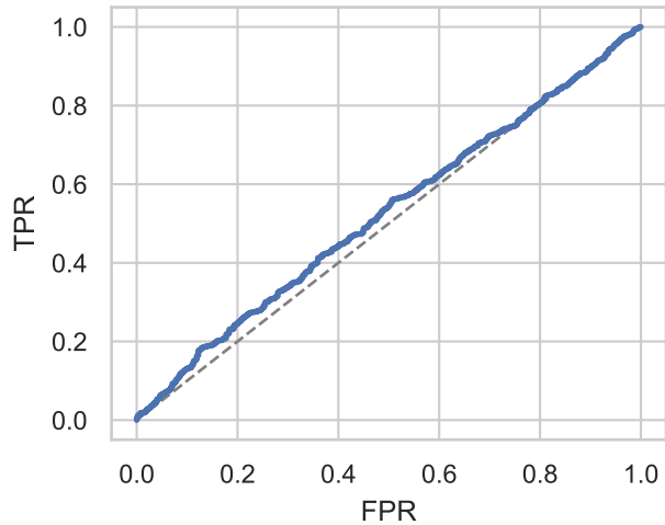
ROC (AUC=0.5246)
