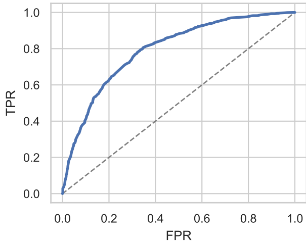
ROC (AUC=0.7936)
