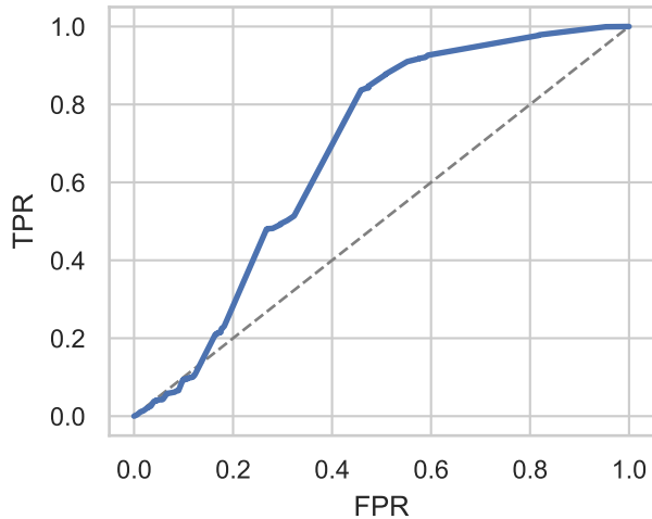
ROC (AUC=0.6797)
