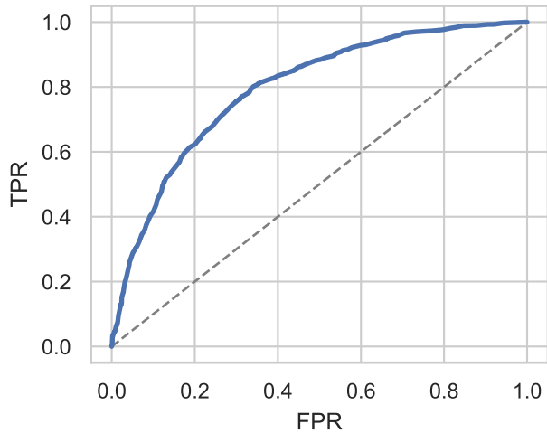
ROC (AUC=0.7951)
