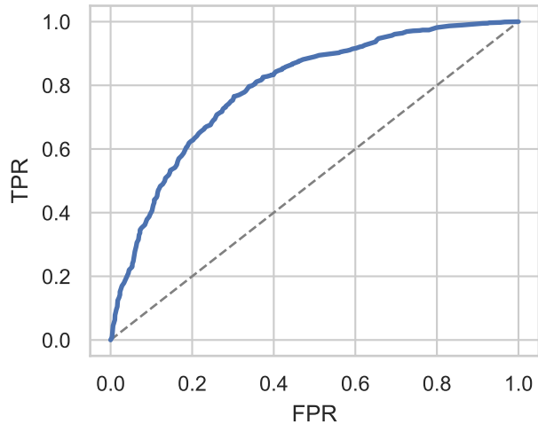
ROC (AUC=0.7922)
