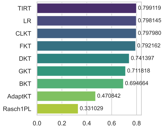
F1 (↑)
