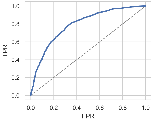
ROC (AUC=0.7935)
