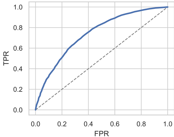
ROC (AUC=0.7414)
