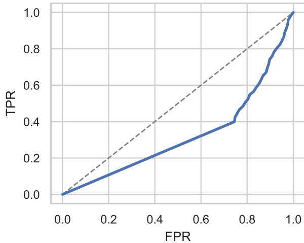
ROC (AUC=0.3224)
