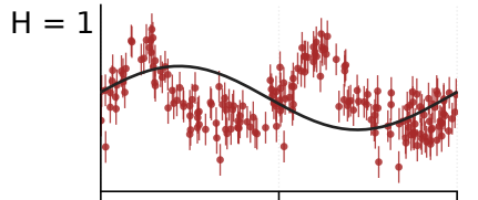
Template fit
