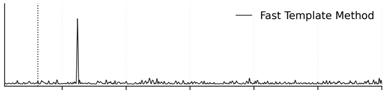
Template periodogram
