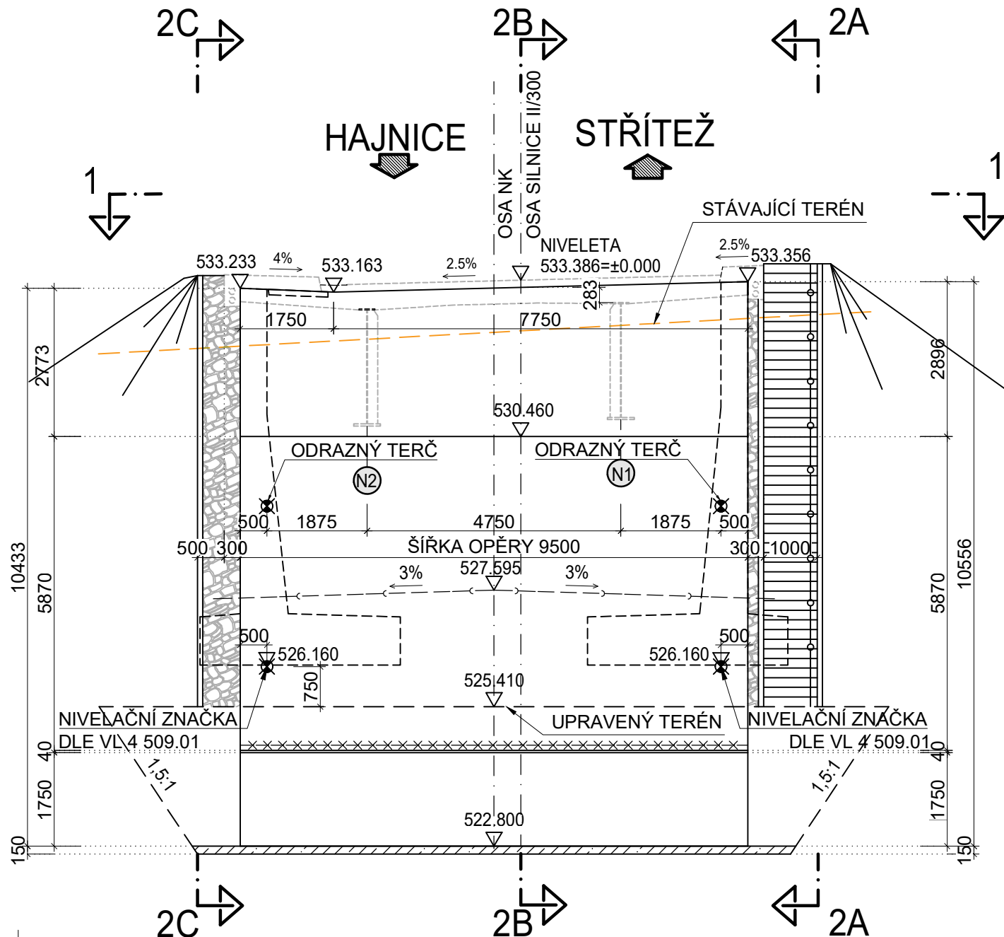
ŘEZ 3A-3A: PŘÍČNÝ - V LÍCI OPĚRY O1 M 1:100
