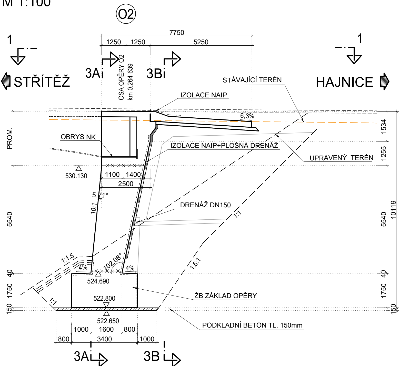
ŘEZ 2C-2C : POHLED NA KŘÍDLO M 1:100
