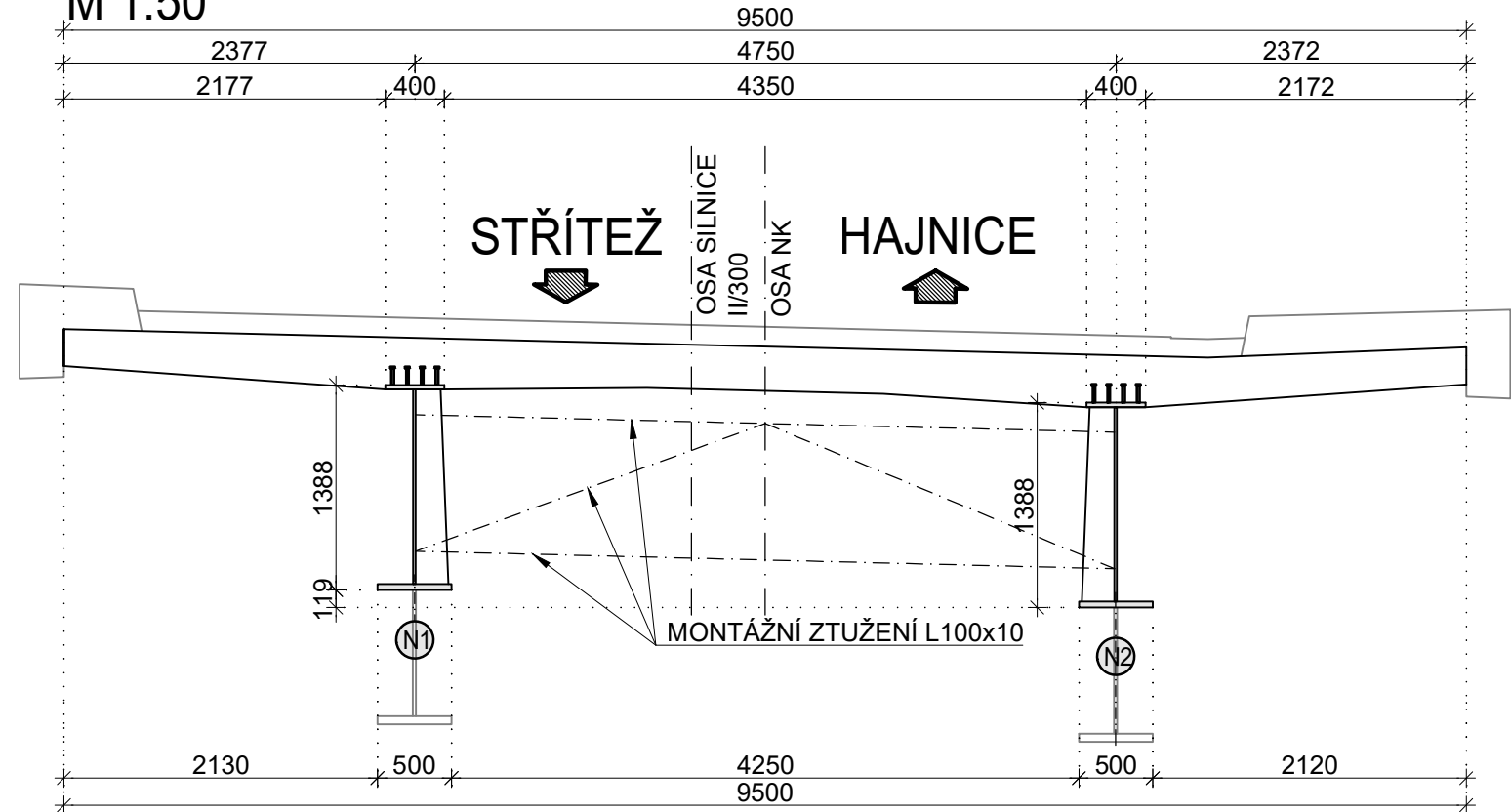
PŘÍČNÝ ŘEZ: ŘEZ 3-3 M 1:50
