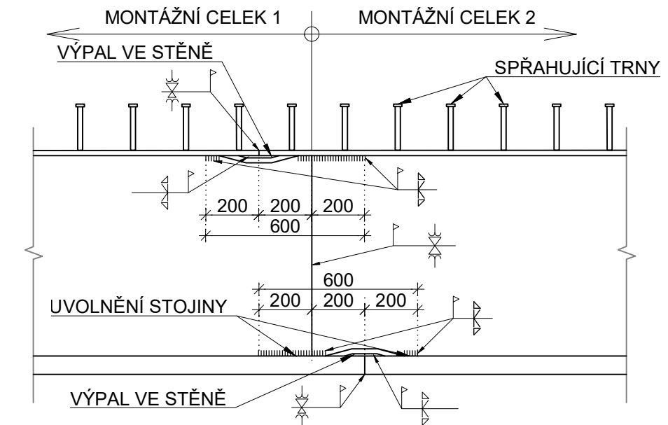
DETAIL A: MONTÁŽNÍ STYK M 1:20
