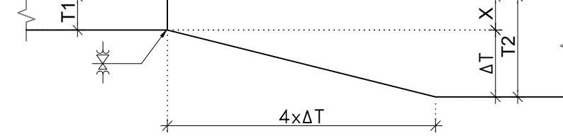
DETAIL B: ZMĚNA TLOUŠTKY PÁSNIC M 1:20
