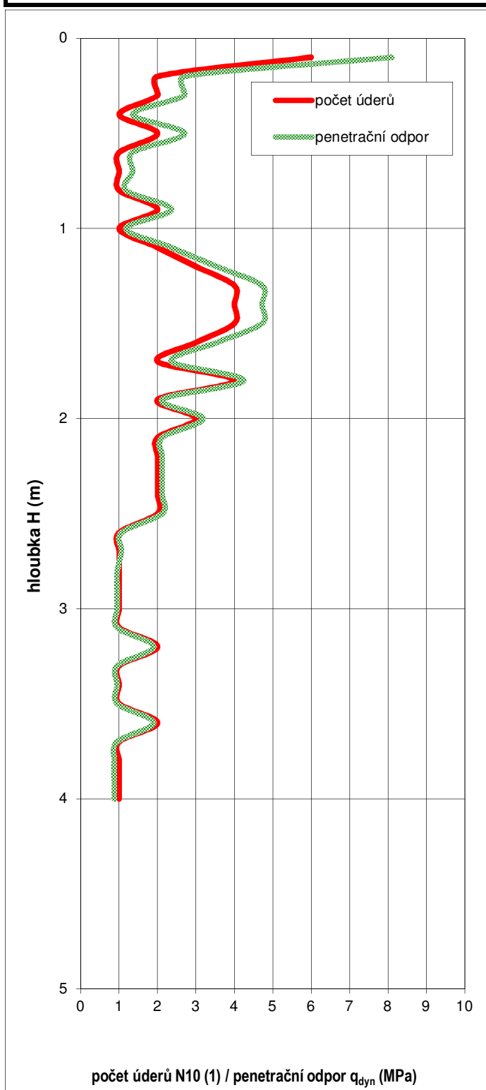
GRAF PRŮBEHU ZKOUSKY
