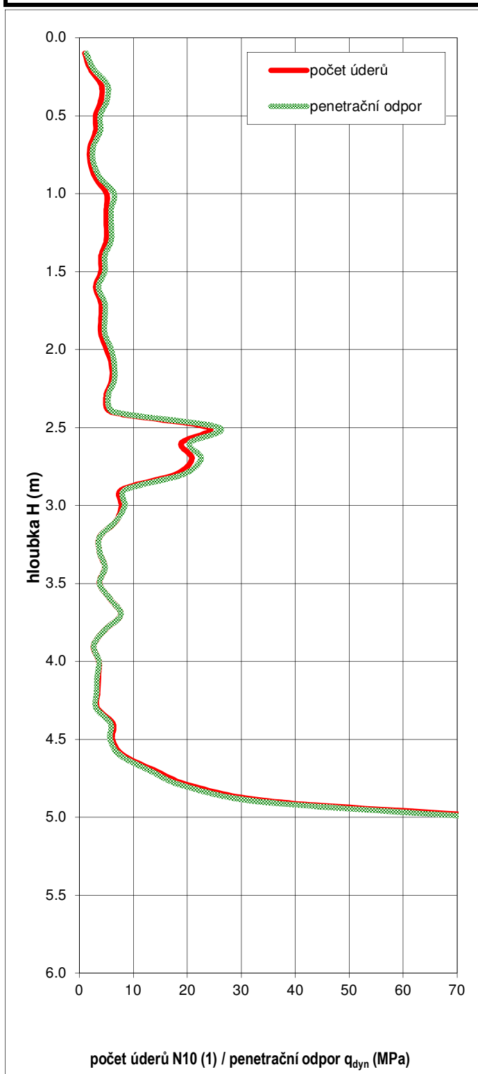
GRAF PRŮBEHU ZKOUŠKY
