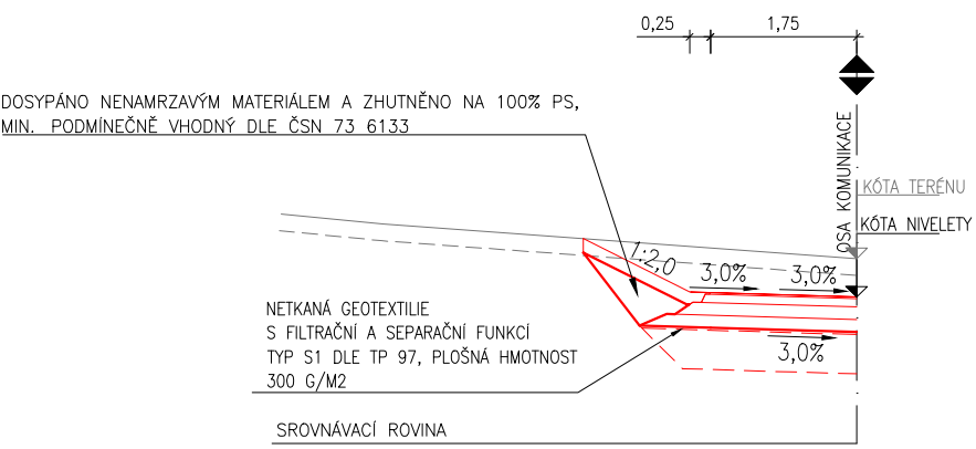
SO 161 P 4,0/30 – V ŽÁŘEZU BEZ PŘÍKOPU
