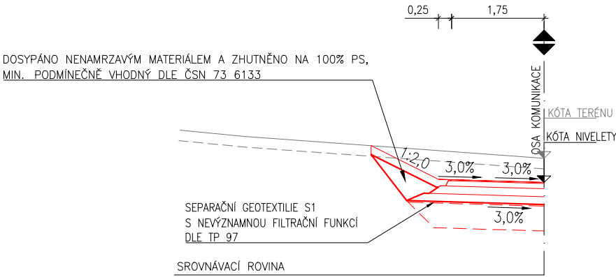
SO 161 P 4,0/30 – V ŽÁŘEZU BEZ PŘÍKOPU
