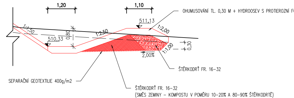
PŘELIVNÝ PŘÍKOP STANDARDNÍ KONSTRUKCE (NA ZBYLÝCH ÚSECÍCH PŘÍKOPU)
