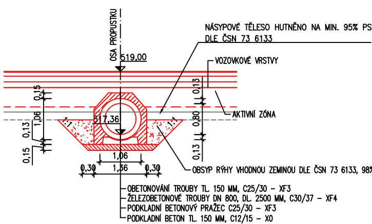
PŘÍČNÝ ŘEZ ULOŽENÍM PROPUSTKU POD KOMUNIKACÍ
