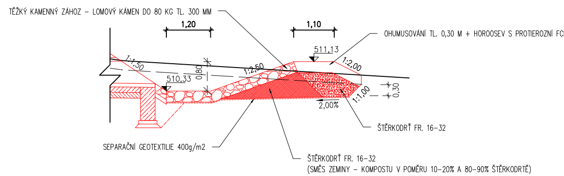
PŘELIVNÝ PŘÍKOP KONSTRUKCE ZA VÝTOKEM (V DÉLCE 2 M OD KONST. NA VÝTOKU)
