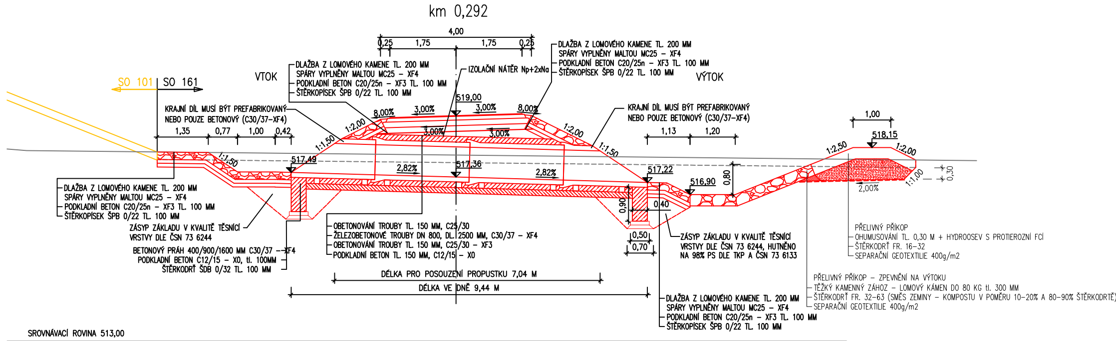
PŘELIVNÝ PŘÍKOP KONSTRUKCE NA VÝTOKU (V DÉLCE 2 M OD OSY PROPUSTKU)
