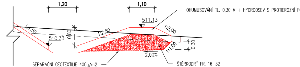
PŘELIVNÝ PŘÍKOP STANDARDNÍ KONSTRUKCE (NA ZBYLÝCH ÚSECÍCH PŘÍKOPU)
