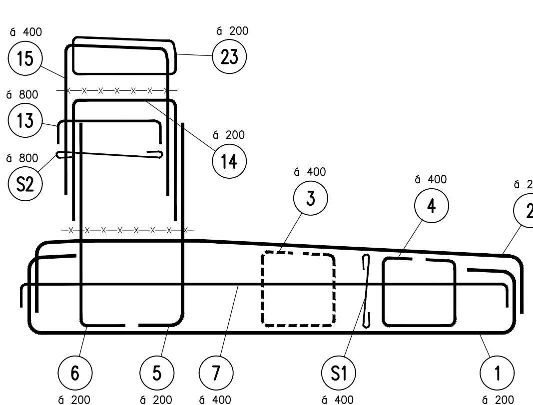
SCHÉMA VÝZTUŽE 1:25
