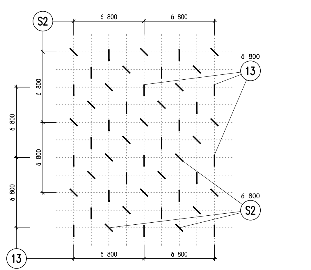
SCHÉMA VÝZTUŽE 1:25
