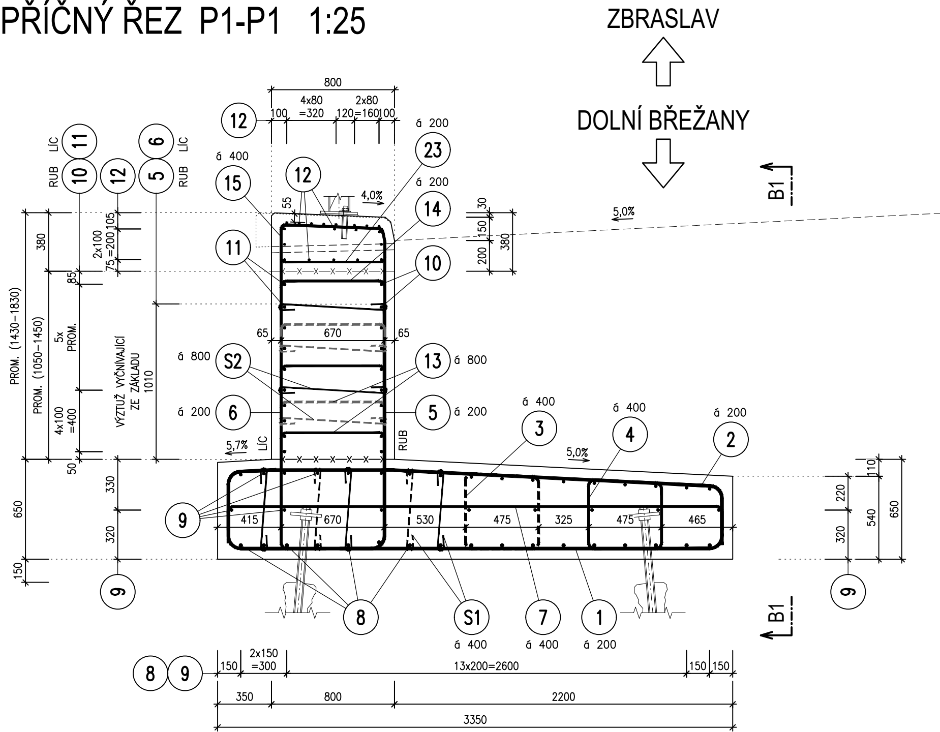
PŘÍČNÝ ŘEZ P1-P1 1:25
