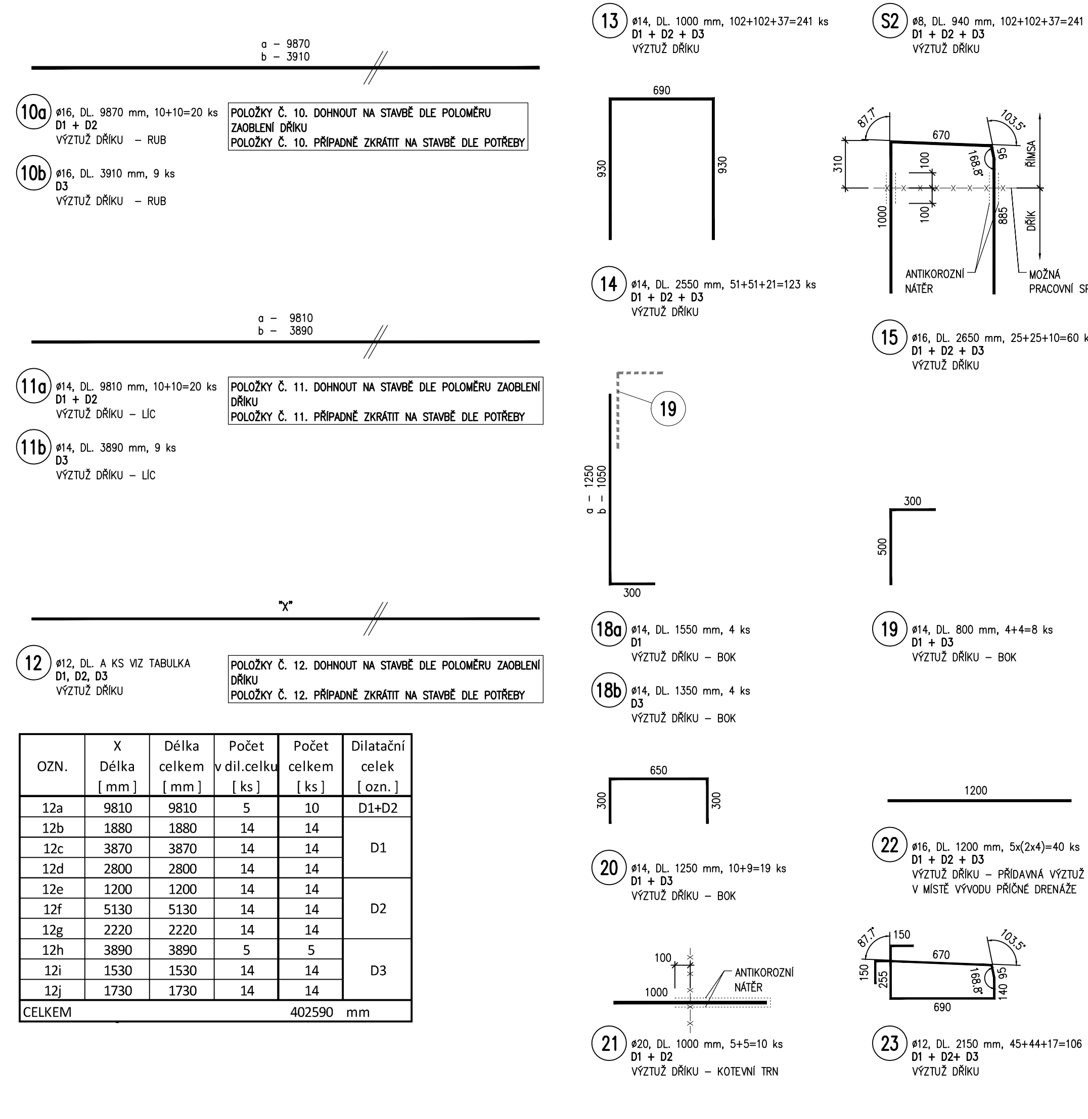
VÝTAH VÝZTUŽE - DŘÍK 1:25
