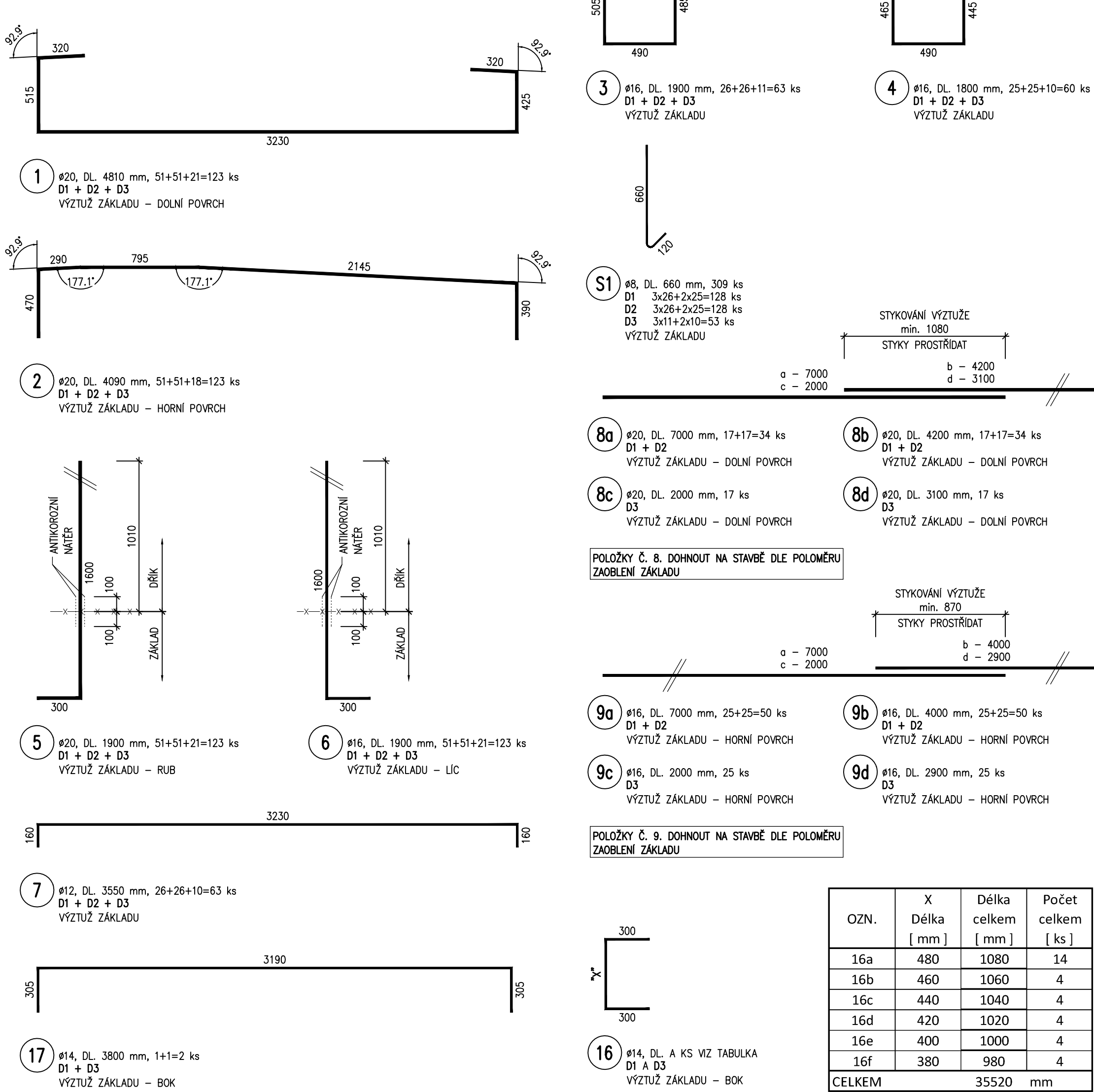
VÝTAH VÝZTUŽE - ZÁKLAD 1:25
