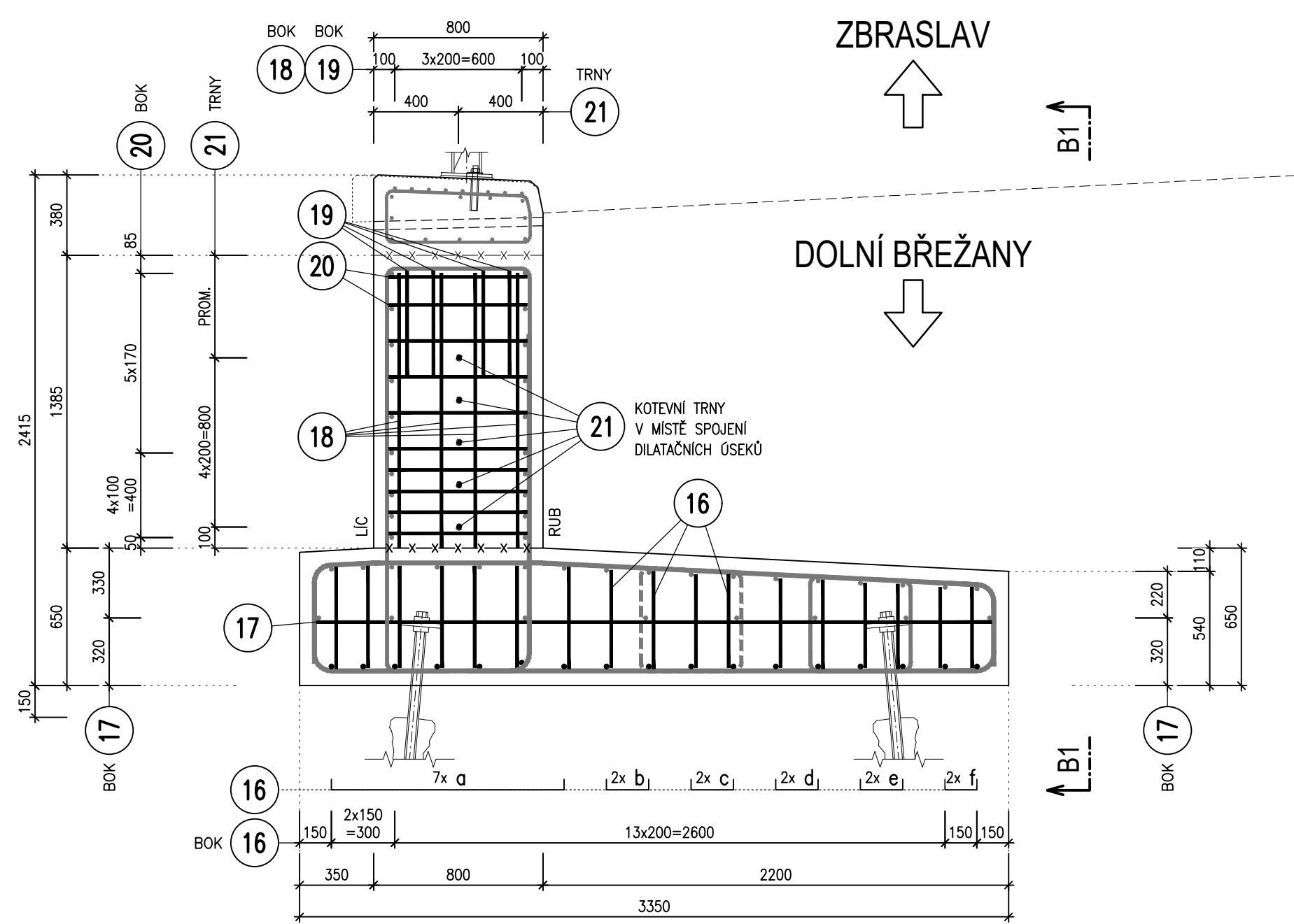
POHLED P2-P2 1:50
