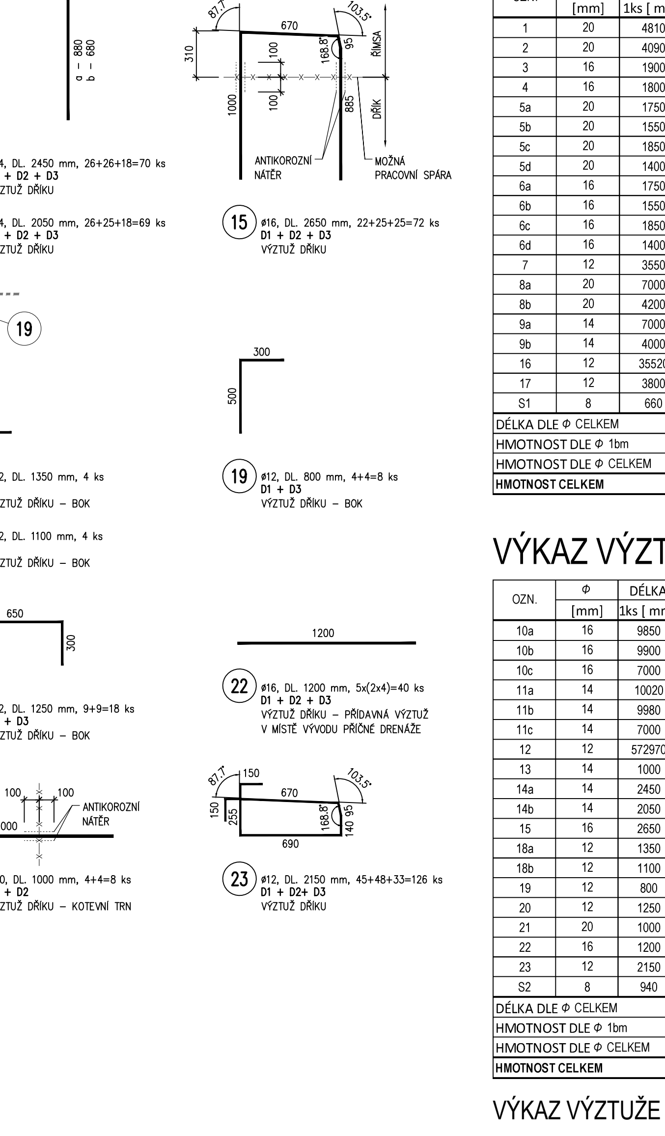
VÝTAH VÝZTUŽE - DŘÍK 1:25 VÝZTUŽ KÓTOVÁNA NA VNĚJŠÍ OBRYŠ
