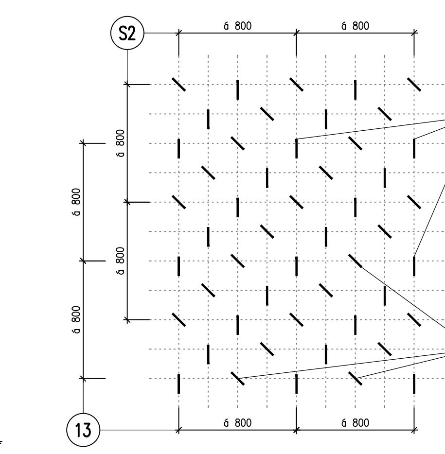
SCHÉMA VÝZTUŽE 1:25 POLOŽKA Č. 13, S2
