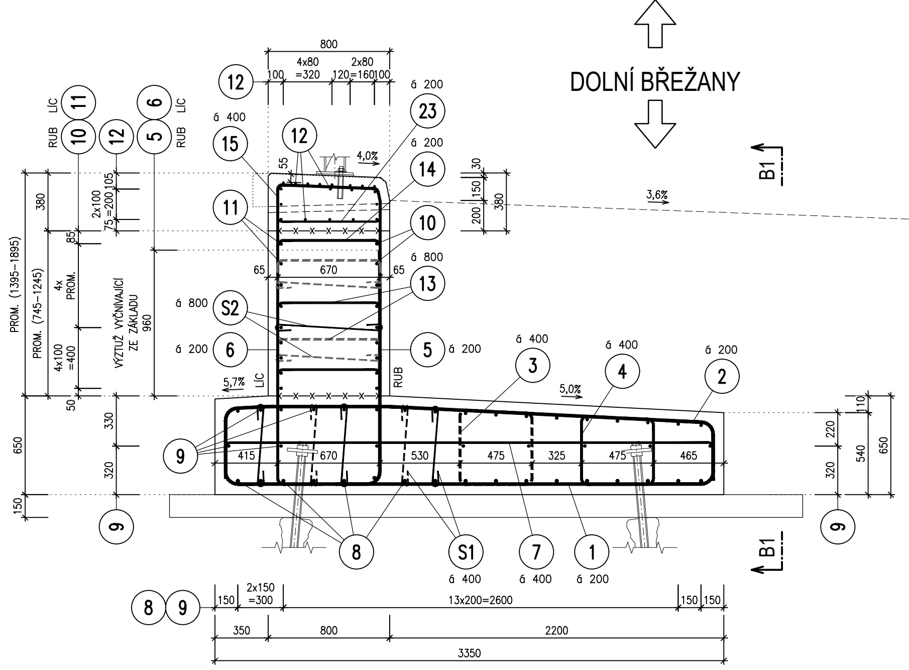
PŘÍČNÝ ŘEZ P1-P1 1:25
