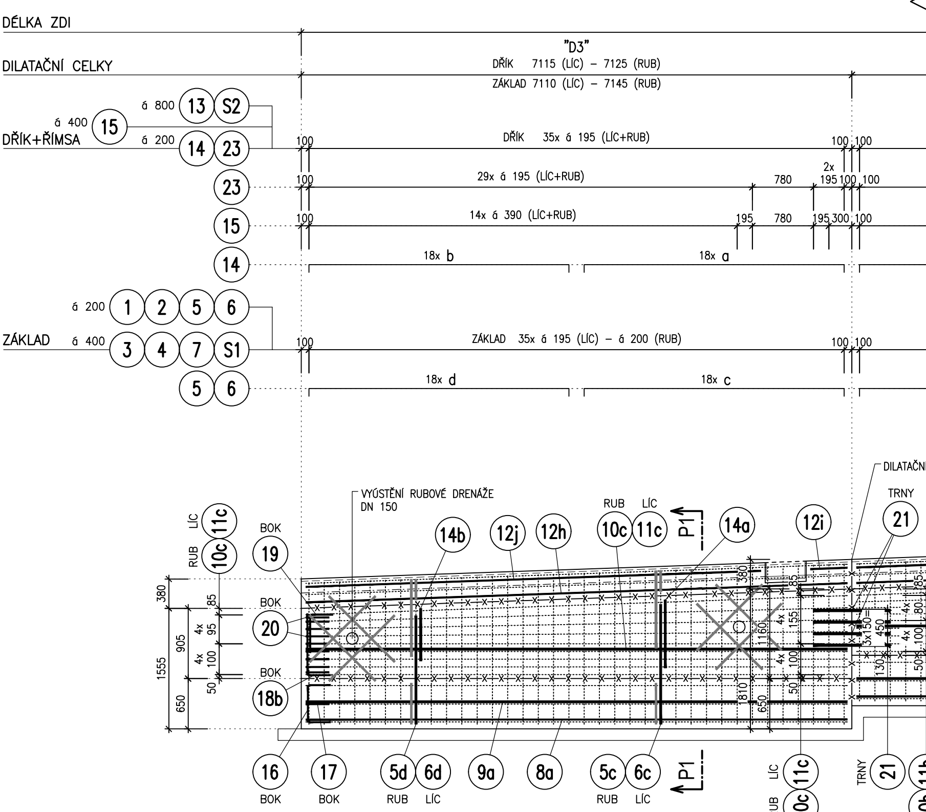
POHLED V LÍCI B1-B1 1:50
