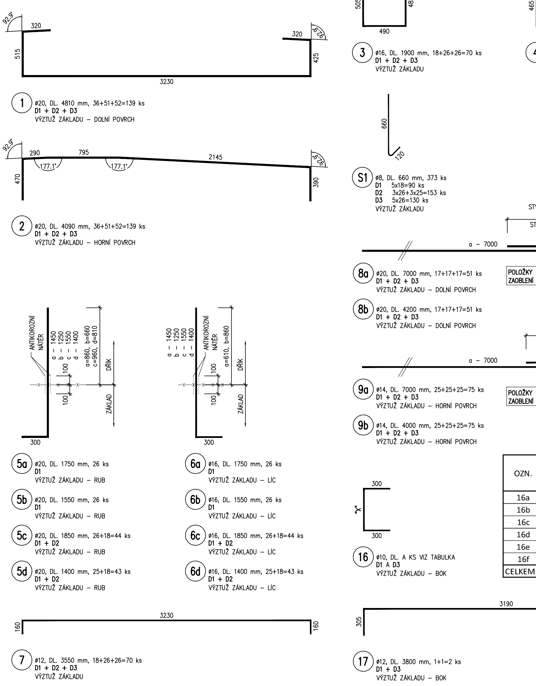
VÝTAH VÝZTUŽE - ZÁKLAD 1:25 VÝZTUŽ KÓTOVÁNA NA VNĚJŠÍ OBRYŠ
