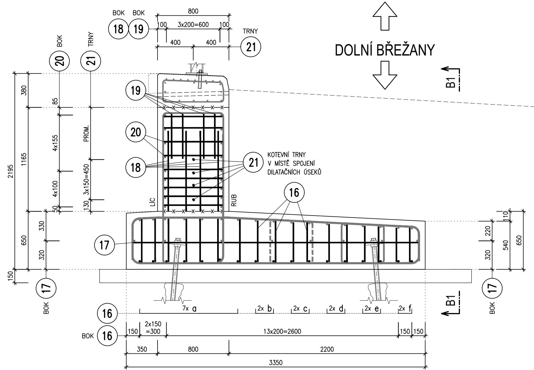
POHLED P2-P2 1:50
