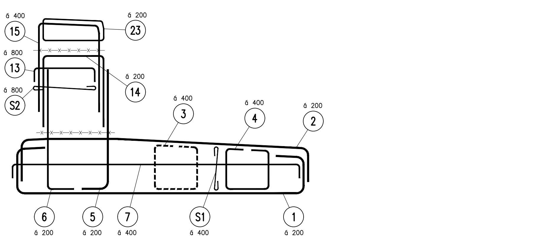
SCHÉMA VÝZTUŽE 1:25
