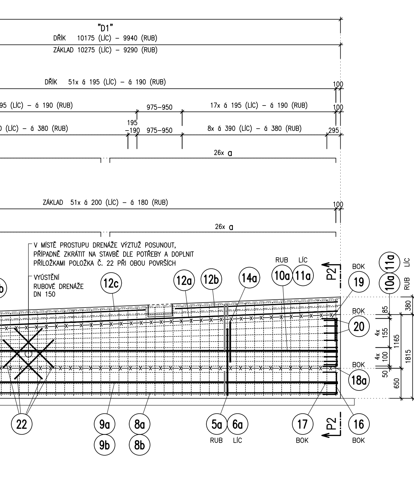
POHLED V LÍCI B1-B1 1:50
