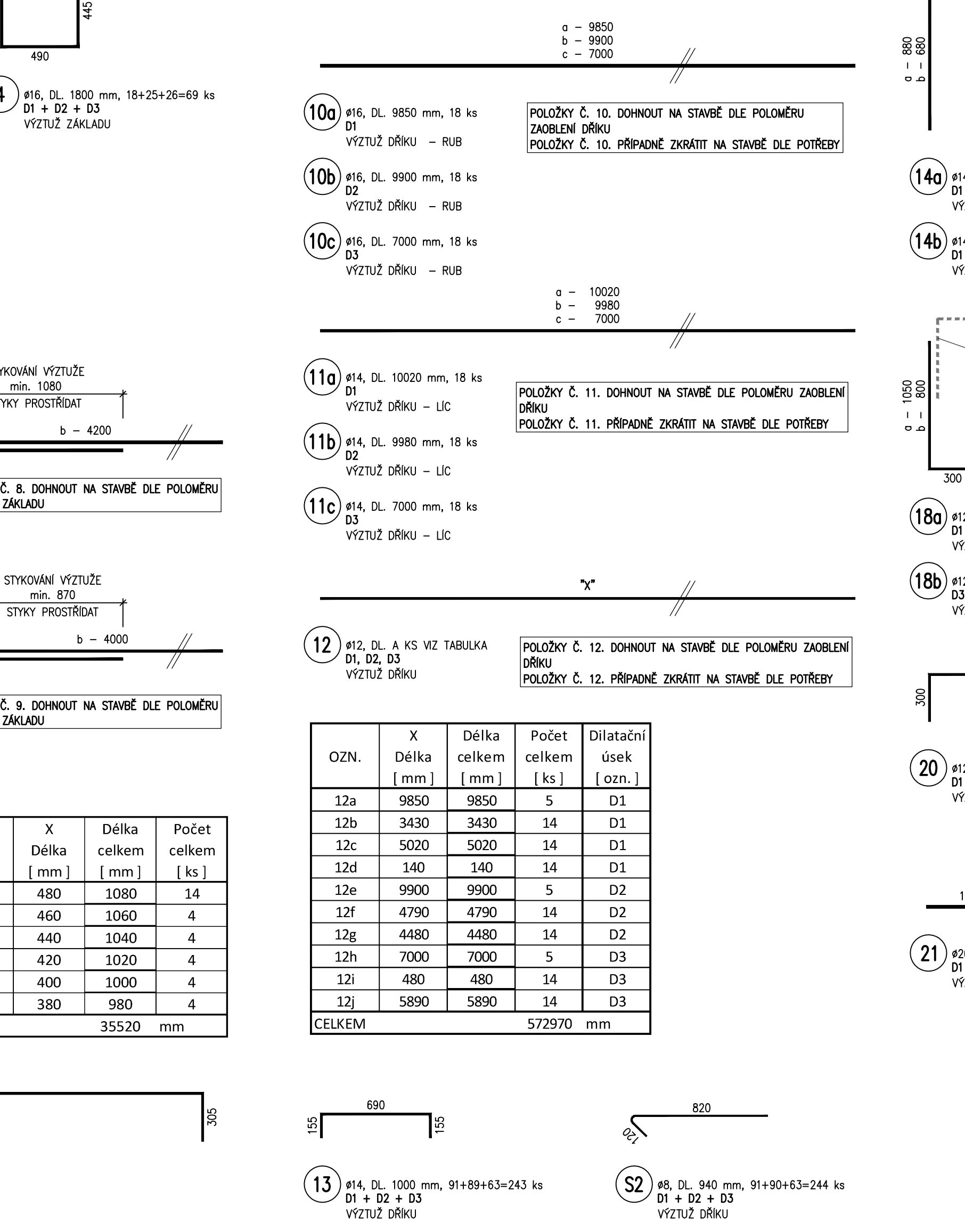
VÝTAH VÝZTUŽE - DŘÍK 1:25 VÝZTUŽ KÓTOVÁNA NA VNĚJŠÍ OBRYŠ
