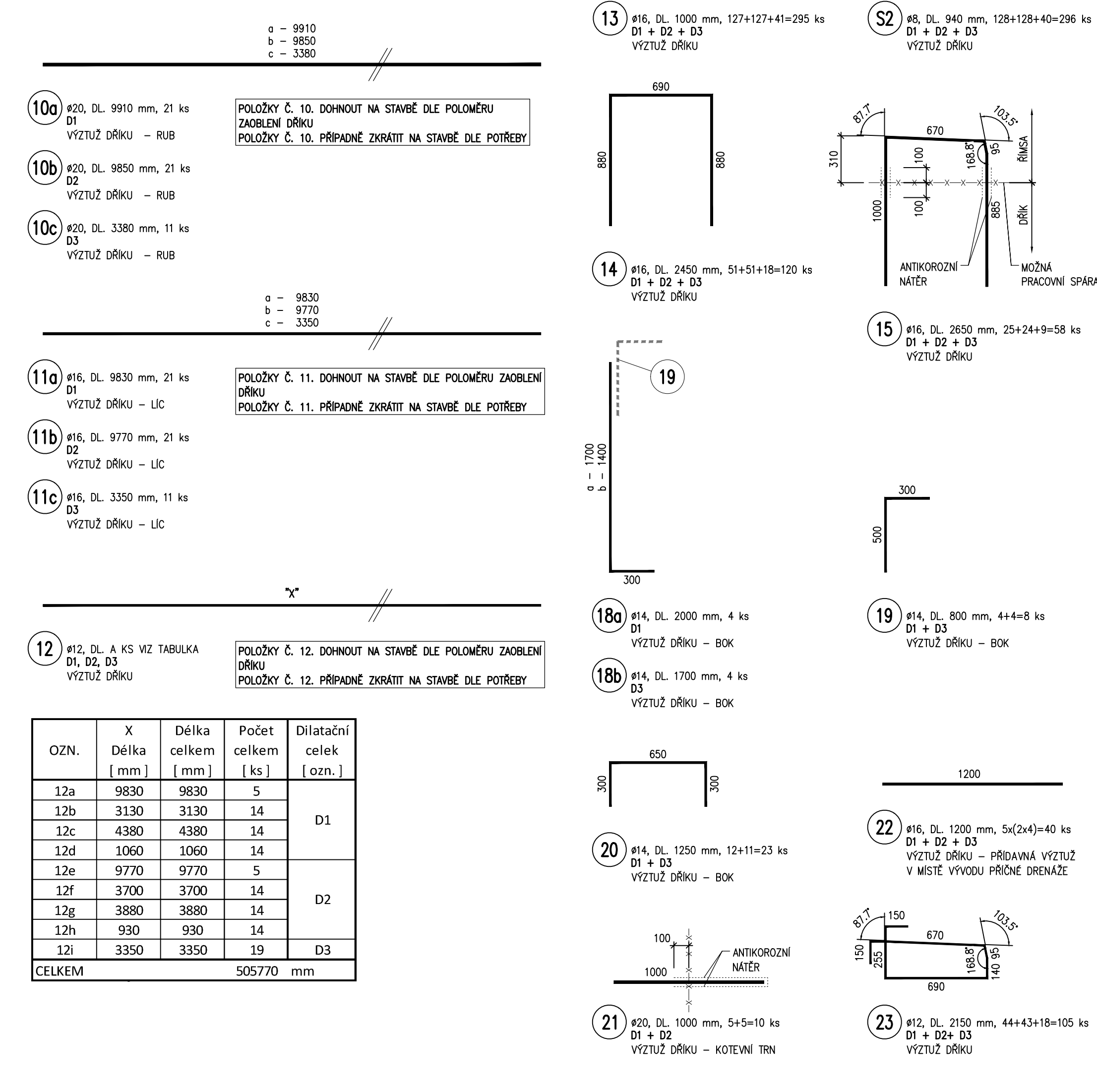
VÝTAH VÝZTUŽE - DŘÍK 1:25 VÝZTUŽ KÓTOVÁNA NA VNĚJŠÍ OBRYŠ
