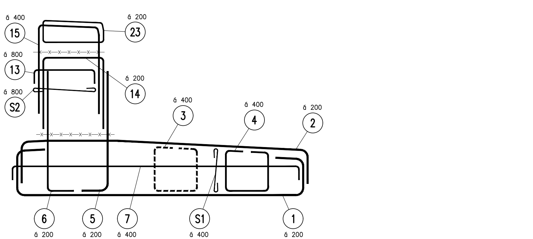
SCHÉMA VÝZTUŽE 1:25
