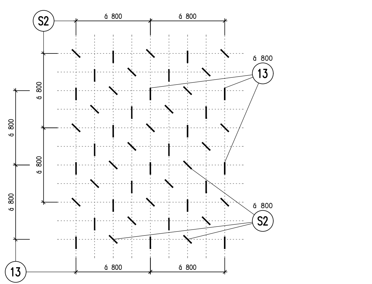
SCHÉMA VÝZTUŽE 1:25 POLOŽKA Č. 13, S2
