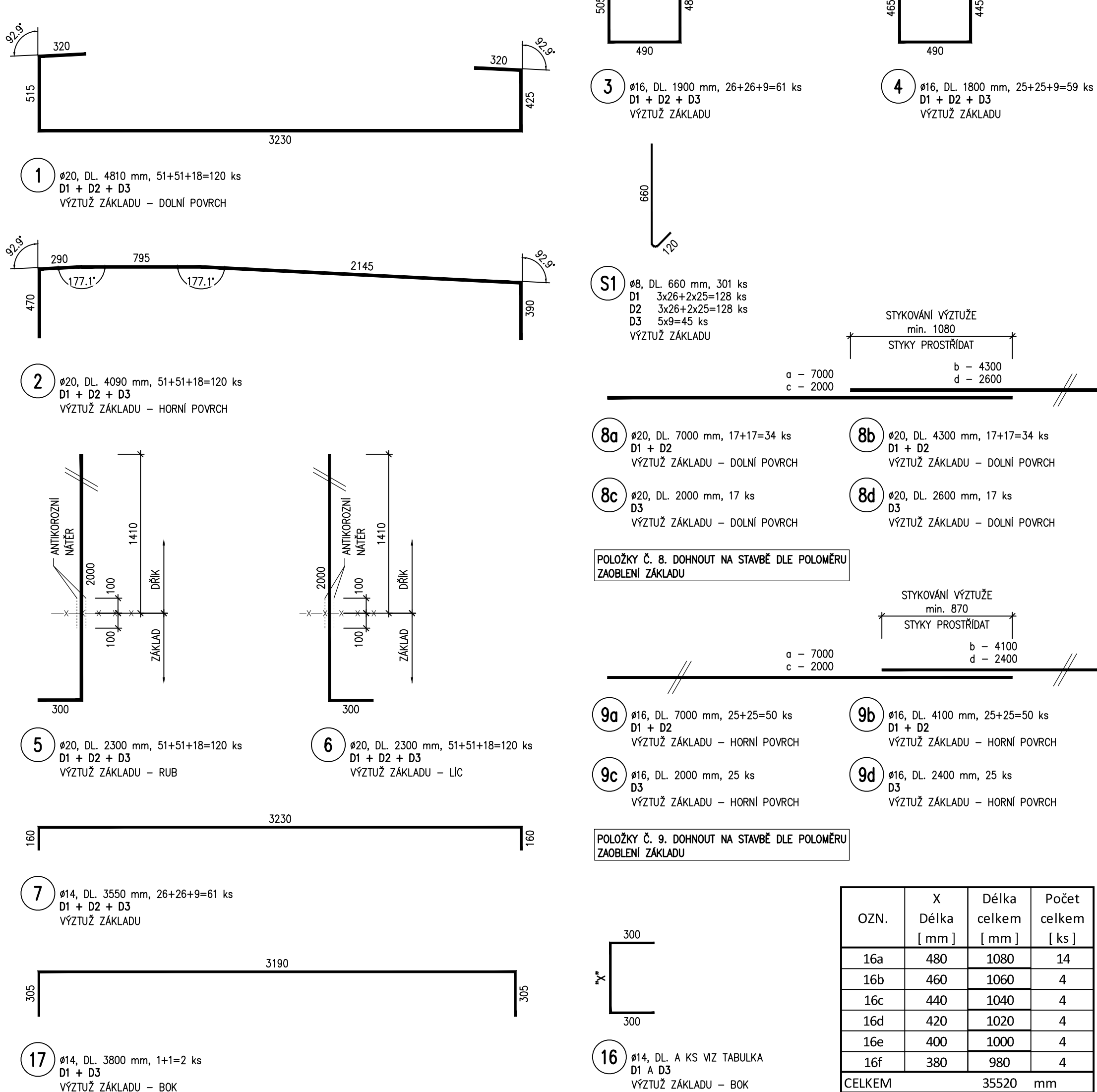
VÝTAH VÝZTUŽE - ZÁKLAD 1:25 VÝZTUŽ KÓTOVÁNA NA VNĚJŠÍ OBRYŠ
