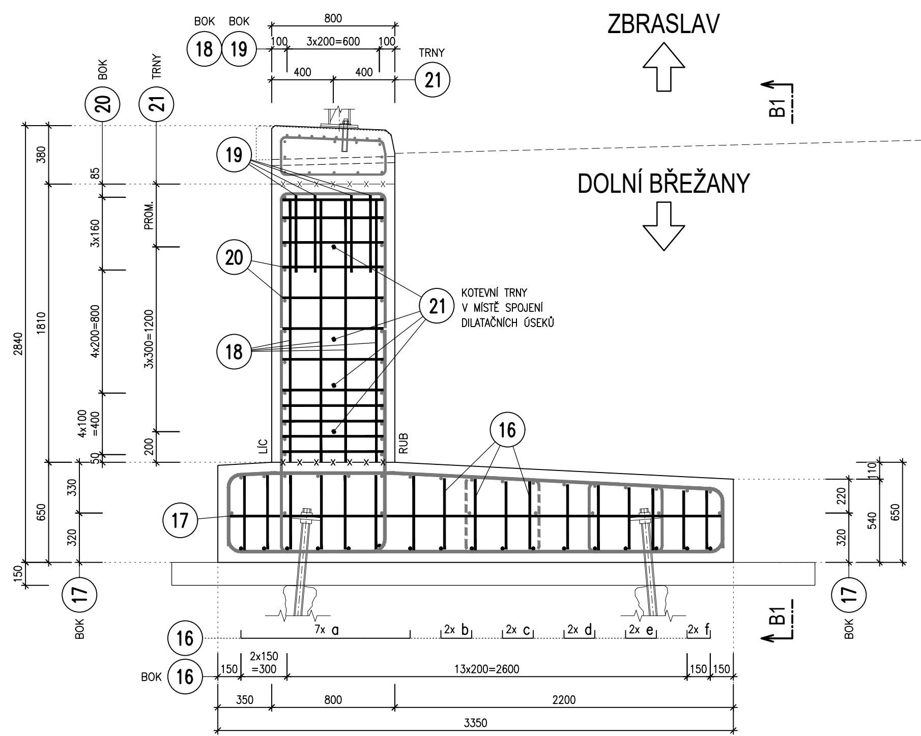
POHLED P2-P2 1:50
