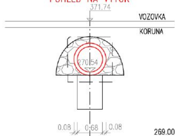
POHLED NA VÝTOK
