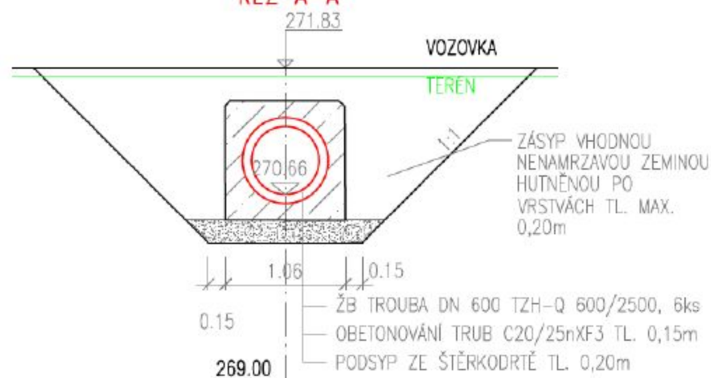
ŘEZ A-A'
