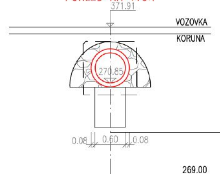
POHLED NA VTOK
