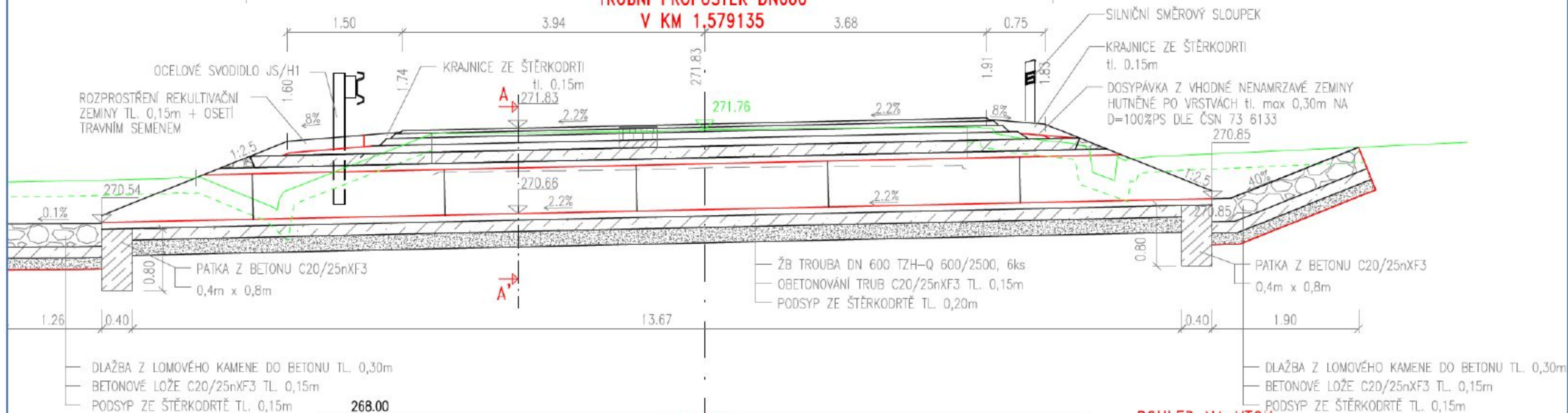
ŘEZ A-A'
