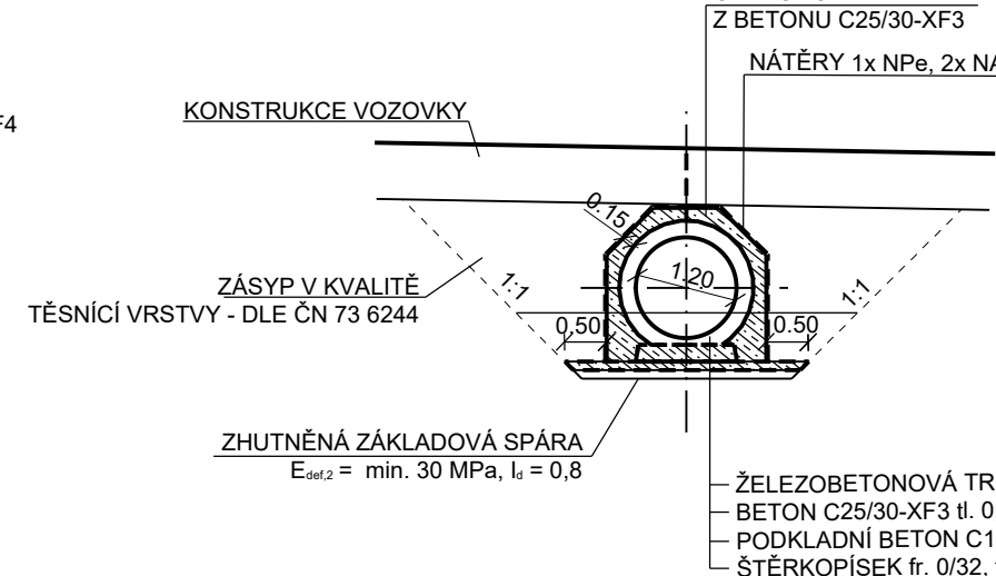
PŘÍČNÝ ŘEZ C-C
