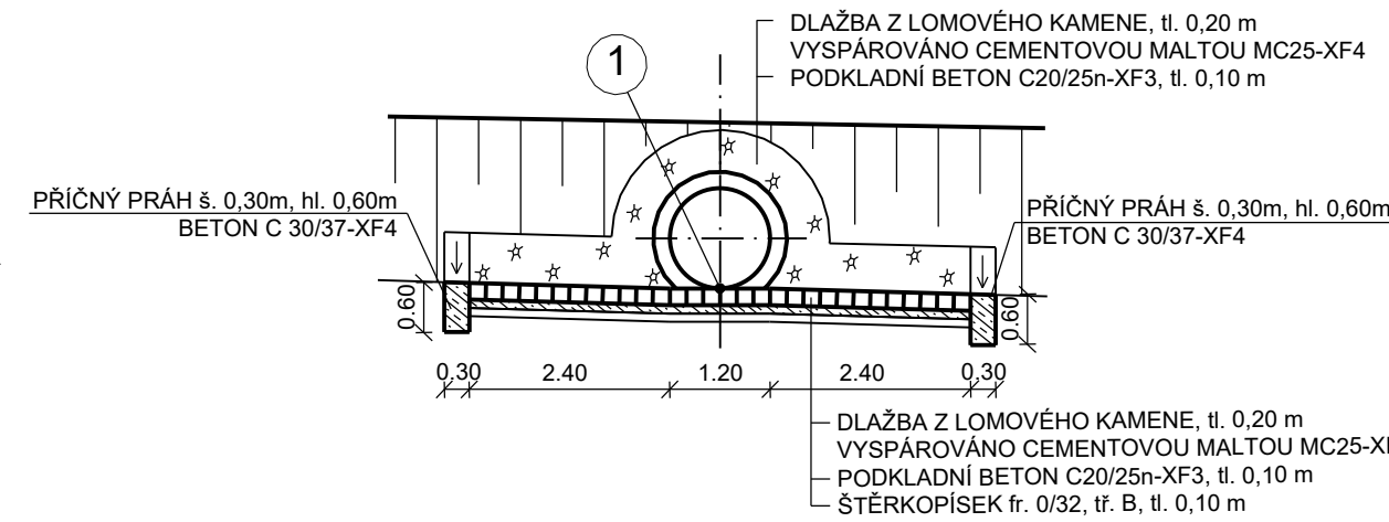
POHLED NA VТОK ŘEZ B-B
