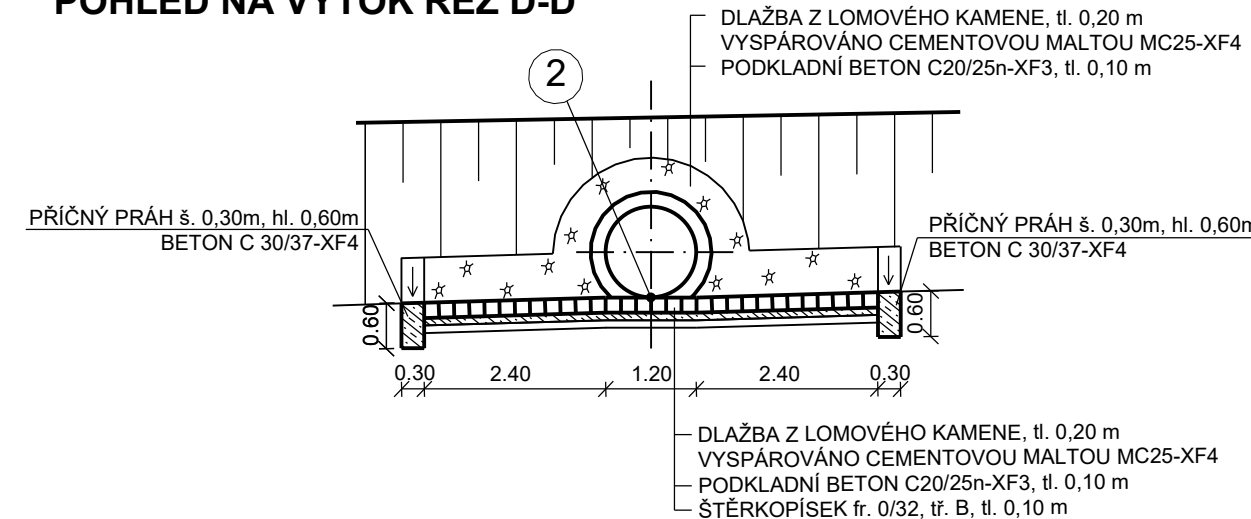
POHLED NA VÝTOK ŘEZ D-D
