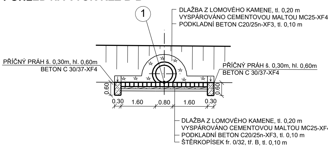
POHLED NA VTOK ŘEZ B-B'
