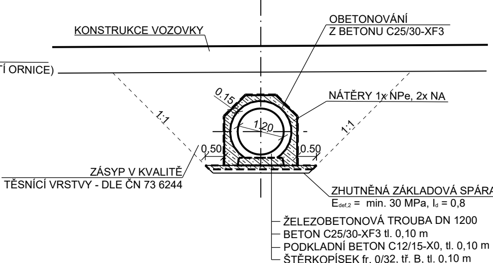
PŘÍČNÝ ŘEZ C-C'
