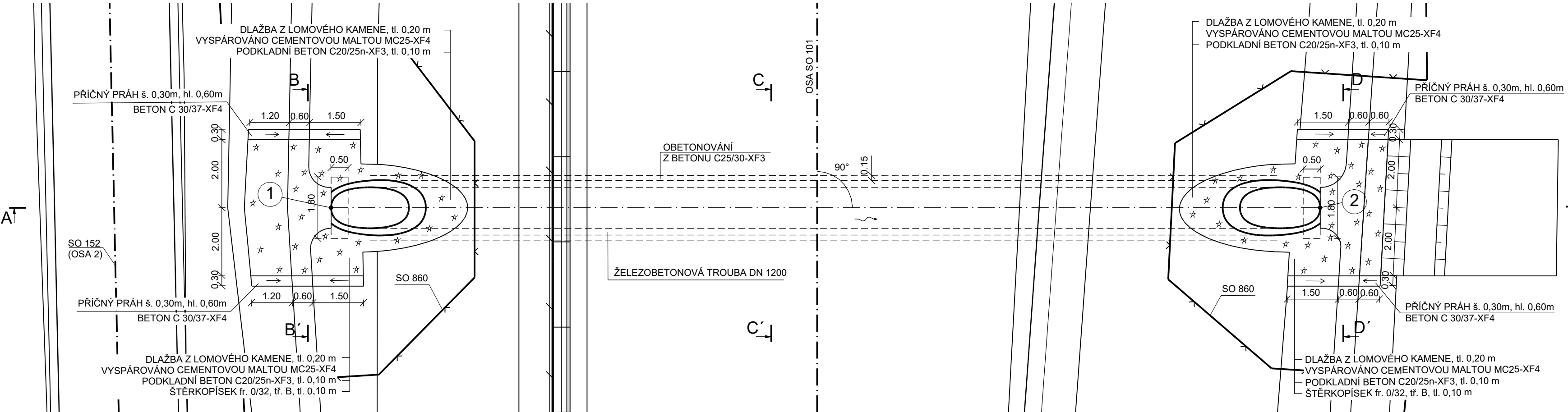
PŮDORYS
