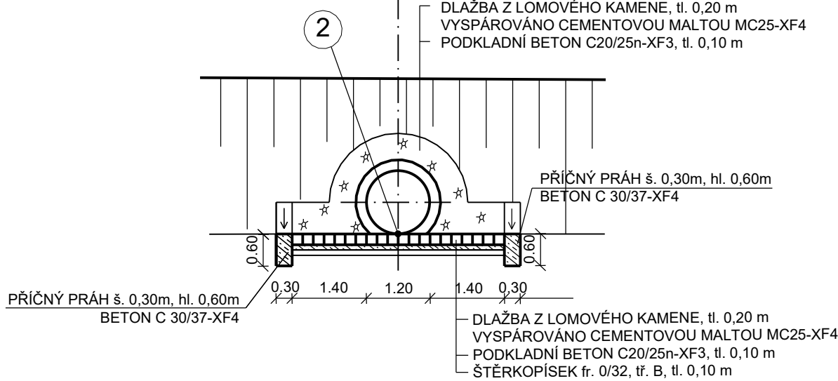
POHLED NA VÝTOK ŘEZ D-D'
