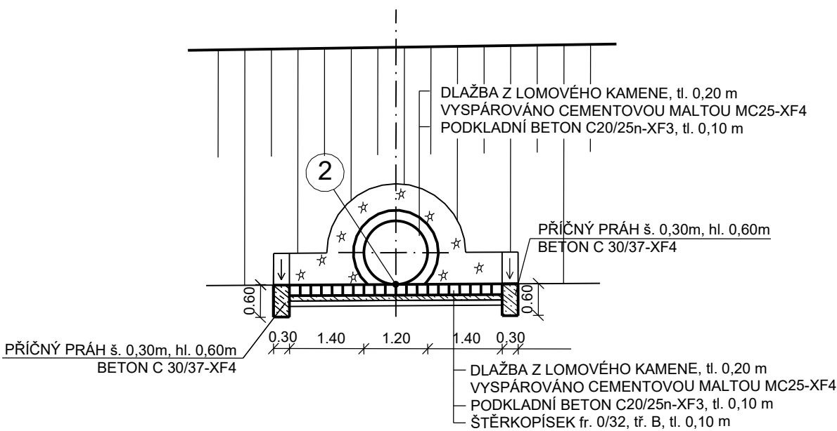
PŘÍČNÝ ŘEZ C-C'
