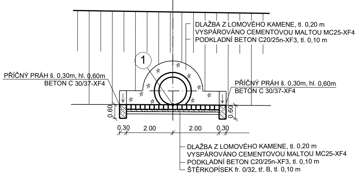
POHLED NA VÝTOK ŘEZ D-D'
