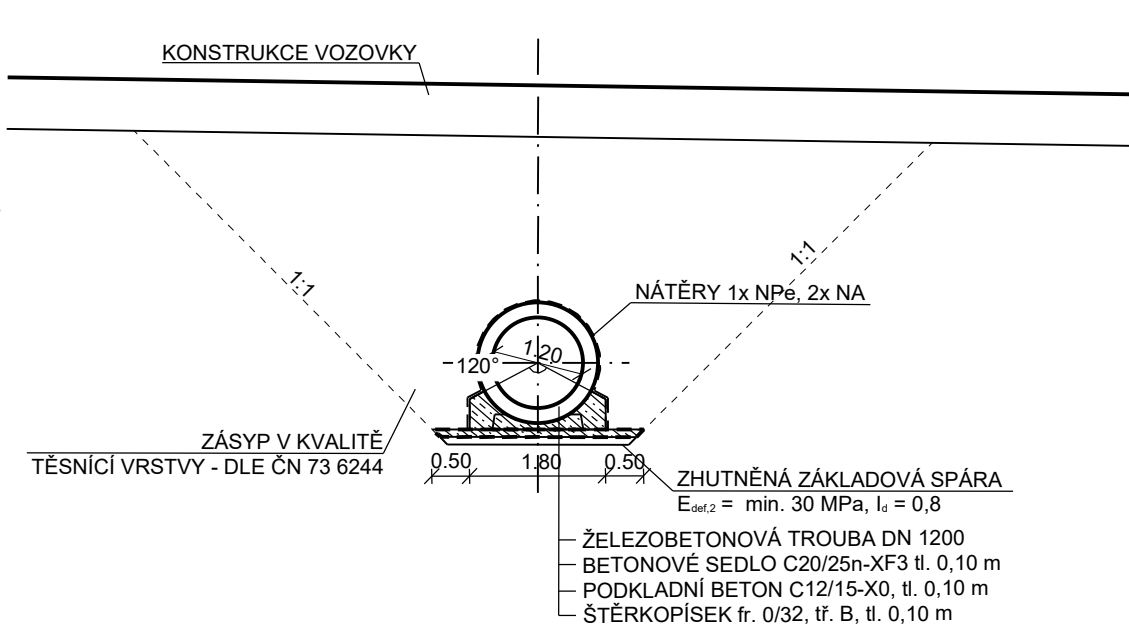
PŘÍČNÝ ŘEZ C-C'
