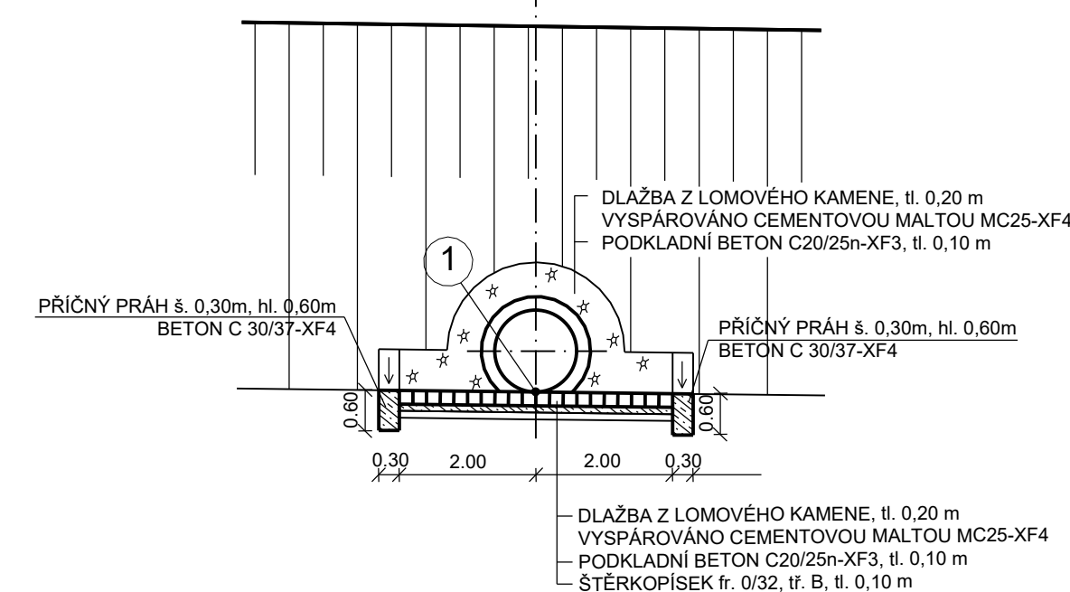
POHLED NA VÝTOK ŘEZ D-D'
