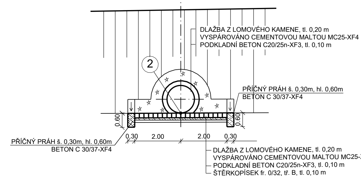
PRÍČNÝ ŘEZ C-C'
