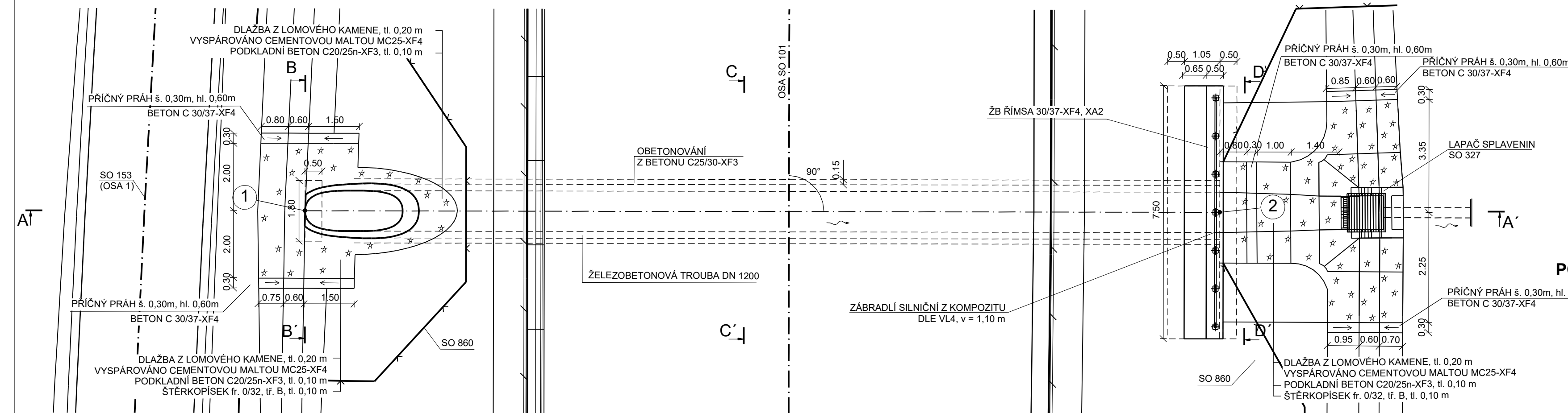
PŮDORYS
