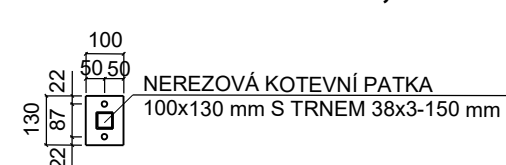
DETAIL KOTEVNÍ PATKY, M 1:10
