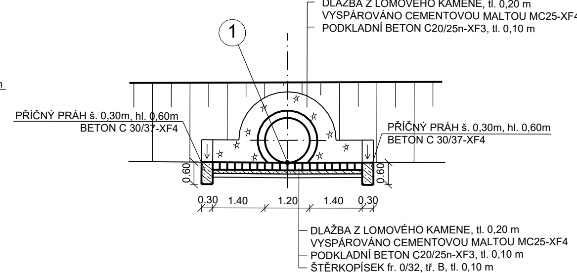
POHLED NA VTOK ŘEZ B-B
