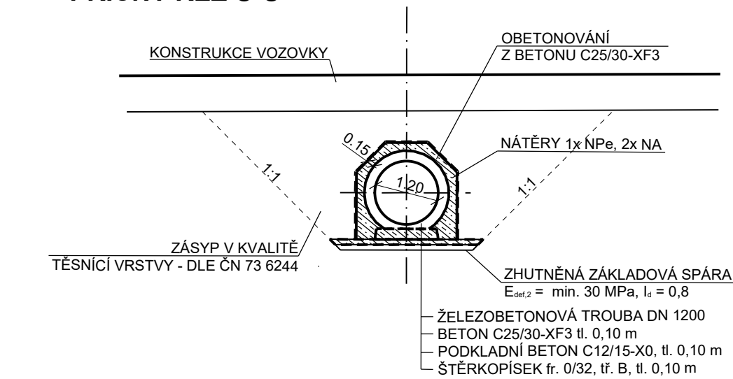
PŘÍČNÝ ŘEZ C-C'
