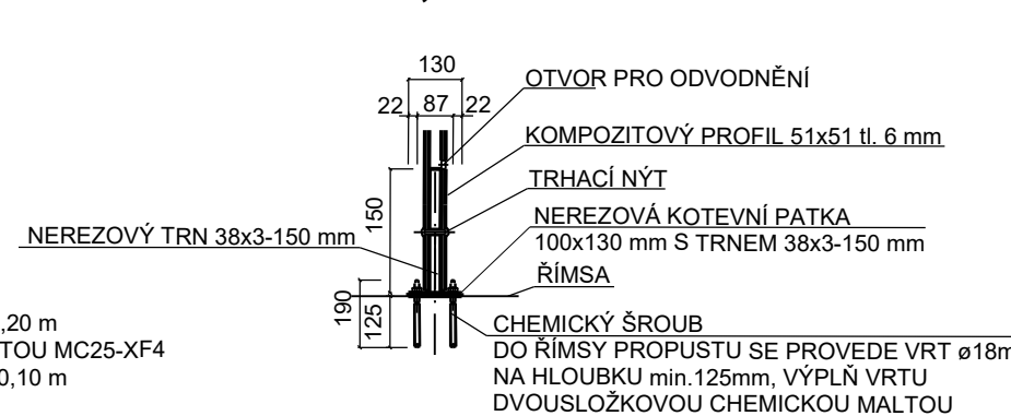
DETAIL UKOTEVNÍ, M 1:10
