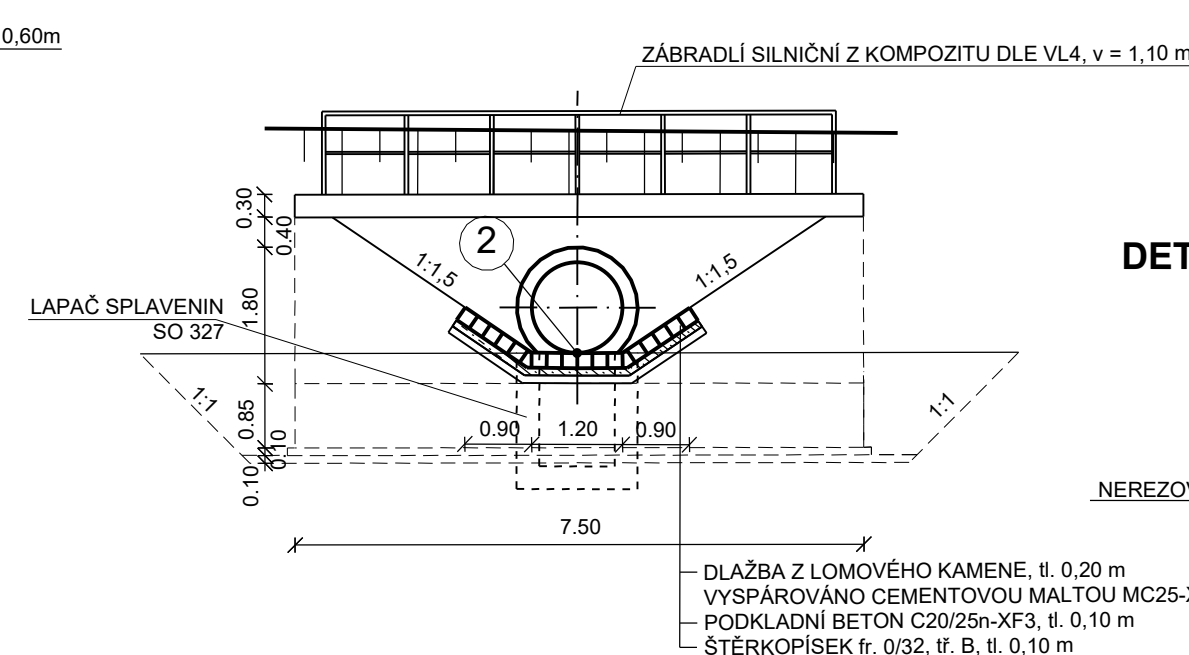
PŘÍČNÝ ŘEZ C-C'
