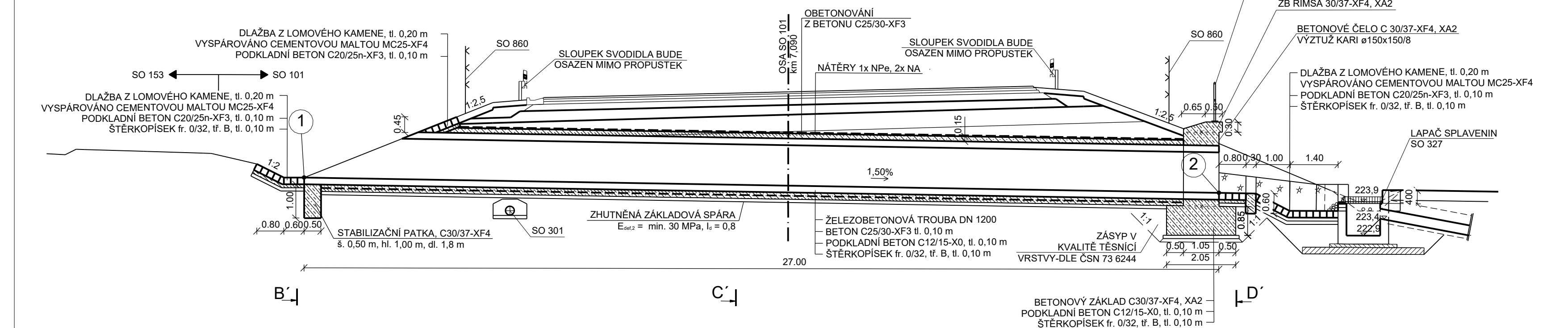
PODÉLNÝ ŘEZ A-A
