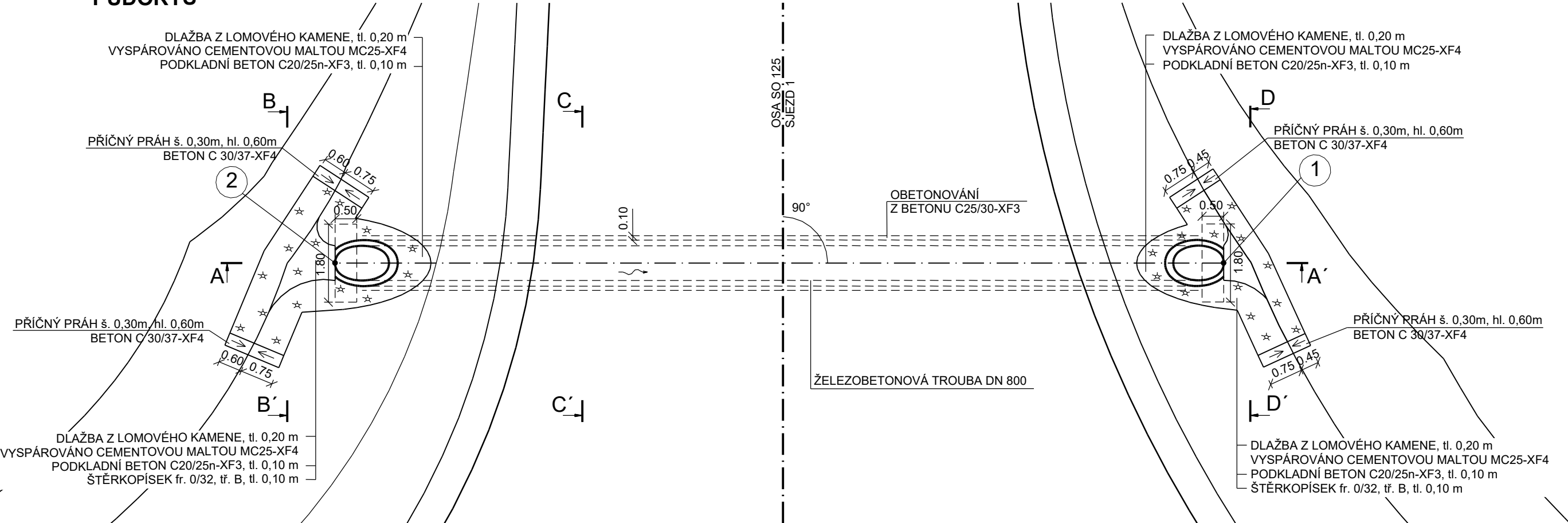
PŮDORYS
