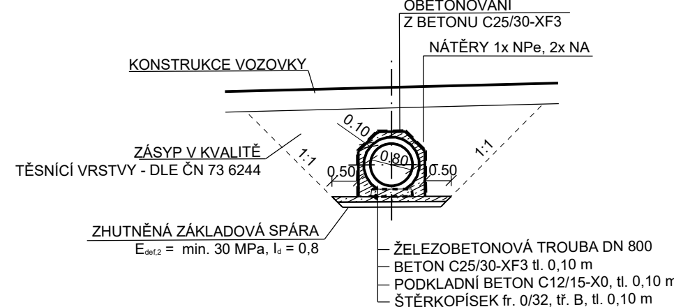
PŘÍČNÝ ŘEZ C-C'
