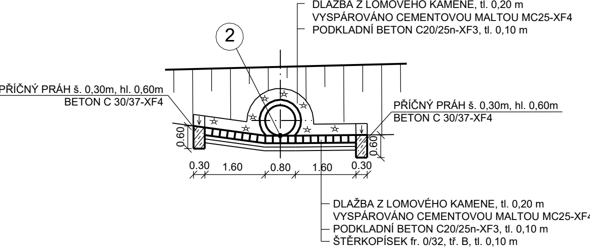
POHLED NA VÝTOK ŘEZ B-B'
