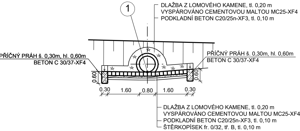
POHLED NA VTOK ŘEZ D-D'
