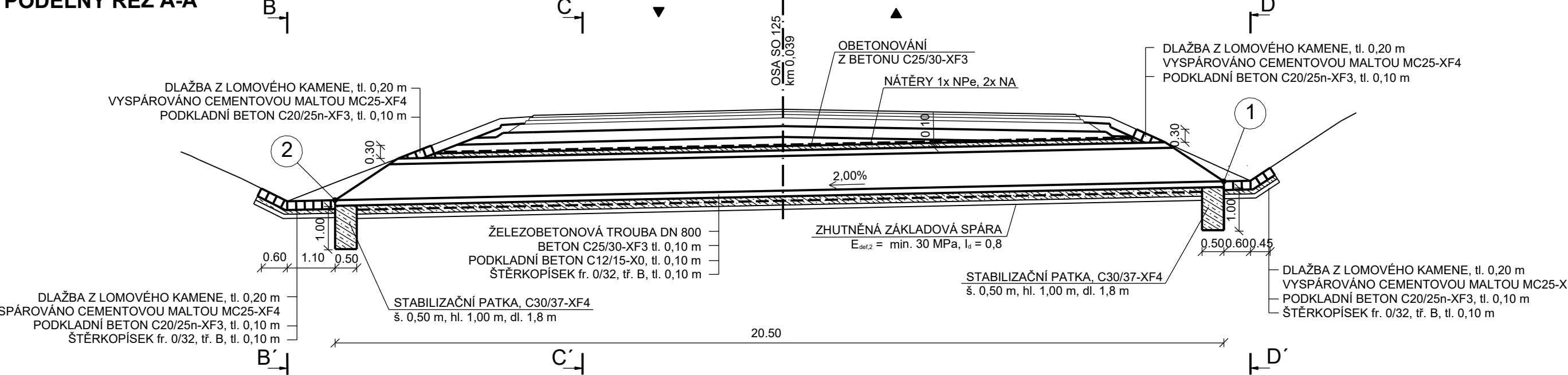
PODÉLNÝ ŘEZ A-A'
