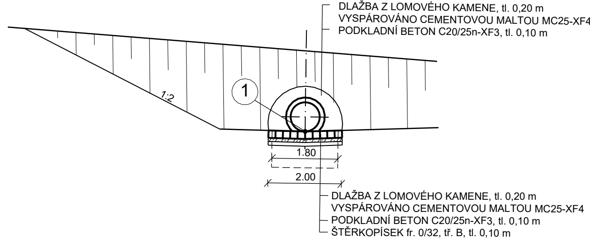
POHLED NA VTOK ŘEZ B-B'
