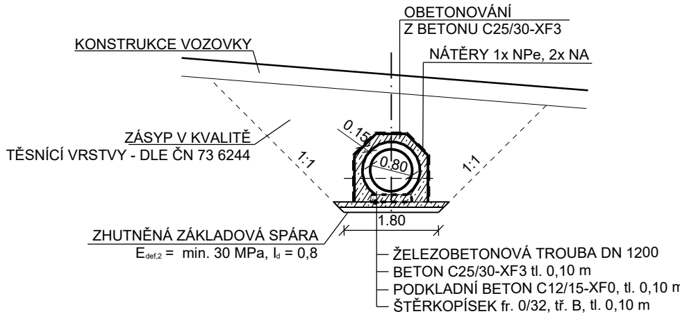
PŘÍČNÝ ŘEZ C-C'
