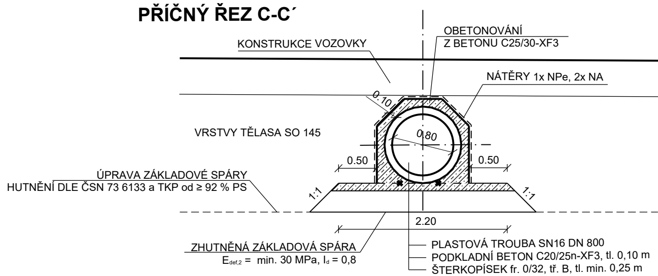
PŘÍČNÝ ŘEZ C-C'
