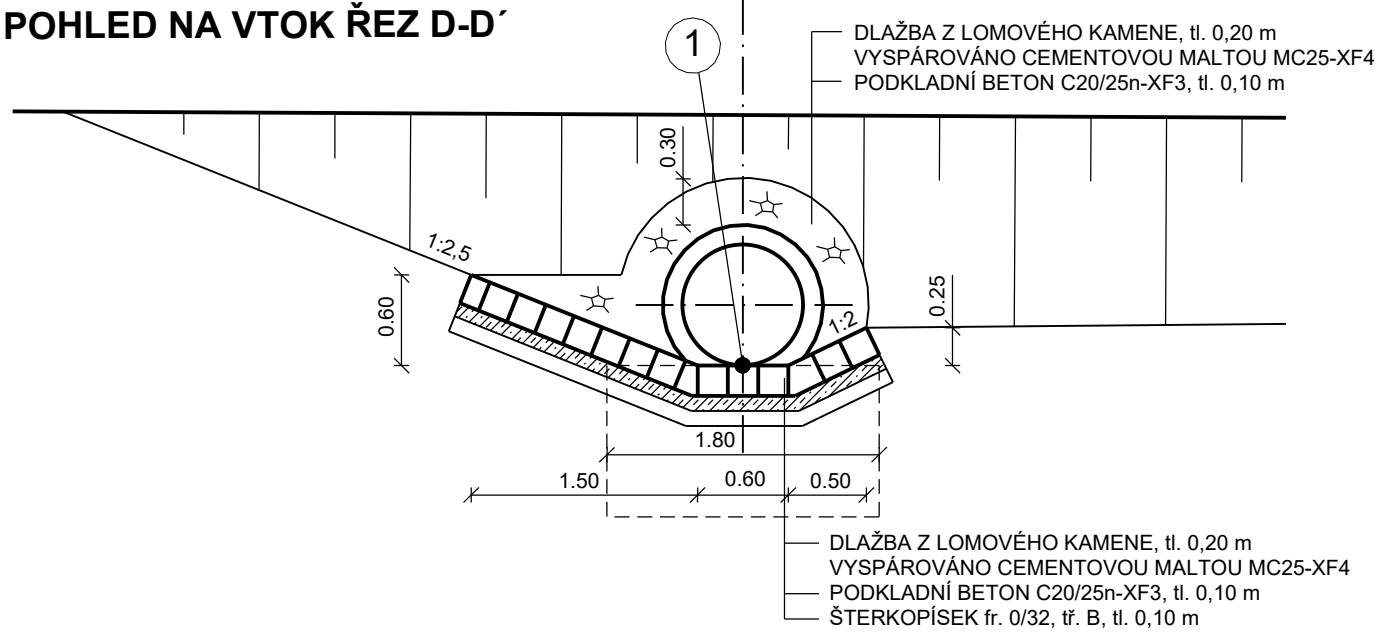
POHLED NA VTOK ŘEZ D-D'
