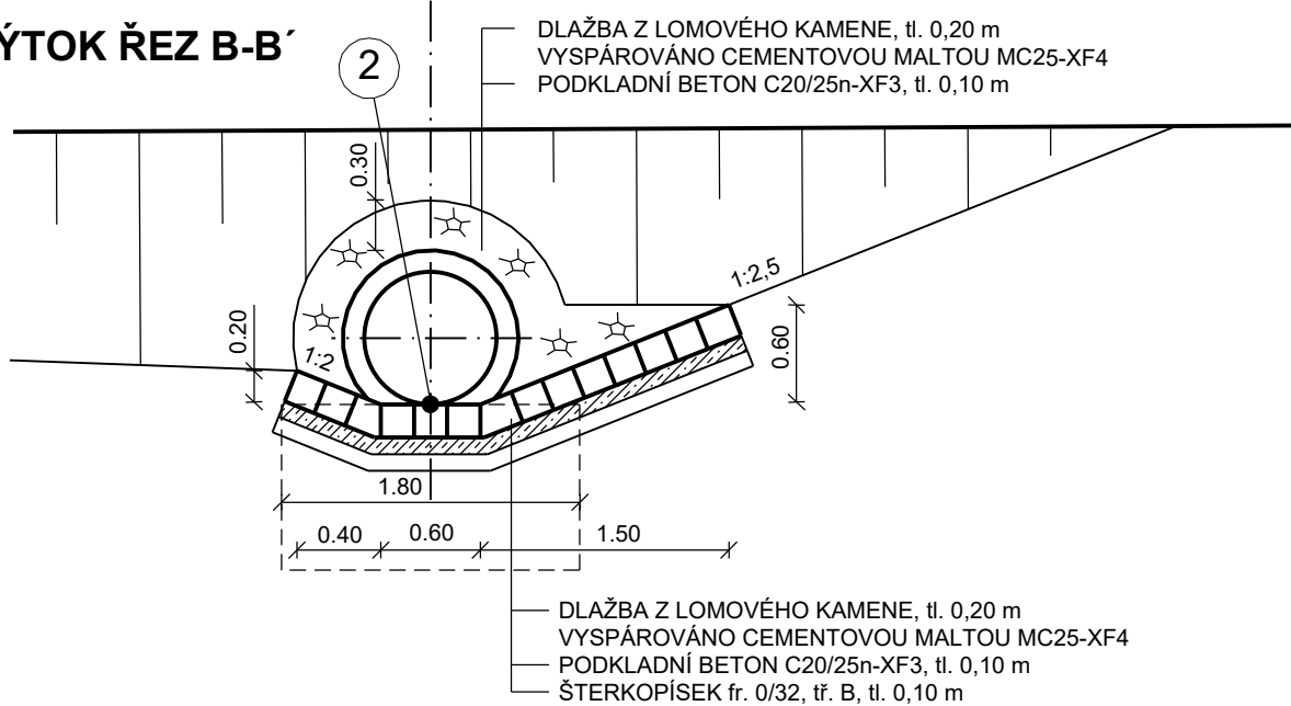
POHLED NA VÝTOK ŘEZ B-B'
