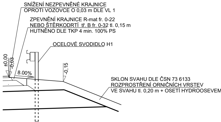
DETAIL V MÍSTĚ KRAJNICE
