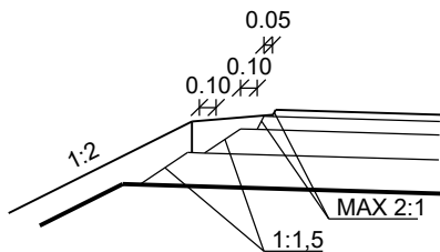
DETAIL UKONČENÍ VRSTEV VOZOVKY
