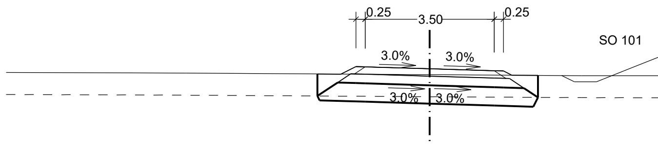
km 0 + 100.000
