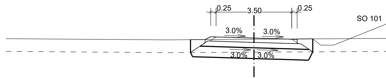
km 0 + 020.000
