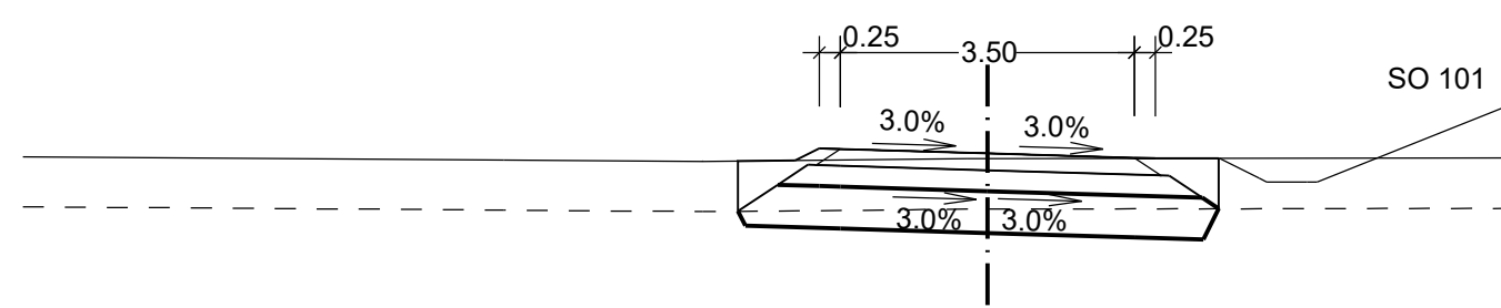
km 0 + 060.000
