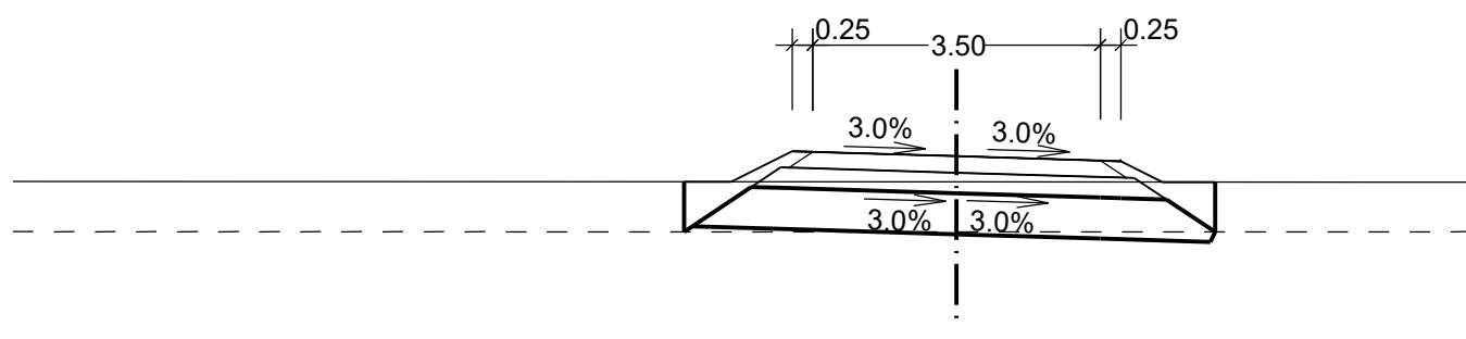
km 0 + 160.000
