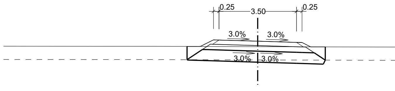
km 0 + 140.000
