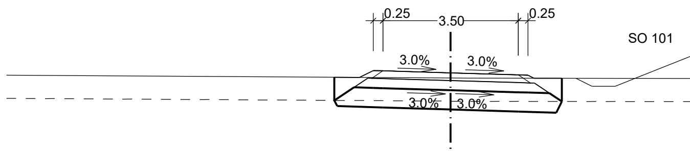
km 0 + 080.000
