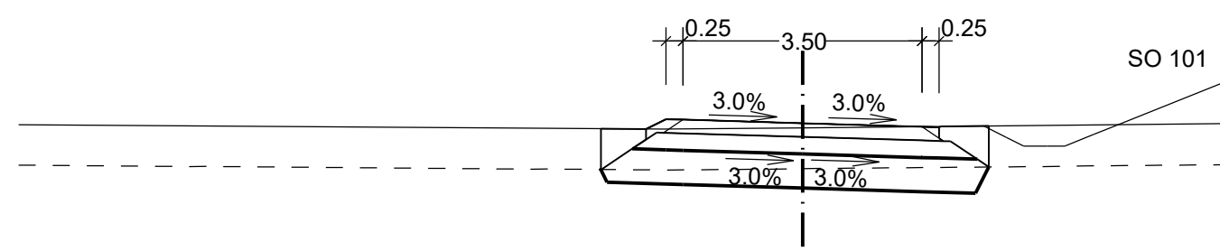
km 0 + 040.000
