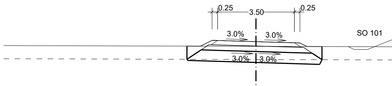
km 0 + 120.000
