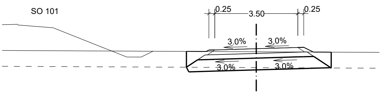
km 0 + 100.000
