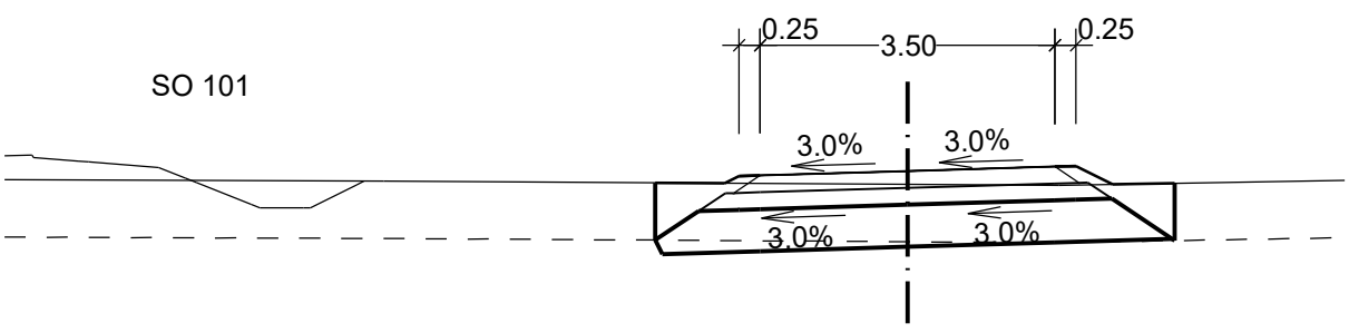
km 0 + 060.000
