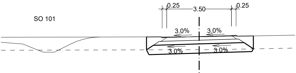
km 0 + 040.000
