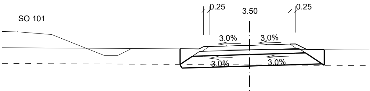
km 0 + 080.000
