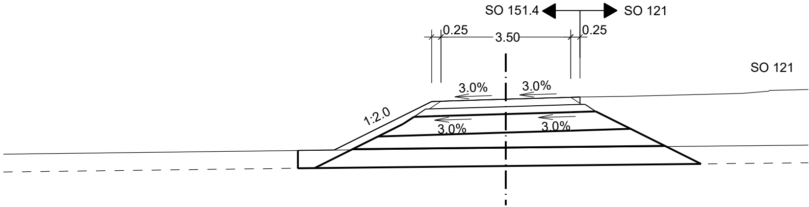
km 0 + 040.000
