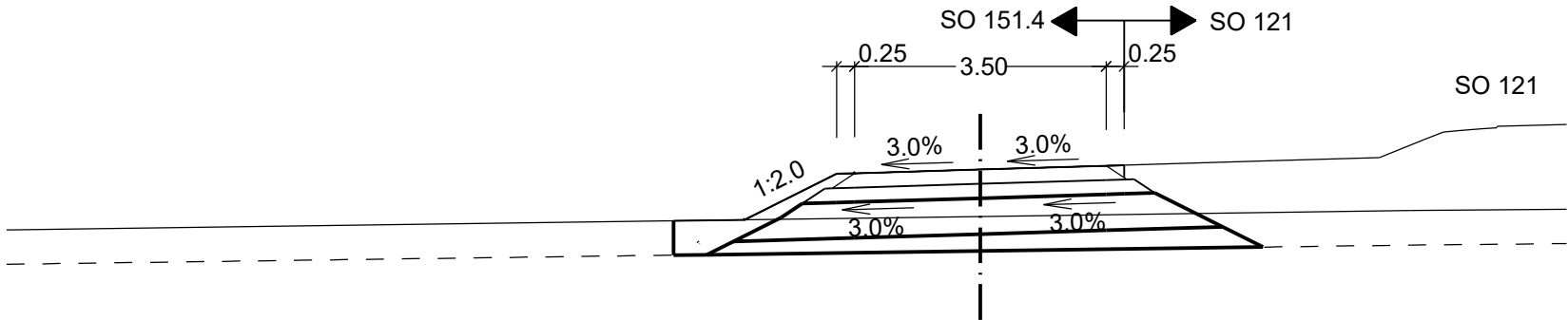
km 0 + 020.000
