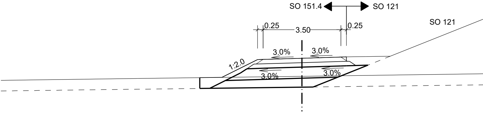
km 0 + 080.000
