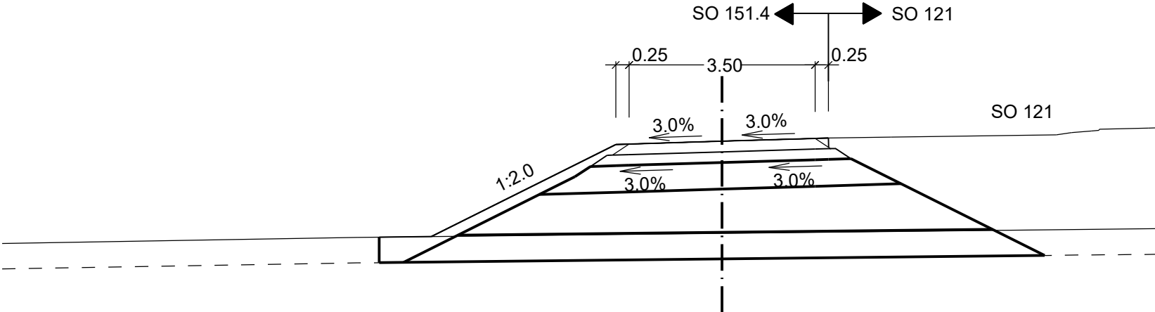
km 0 + 060.000
