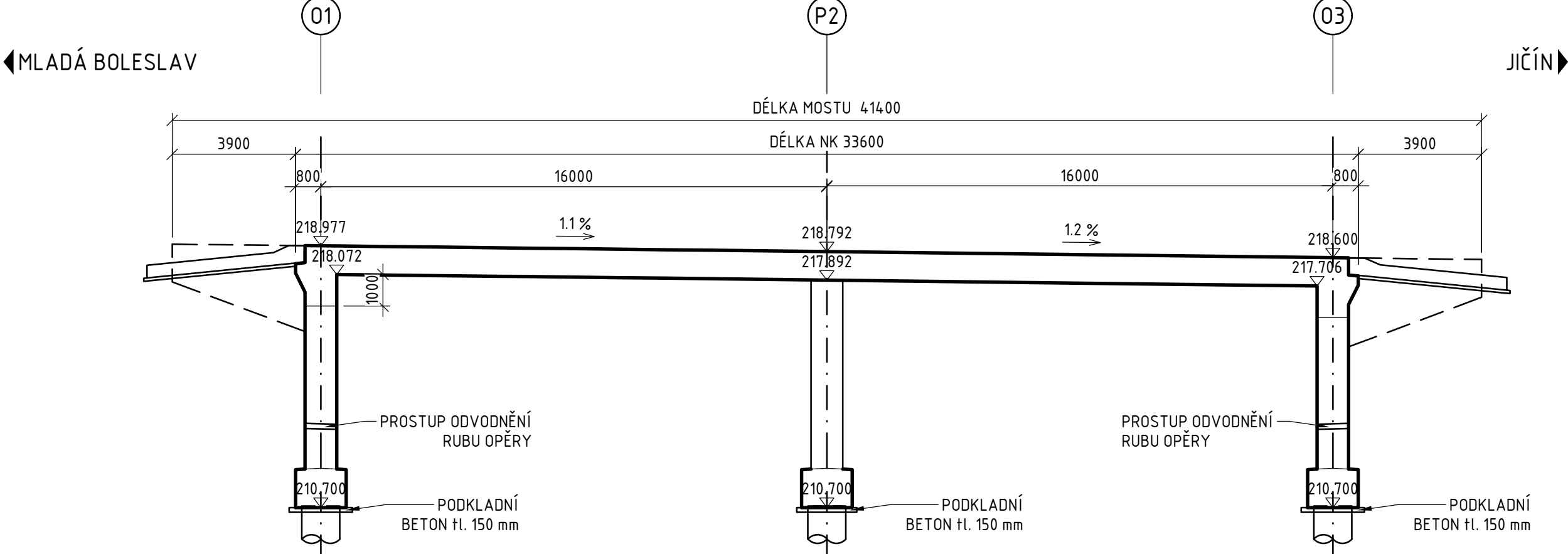
PODÉLNÝ ŘEZ 1:150 V OSE NIVELETY MOSTU
