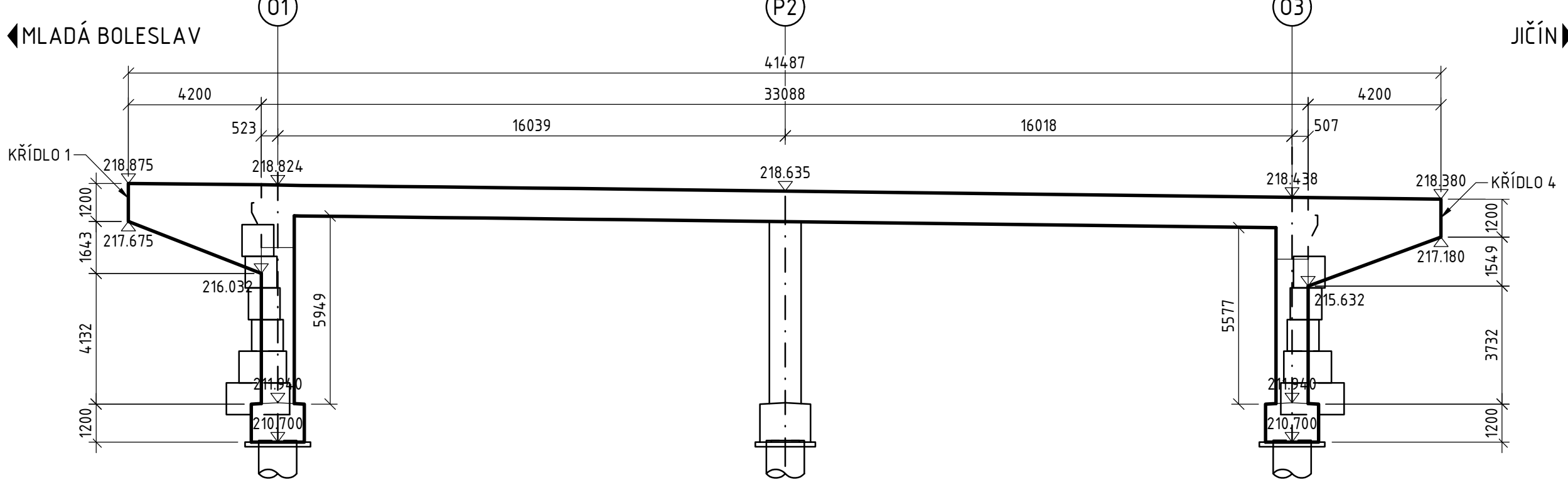
POHLED 1 1:150
