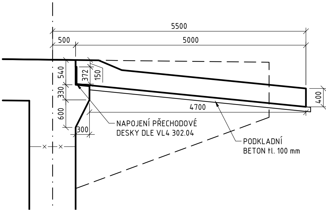
PODÉLNÝ ŘEZ PŘECHODOVOU DESKOU 1:50
