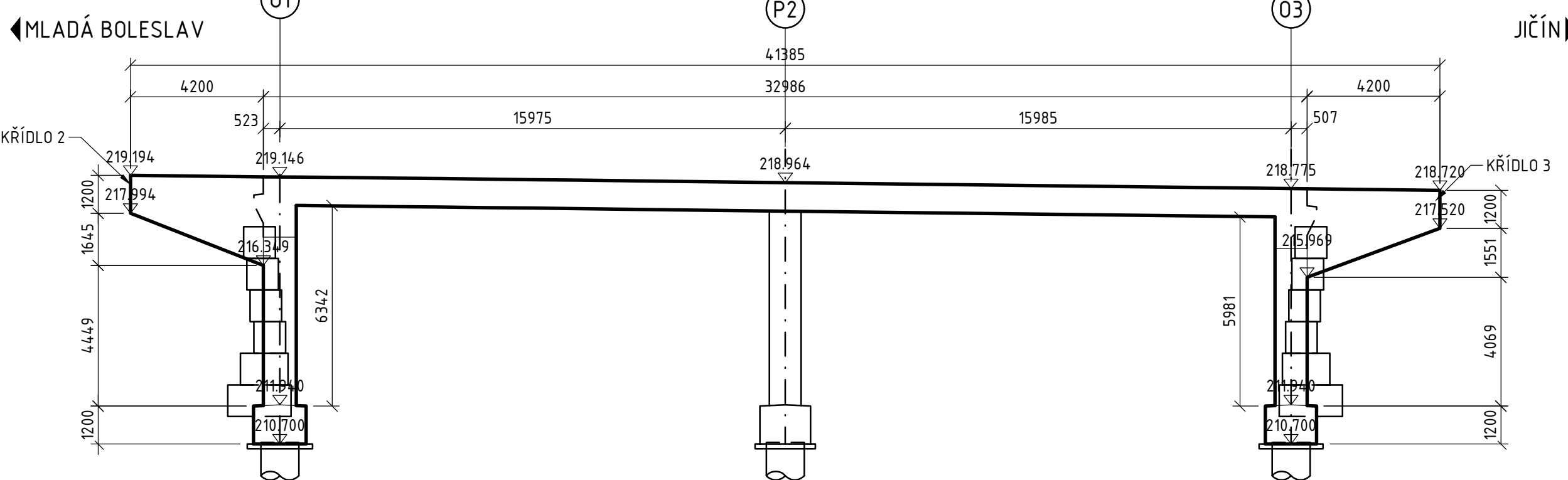
POHLED 2 1:150
