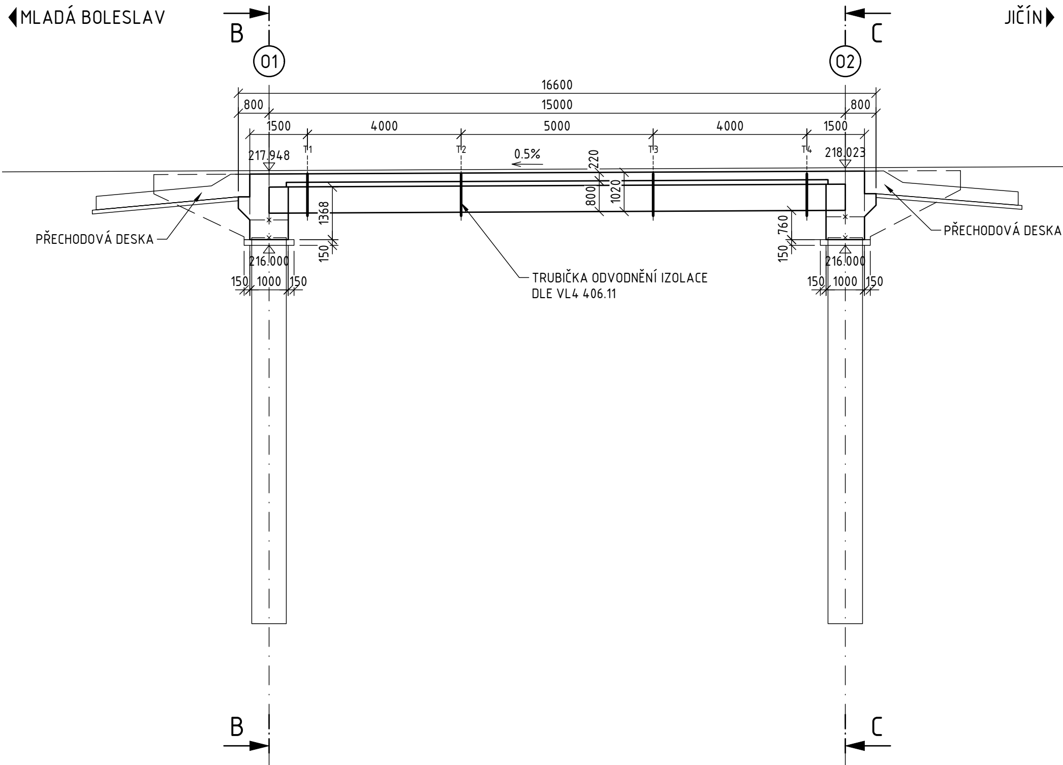
PODÉLNÝ ŘEZ 1:100
