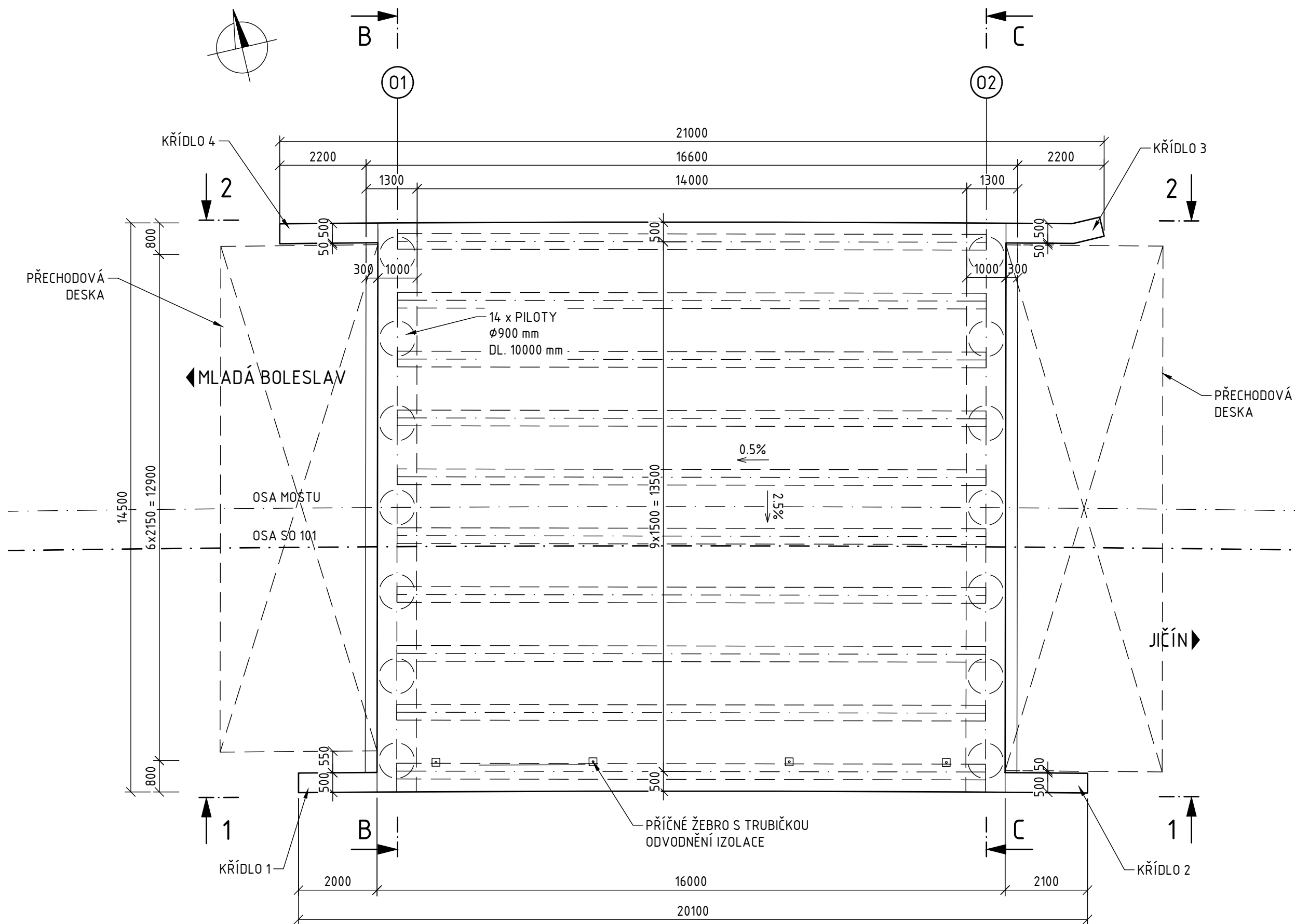
PŮDORYS 1:100
