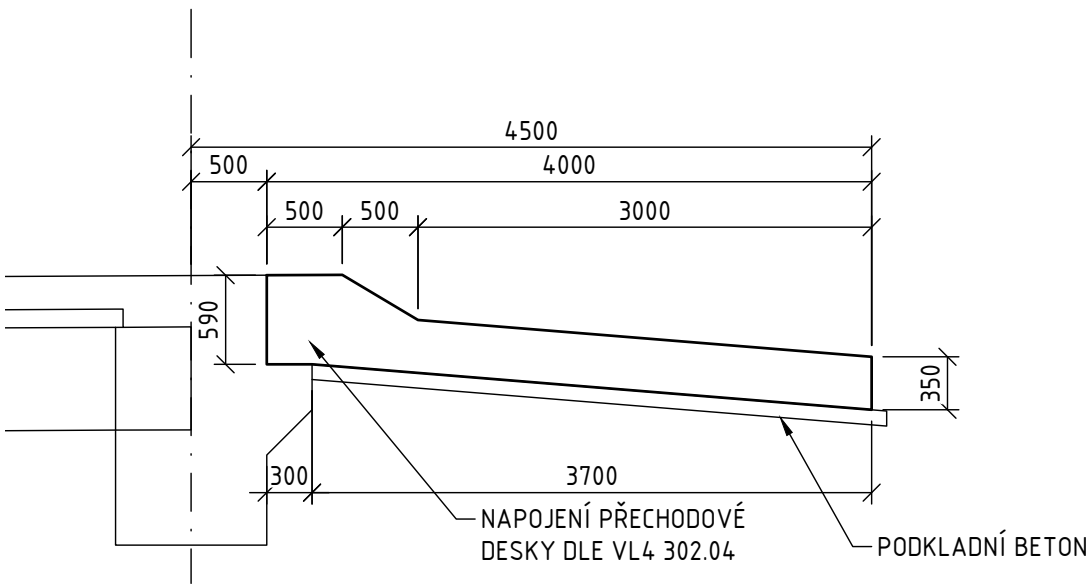
PODÉLNÝ ŘEZ PŘECHODOVOU DESKOU 1:50
