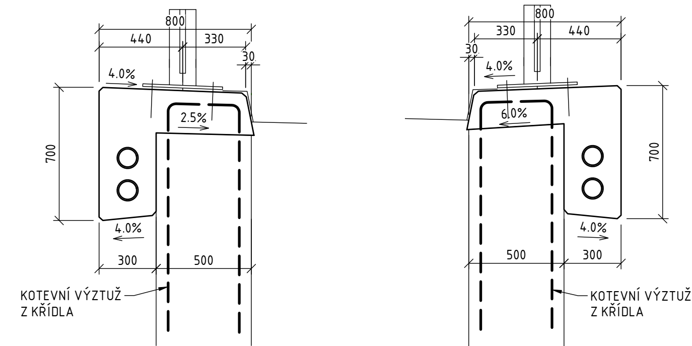
ŘEZ B-B 1:20
