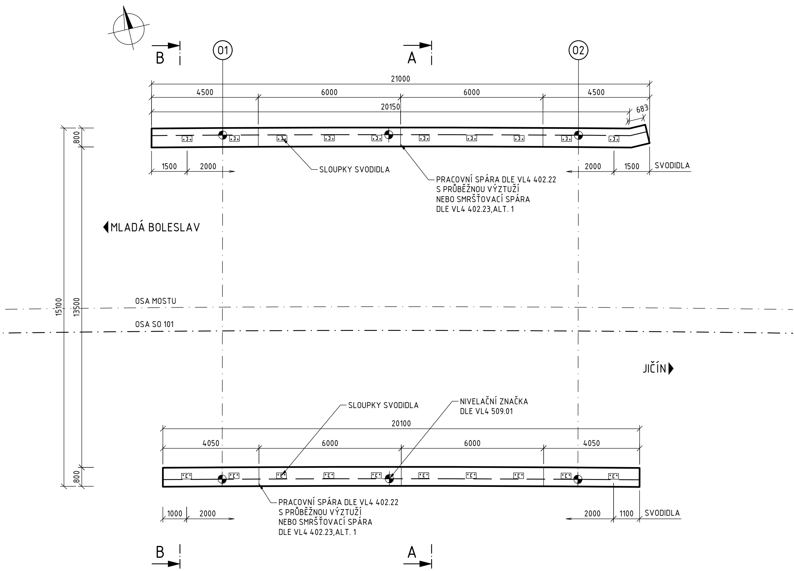
PŮDORYS 1:100
