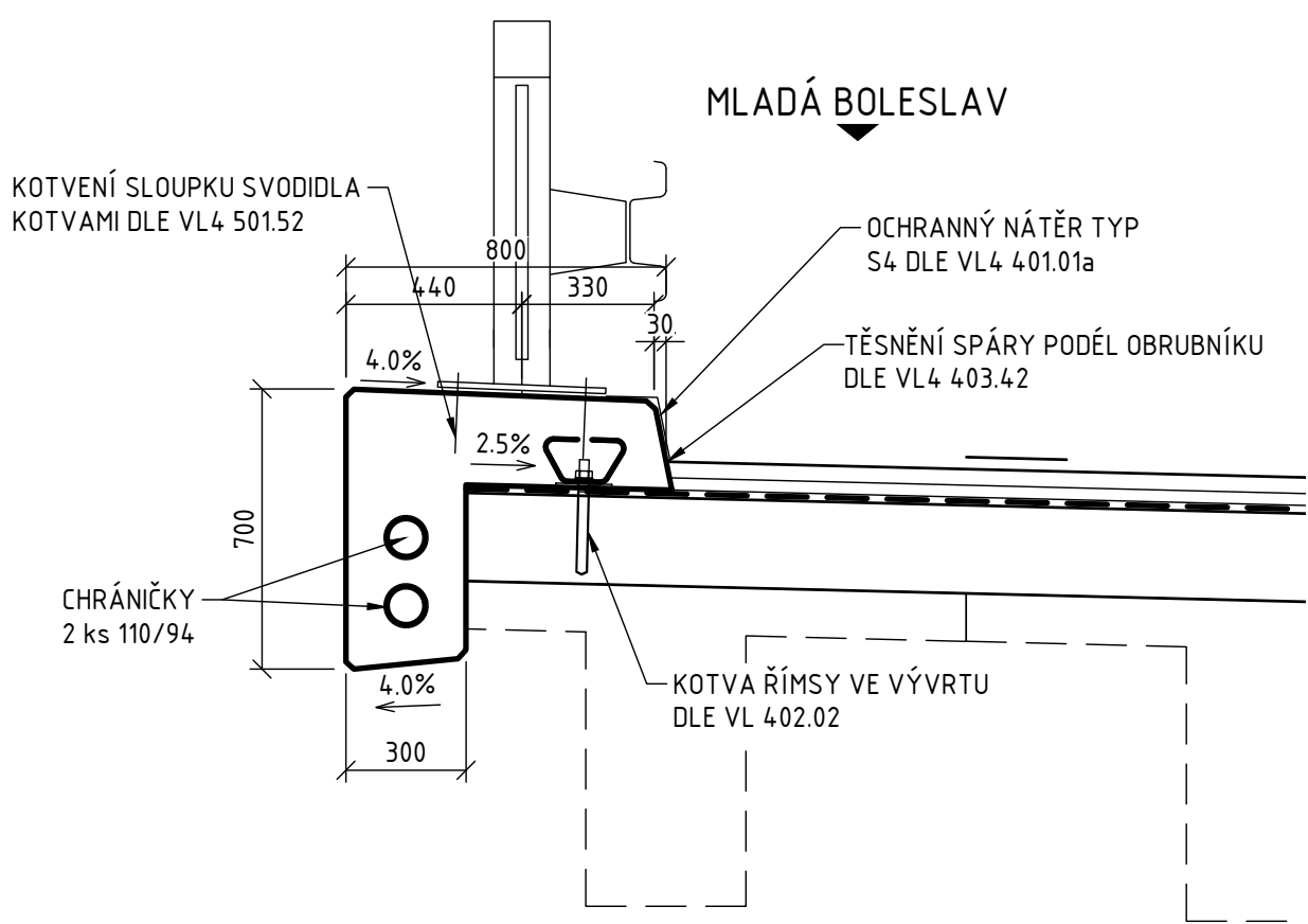
ŘEZ A-A 1:20
