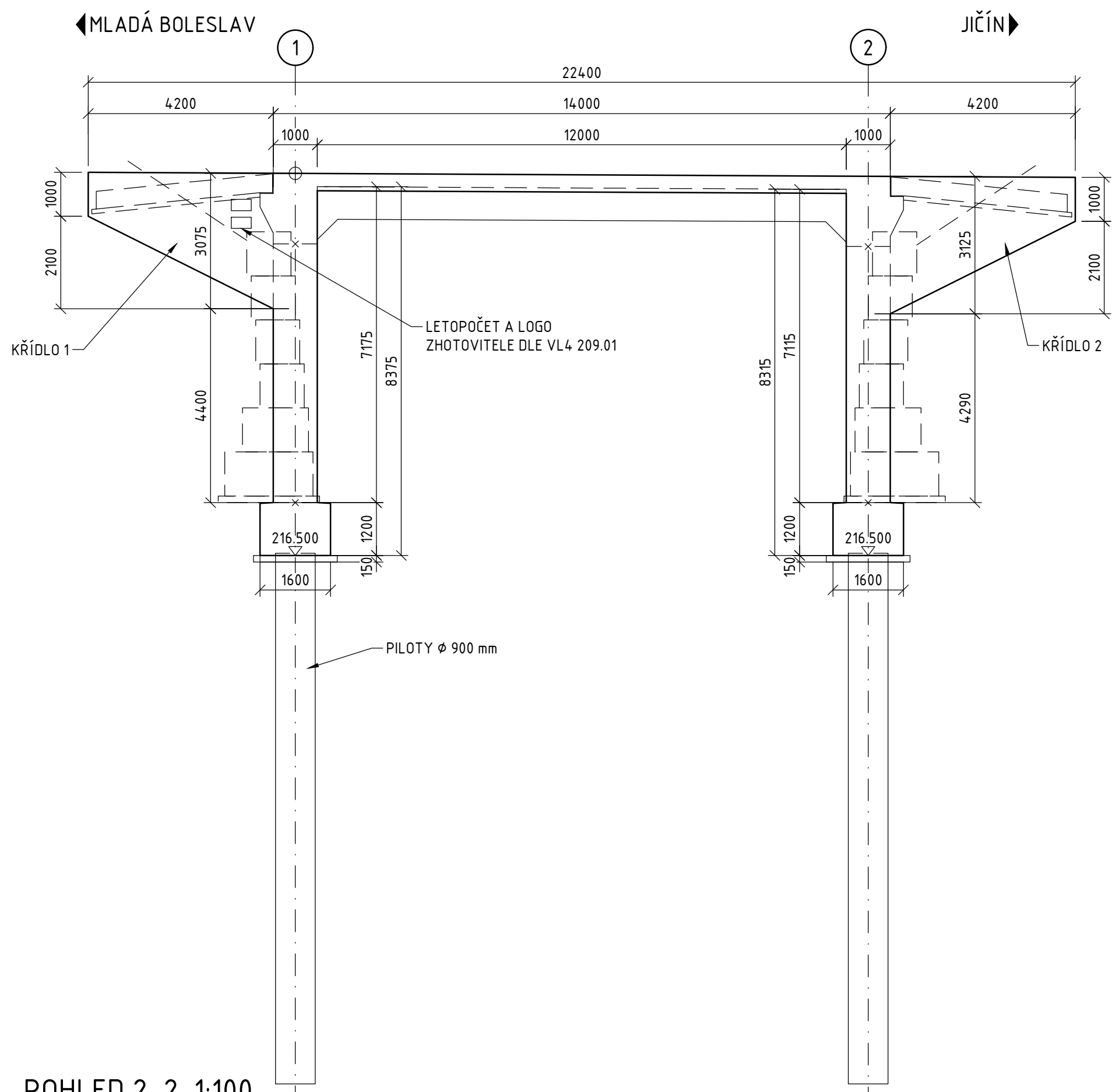
POHLED 2-2 1:100
