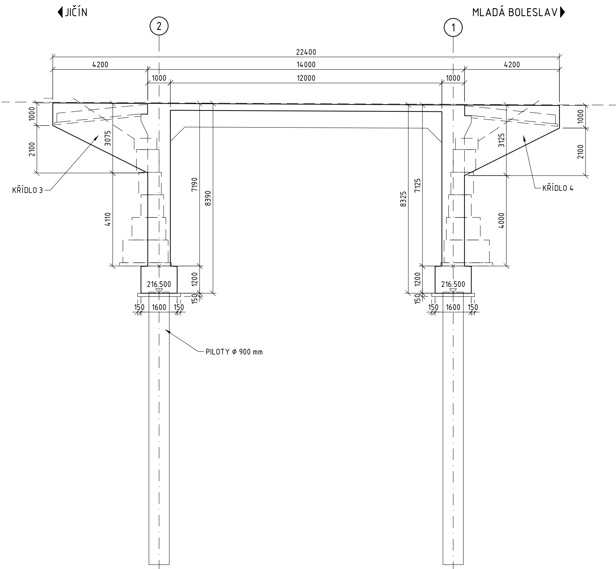
POHLED 2-2 1:100
