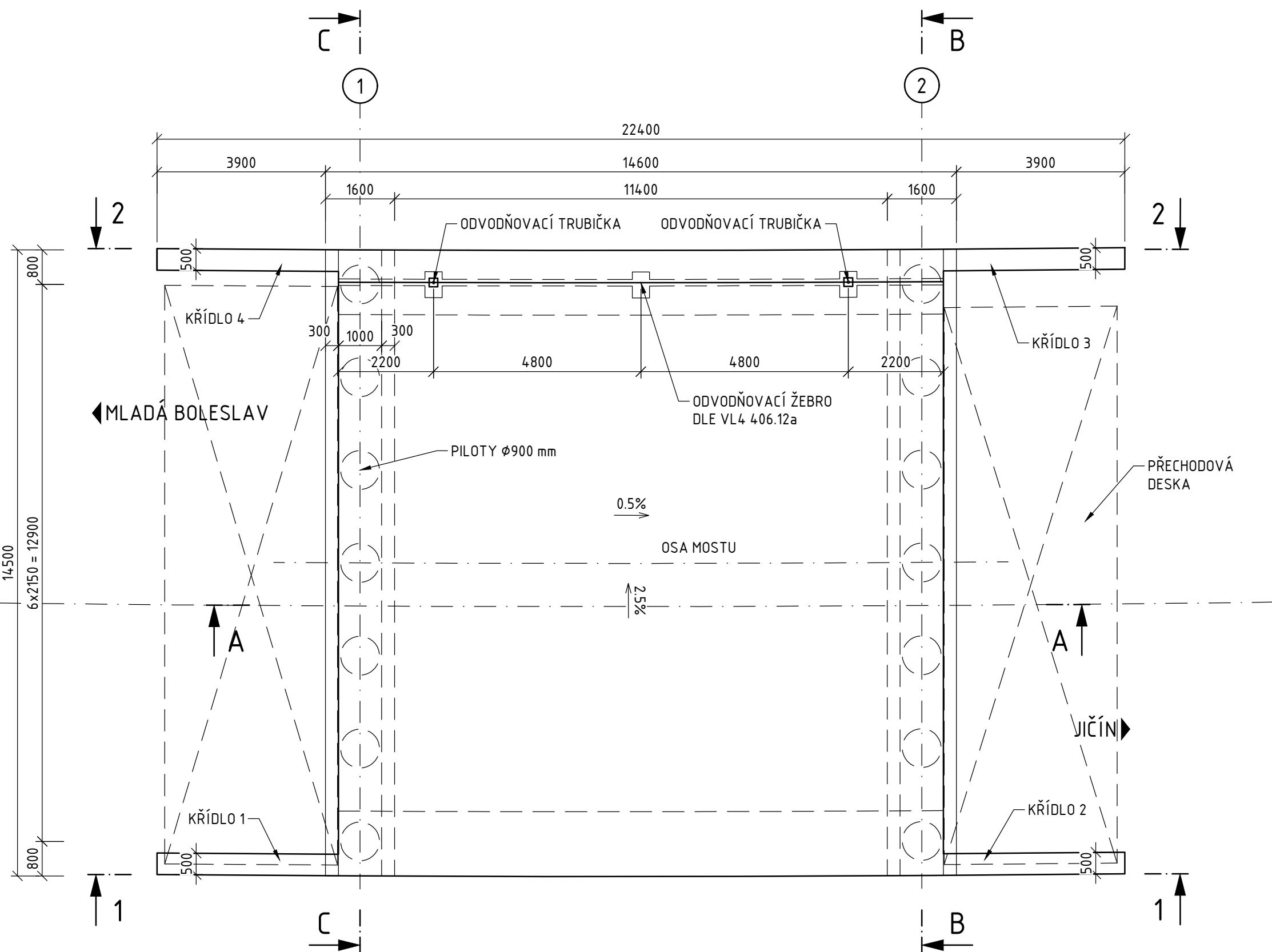
PŮDORYS 1:100
