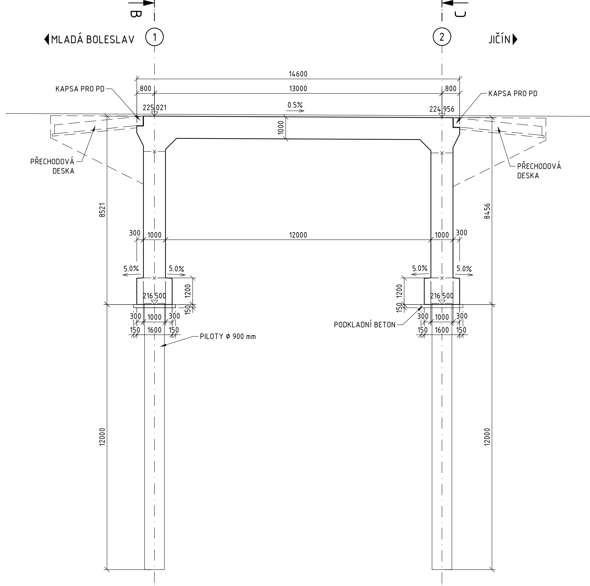
ŘEZ A-A 1:100
