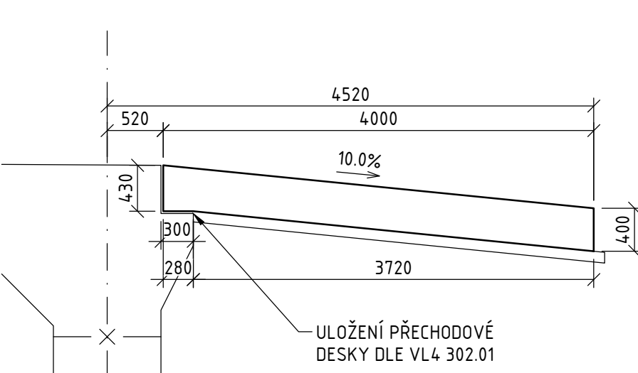
ŘEZ KŘÍDLEM 1, 2, 3, 4
