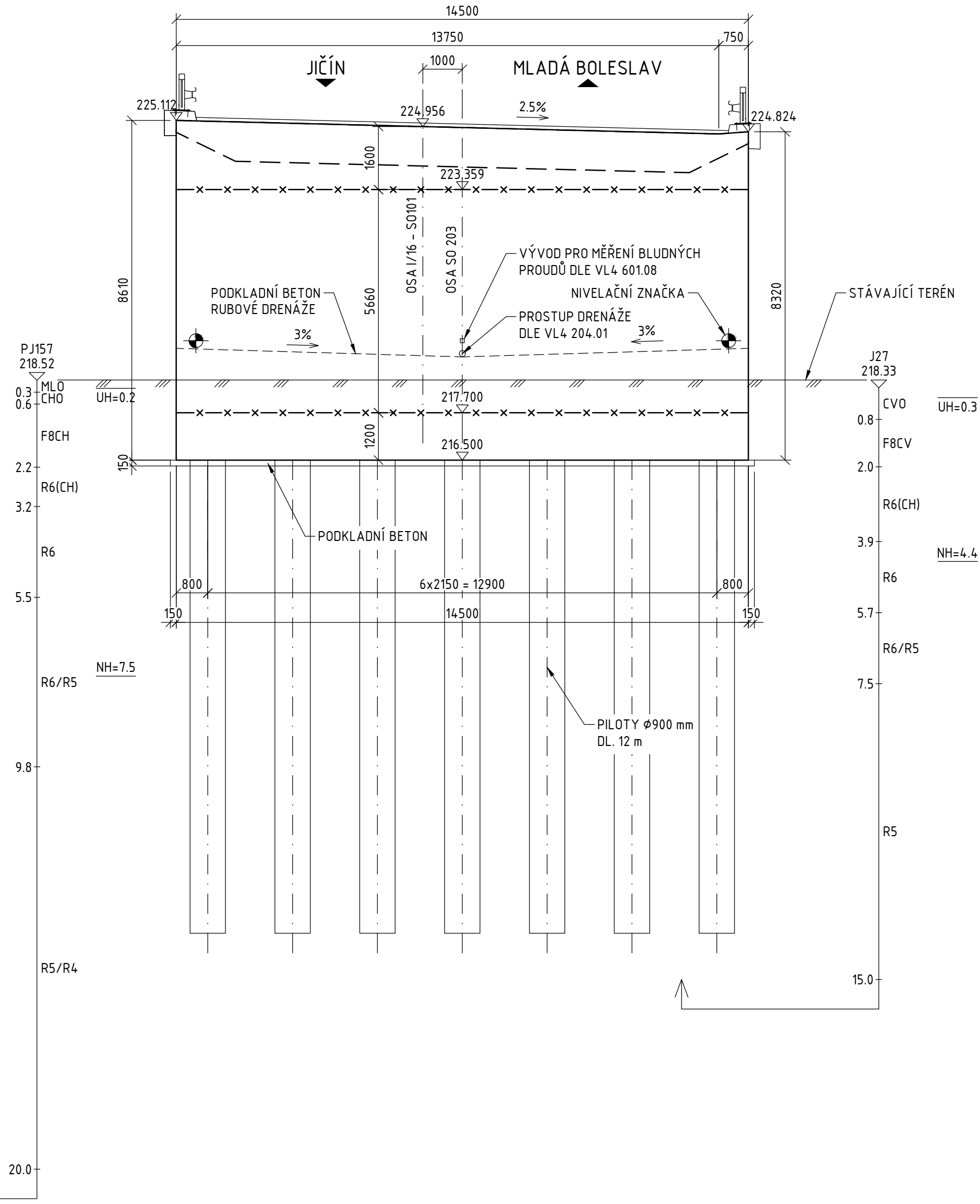
ŘEZ C-C 1:100
