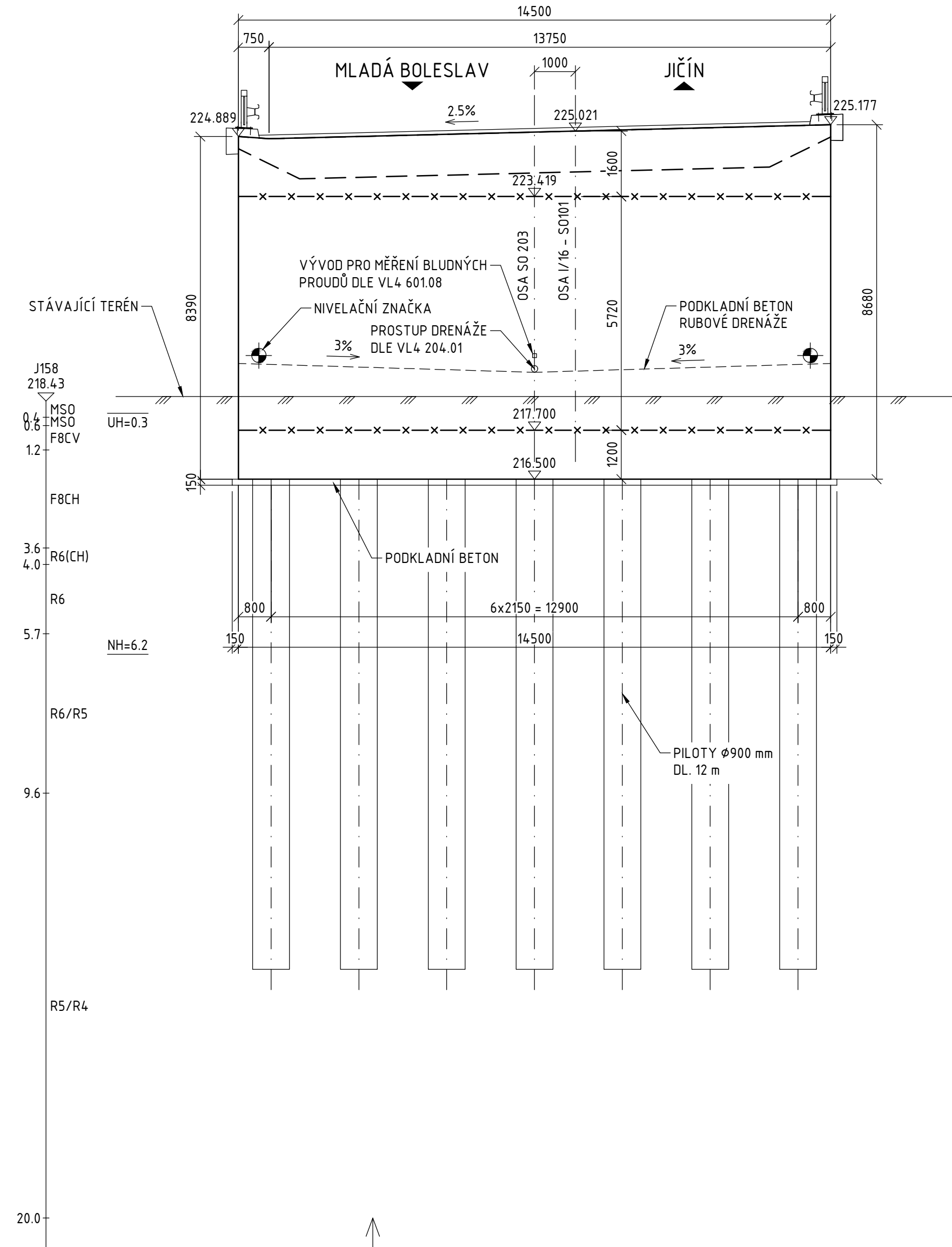
ŘEZ B-B 1:100
