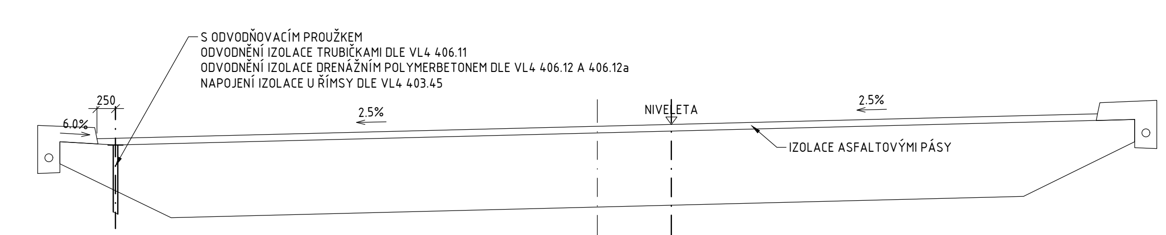
PŘÍČNÝ ŘEZ 1:50
