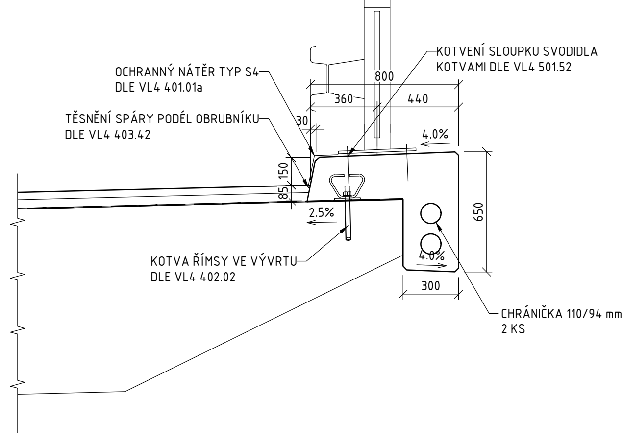
ŘEZ A-A 1:20
