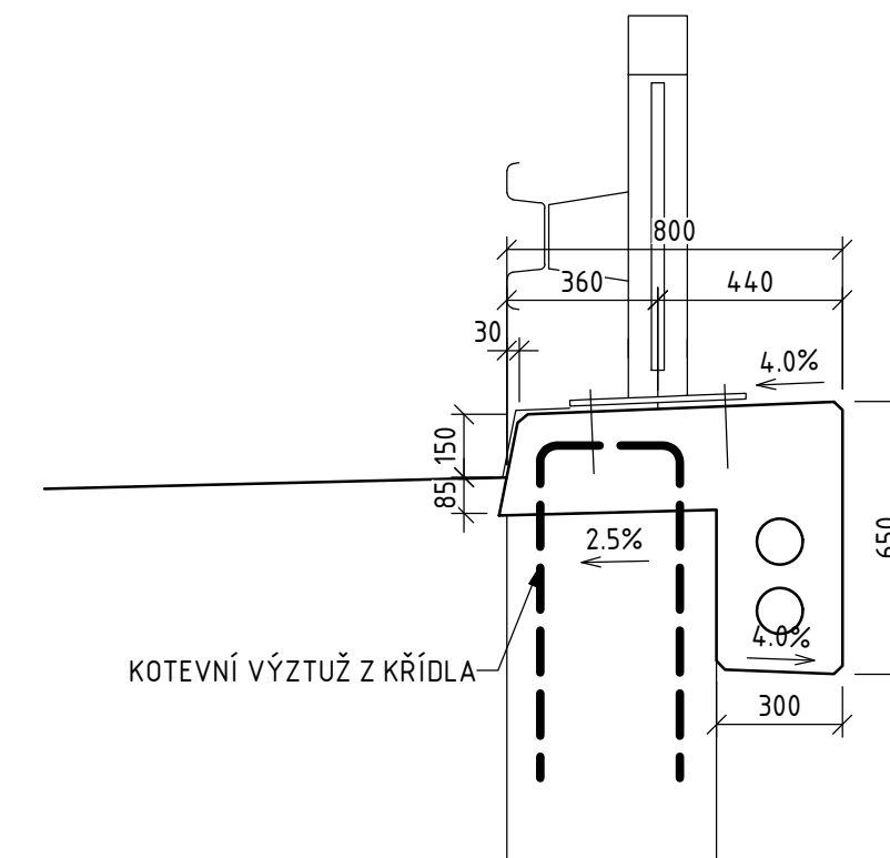
ŘEZ B-B 1:20
