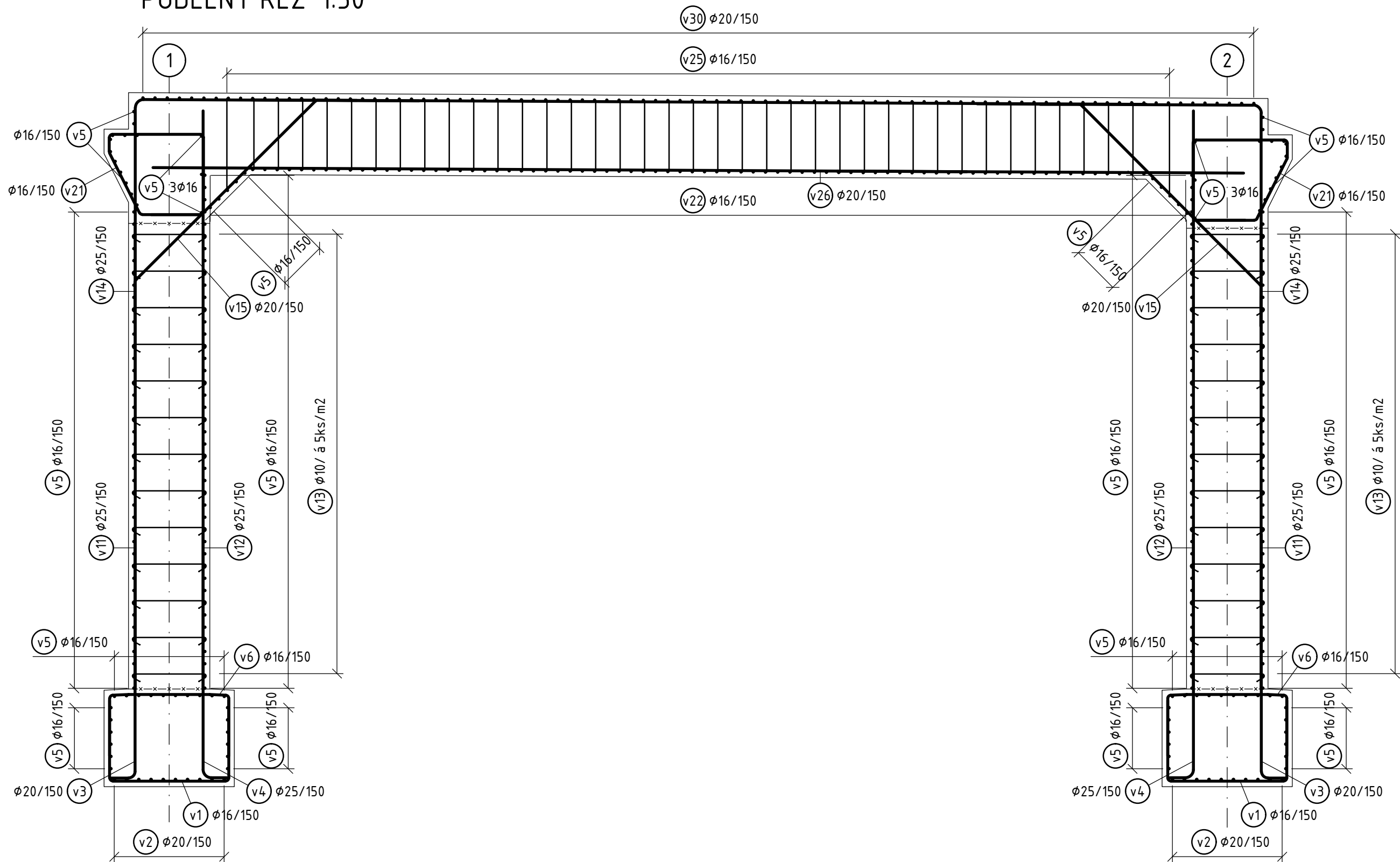
PODÉLNÝ ŘEZ 1:50
