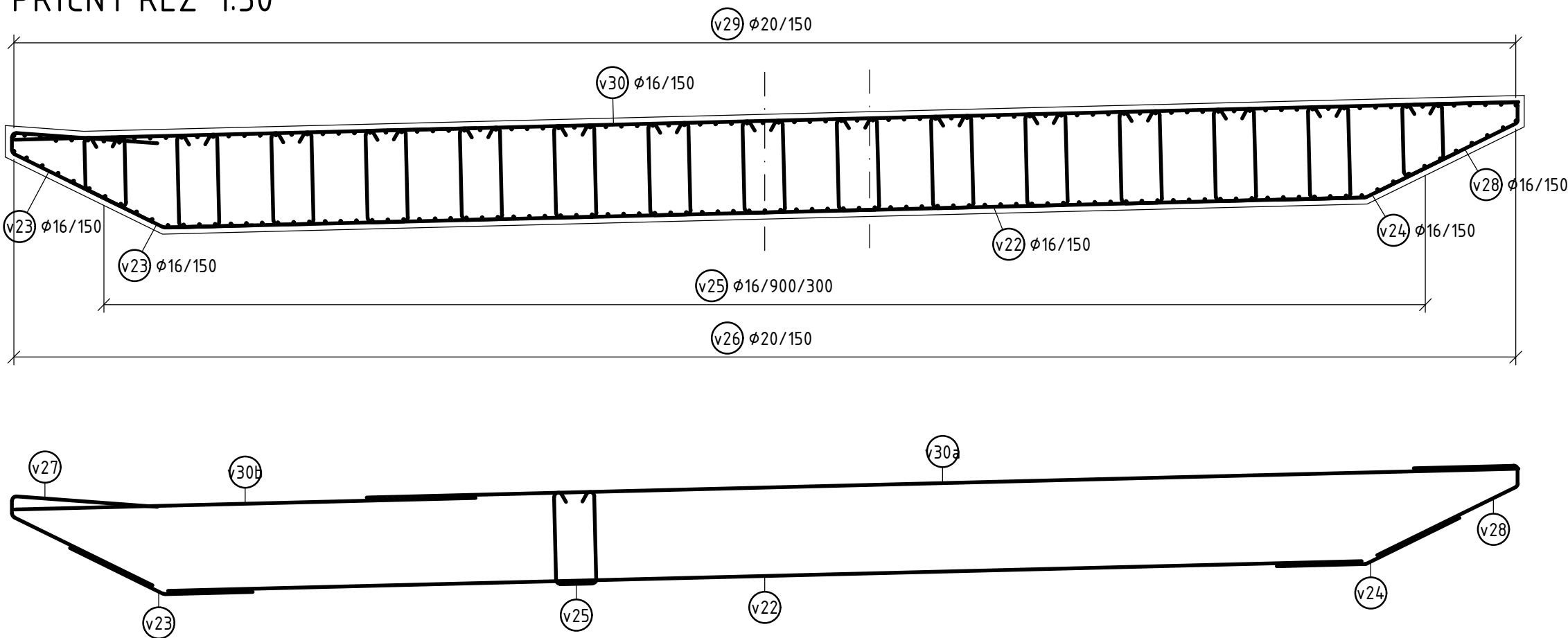
PŘÍČNÝ ŘEZ 1:50
