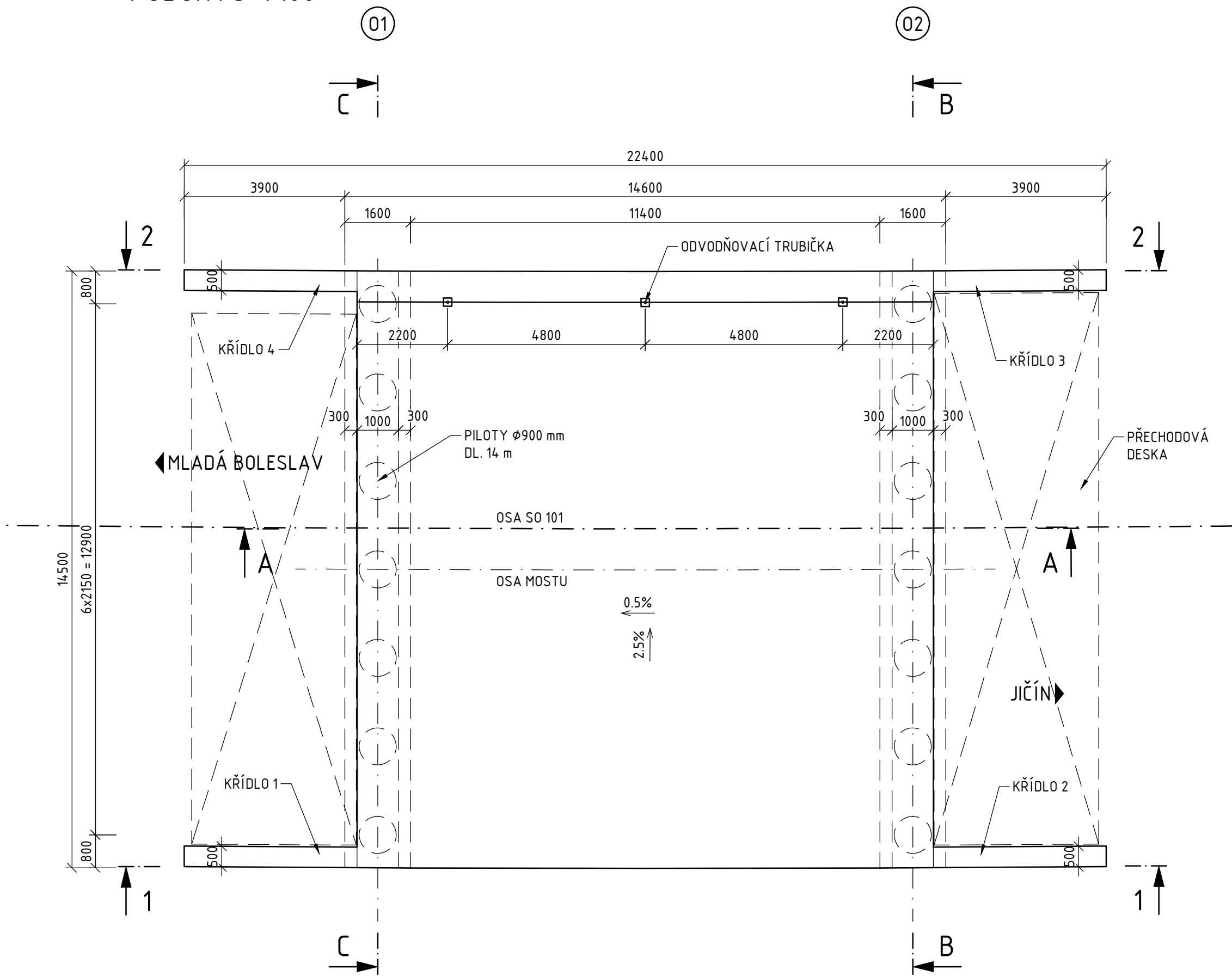
PŮDORYS 1:100
