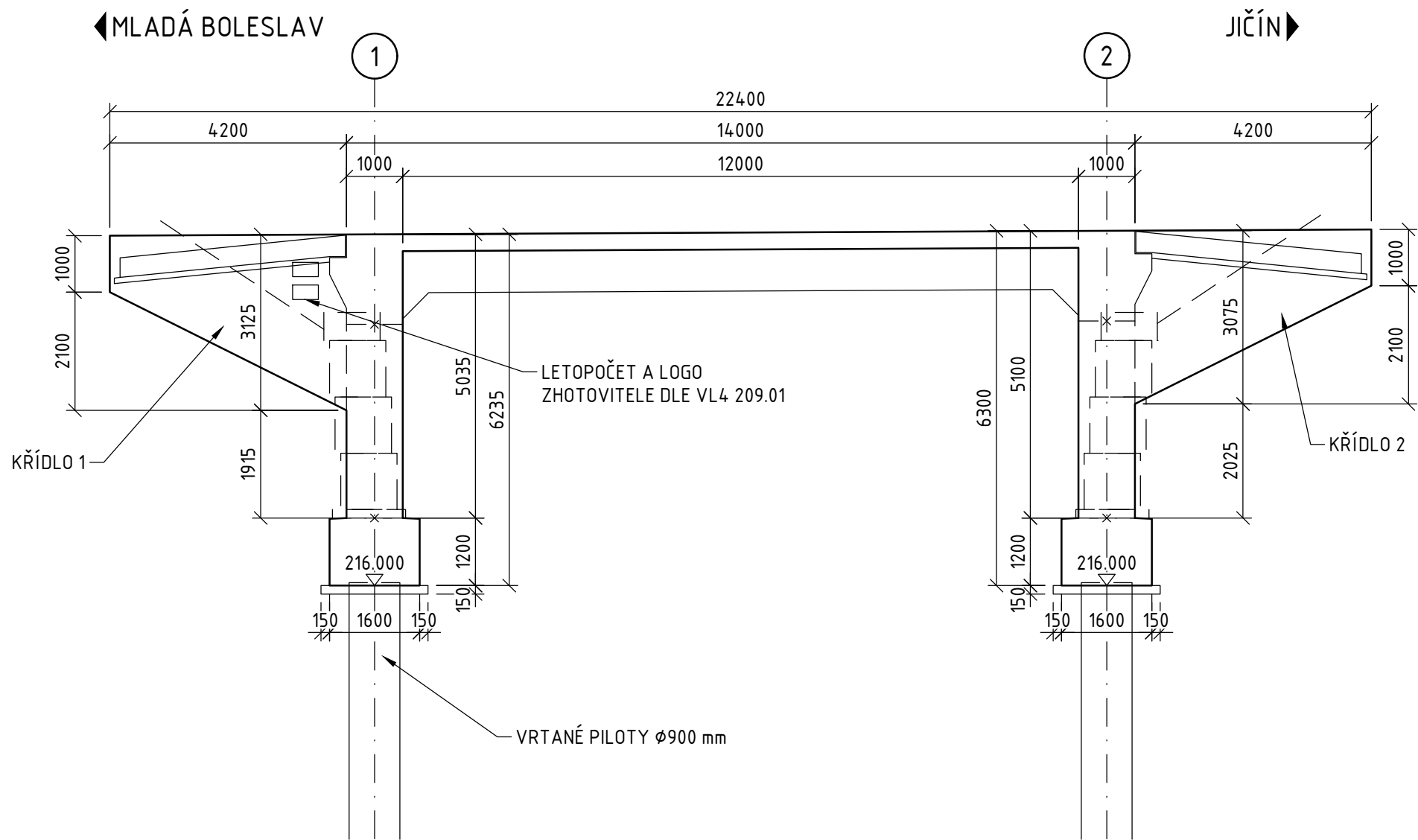
POHLED 1-1 1:100
