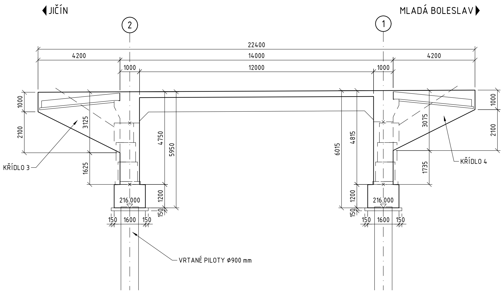
POHLED 2-2 1:100
