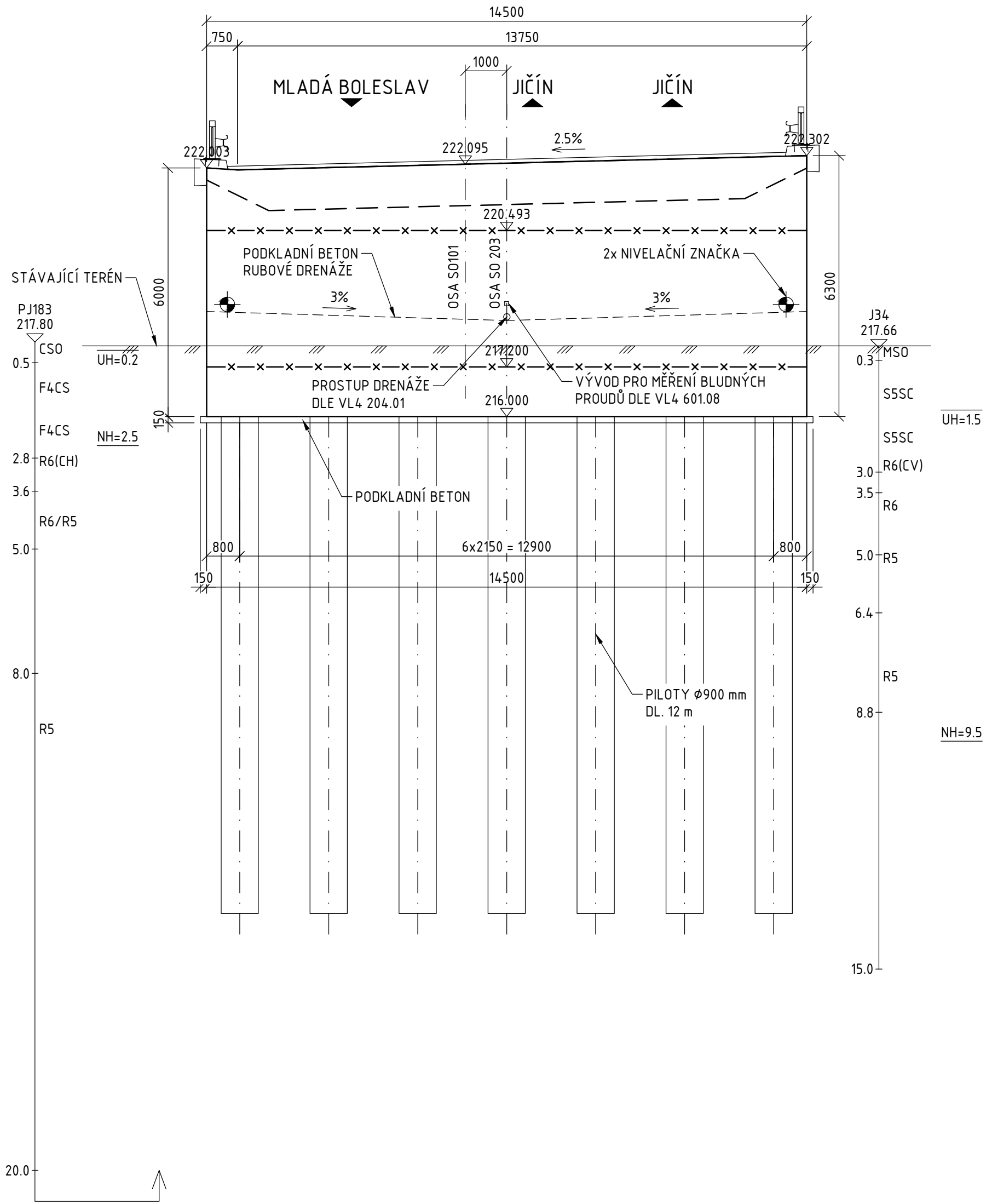
ŘEZ B-B 1:100
