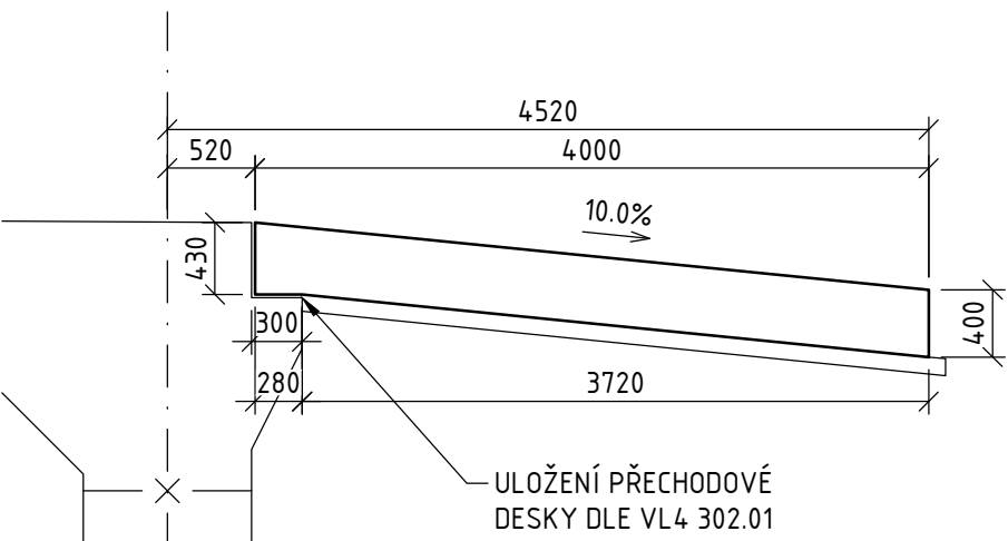
PODÉLNÝ ŘEZ PŘECHODOVOU DESKOU 1:50 VYKRESLENA PŘECHODOVÁ DESKA OPĚRY 2, PŘECHODOVÁ DESKA OPĚRY 1 ŘEŠENA OBDOBNĚ
