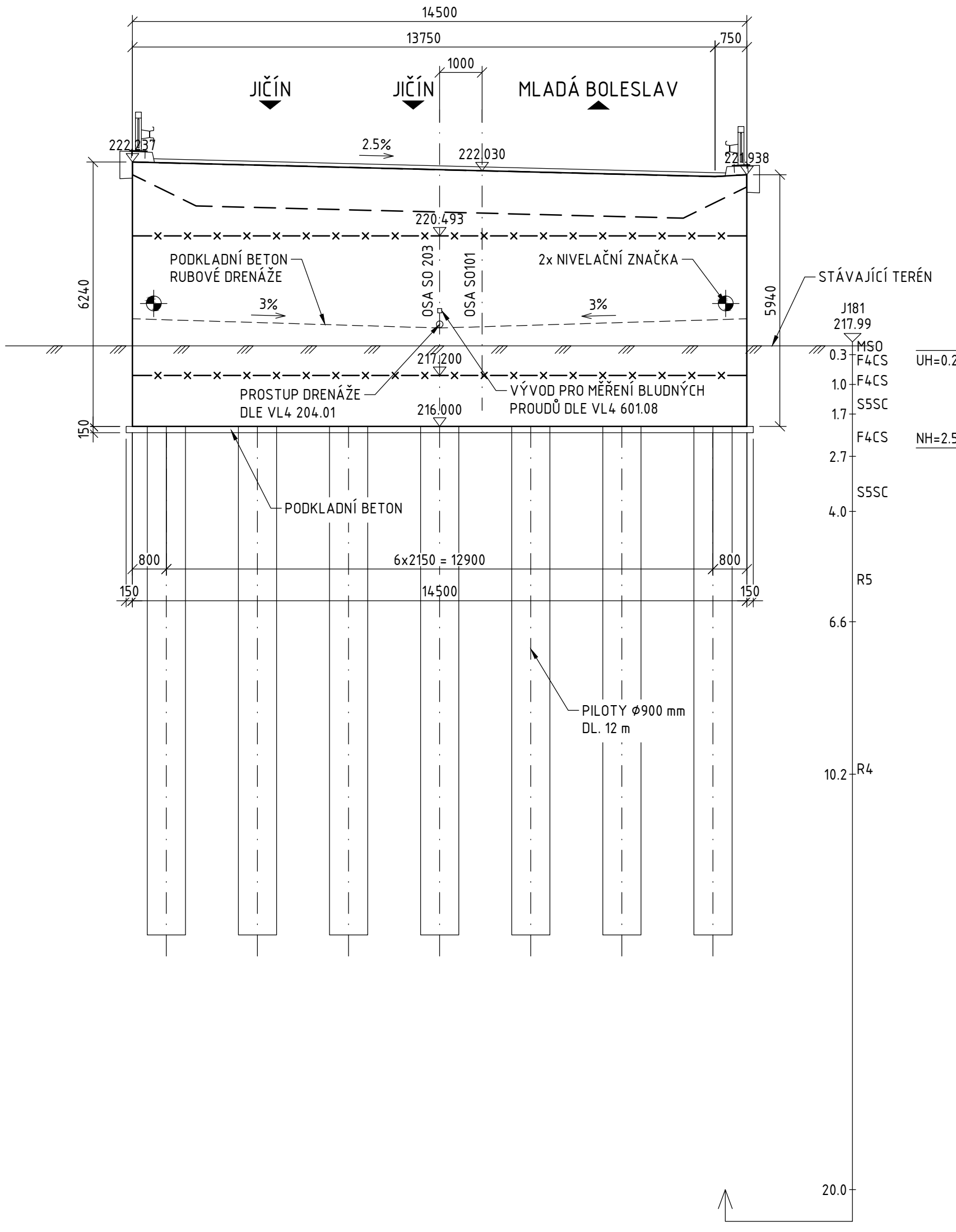
ŘEZ C-C 1:100
