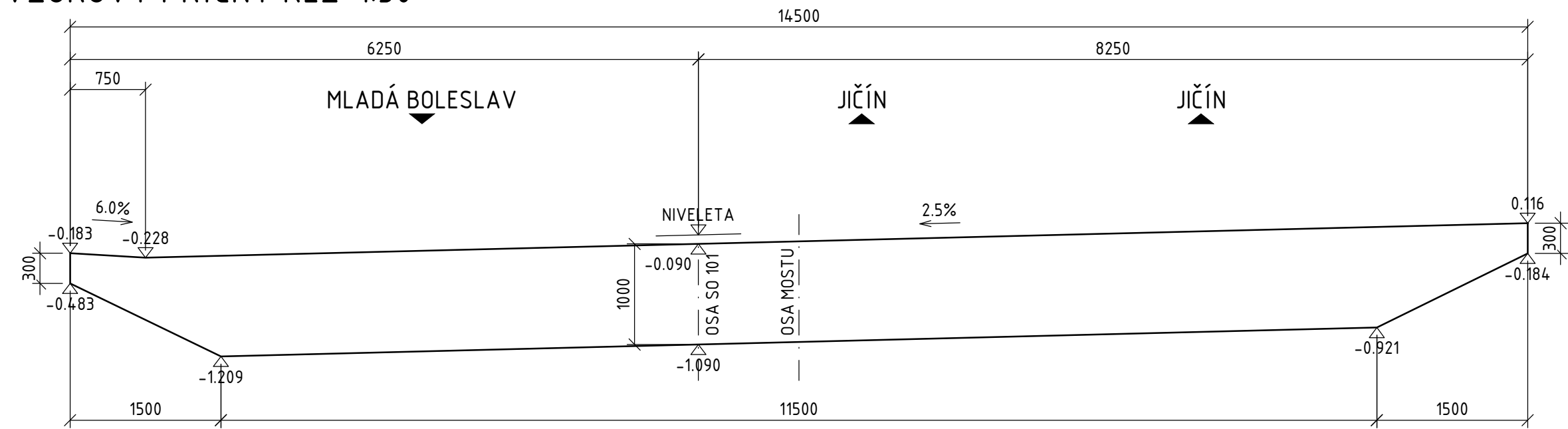
VZOROVÝ PŘÍČNÝ ŘEZ 1:50
