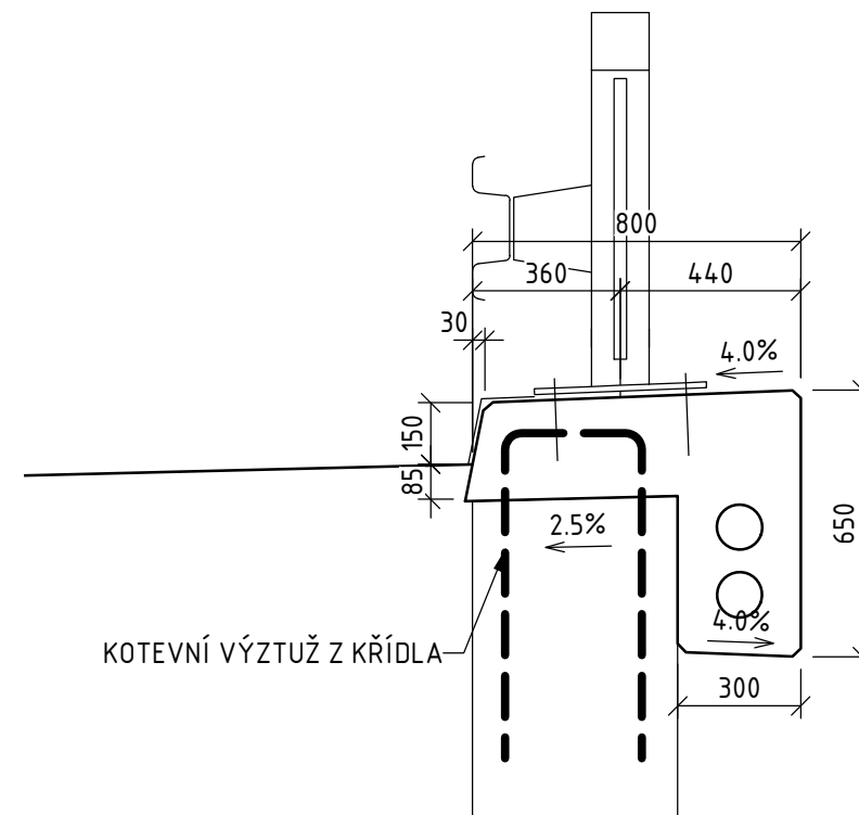
ŘEZ B-B 1:20
