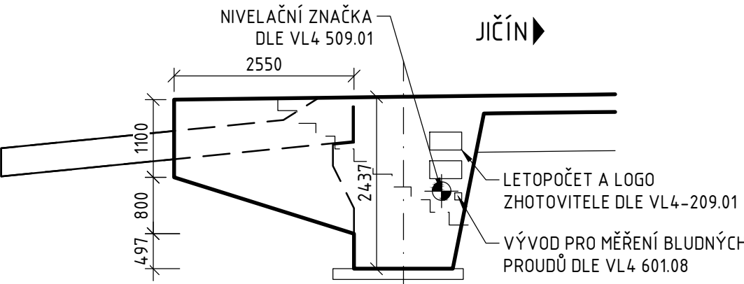
POHLED NA KŘÍDLO 01 VPRAVO 1:75
