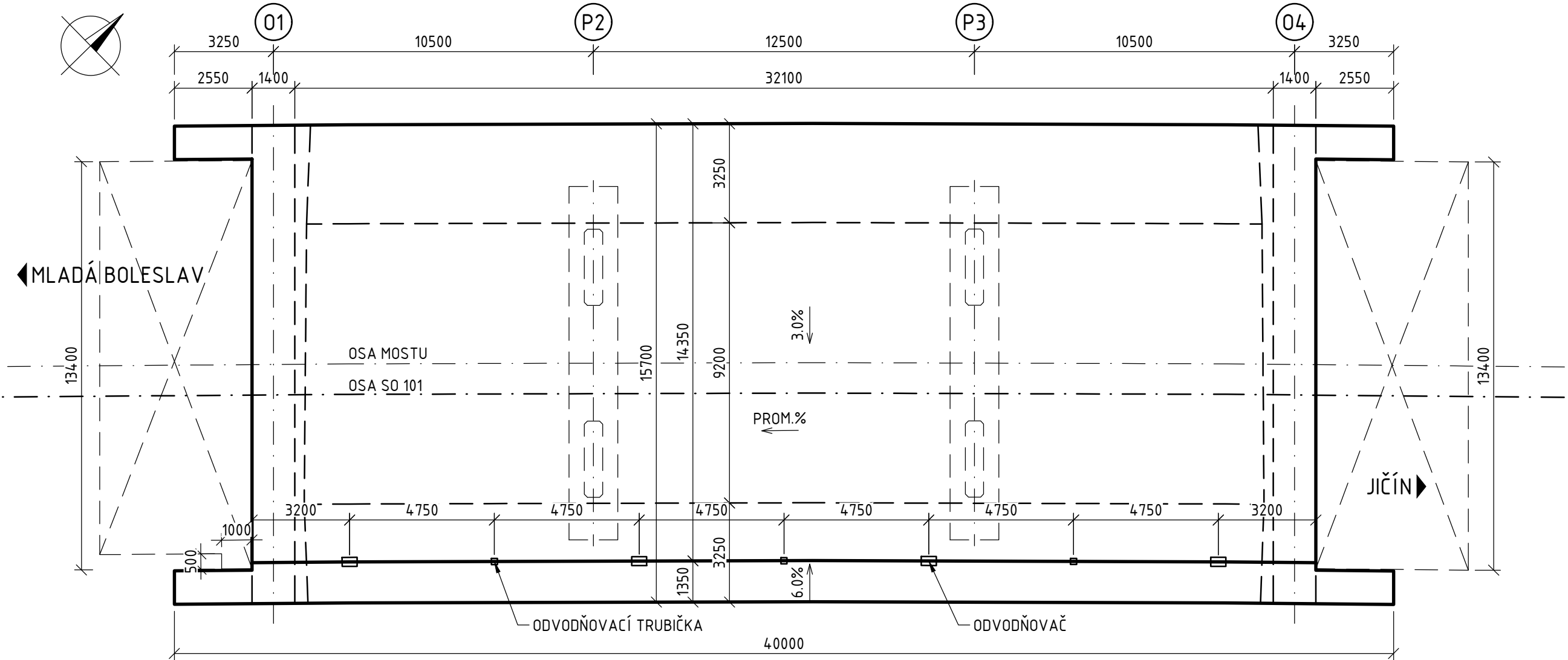
PŮDORYS 1:150
