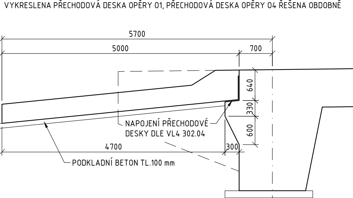
PODÉLNÝ ŘEZ PŘECHODOVOU DESKOU 1:50
