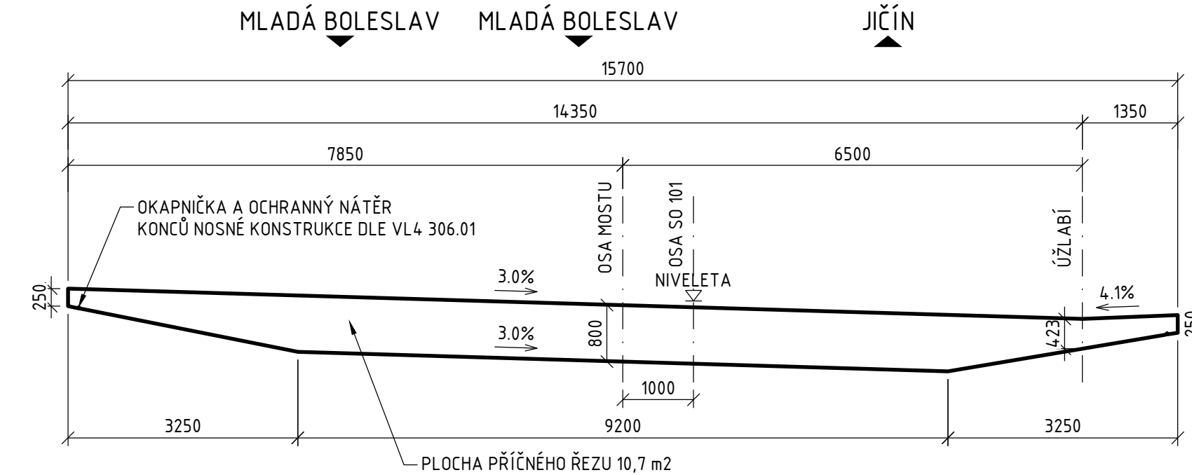
PŘÍČNÝ ŘEZ 1:75
