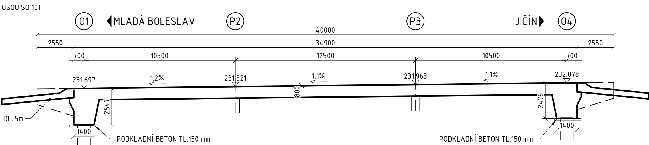
PODÉLNÝ ŘEZ 1:150
