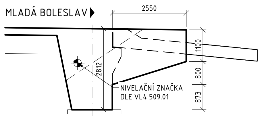
POHLED NA KŘÍDLO 01 VLEVO 1:75
