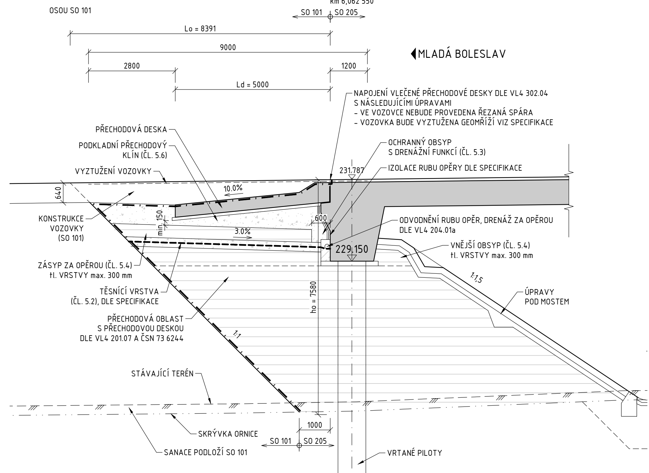
PODÉLNÝ ŘEZ 01 1:75
