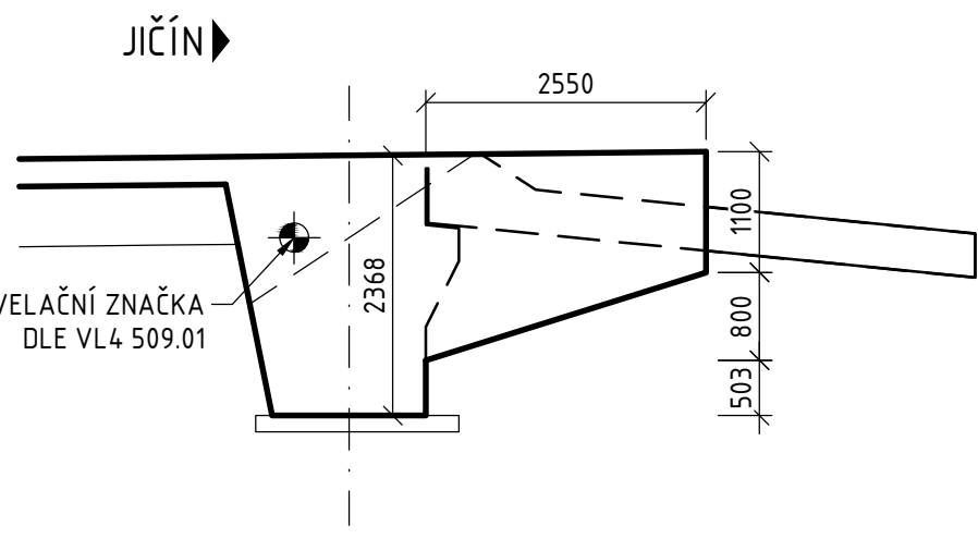
POHLED NA KŘÍDLO 04 VPRAVO 1:75
