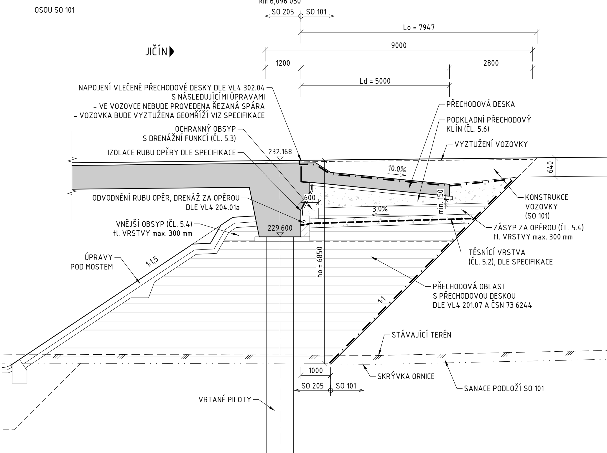
PODÉLNÝ ŘEZ 04 1:75
