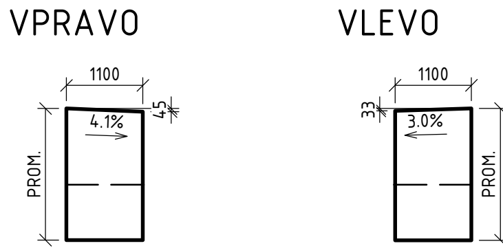
ŘEZ KŘÍDLEM 1:75
