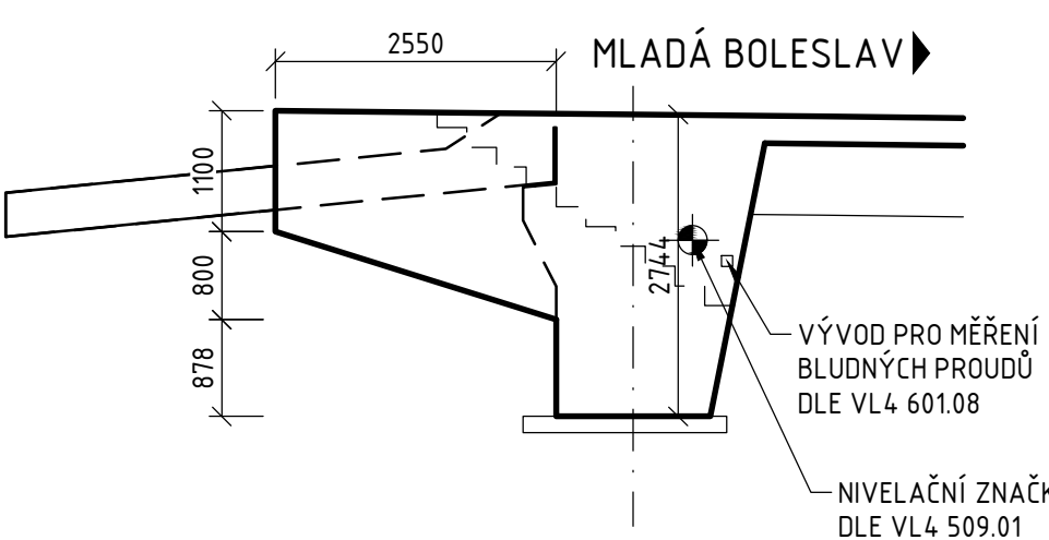
POHLED NA KŘÍDLO 04 VLEVO 1:75
