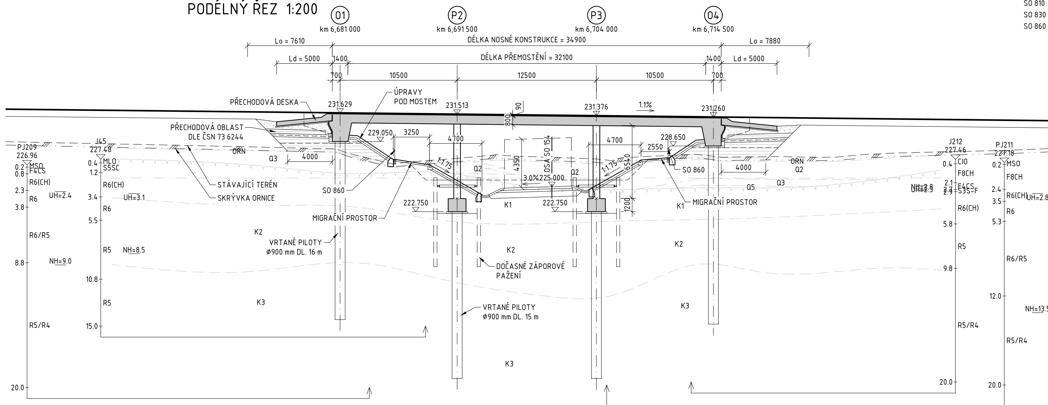
PODÉLNÝ ŘEZ 1:200
