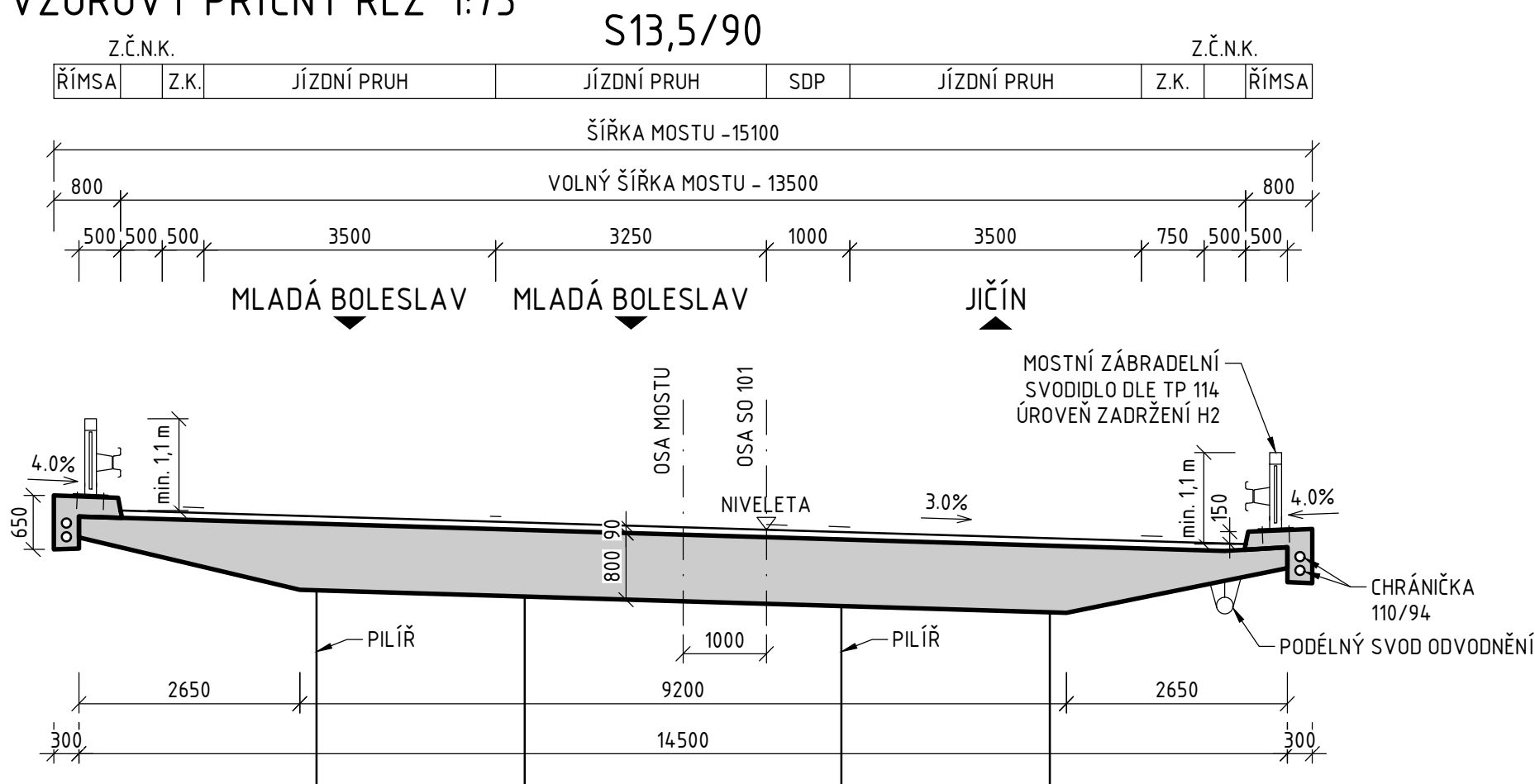
VZOROVÝ PŘÍČNÝ ŘEZ 1:75
