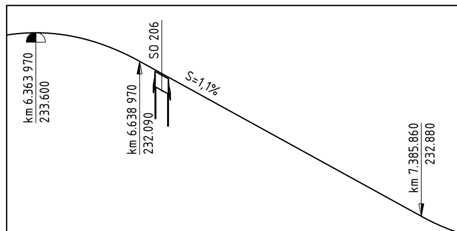
VÝŠKOVÉ VEDENÍ SO 101
