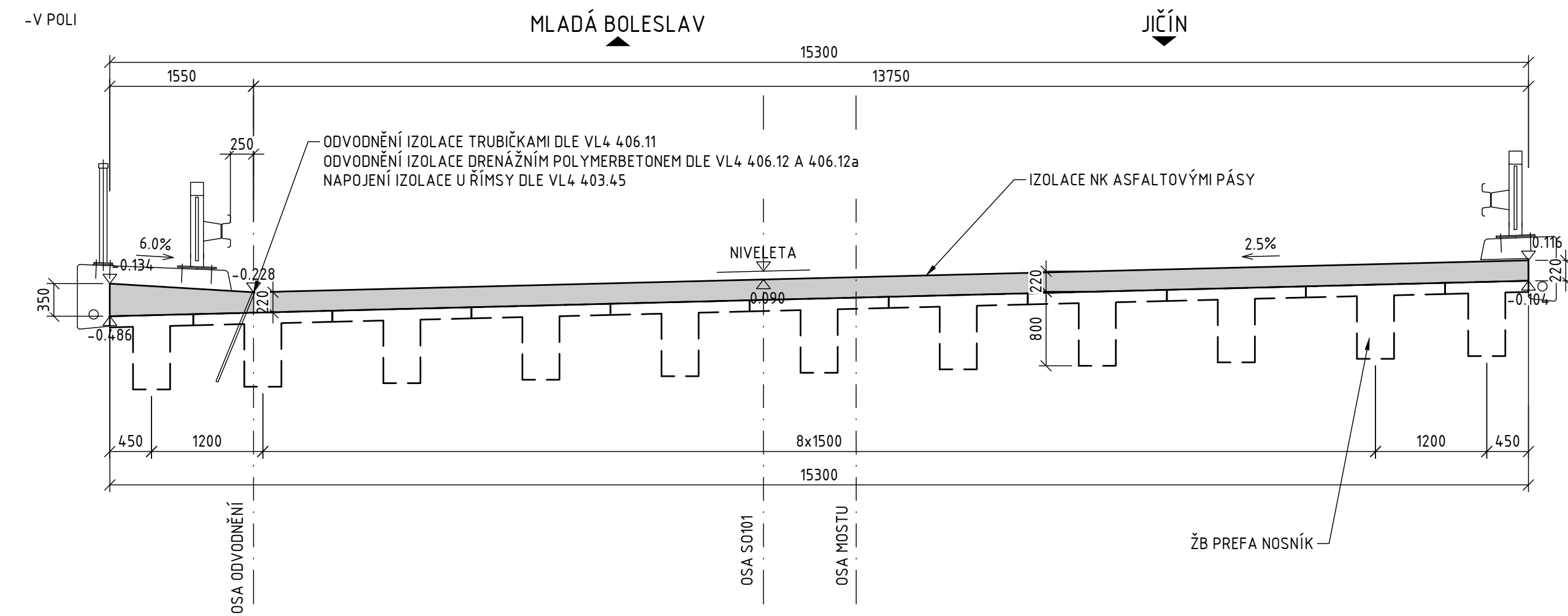
VZOROVÝ PŘÍČNÝ ŘEZ 1:50
