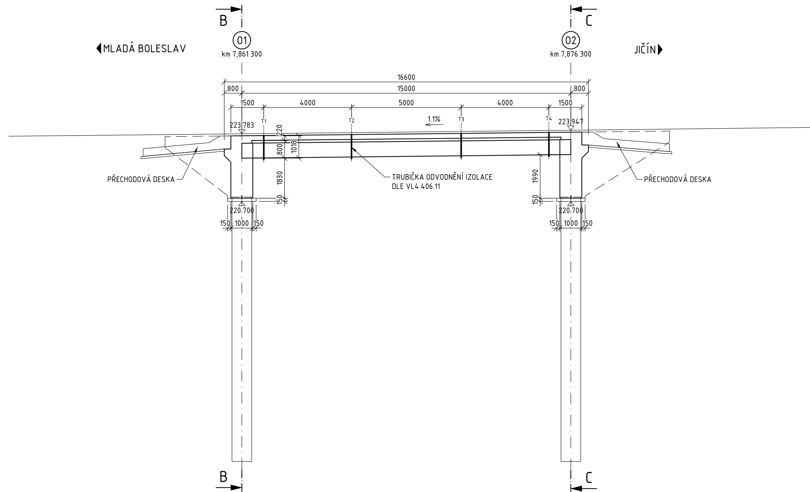
PODÉLNÝ ŘEZ 1:100
