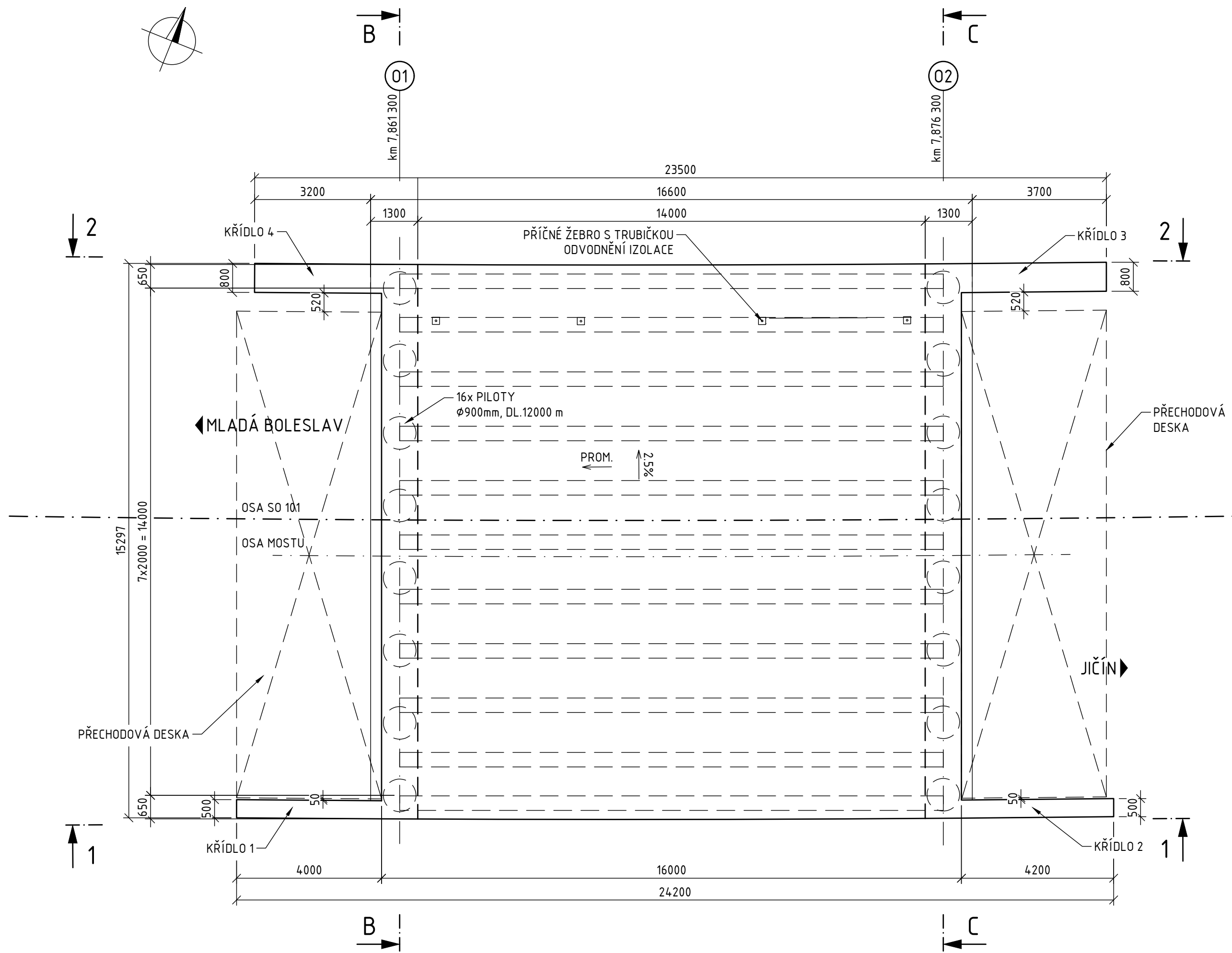
PŮDORYS 1:100
