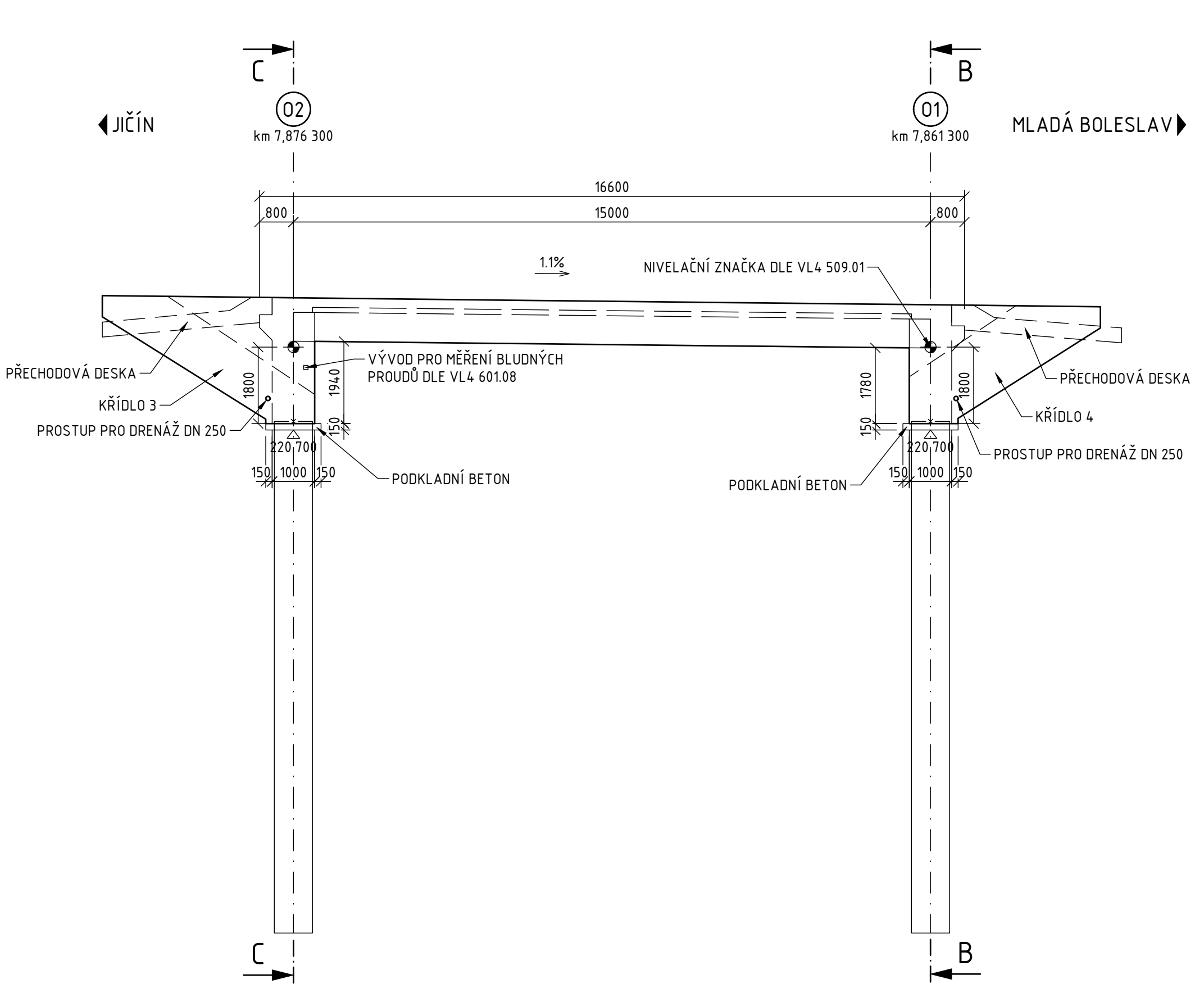
POHLED 2 1:100
