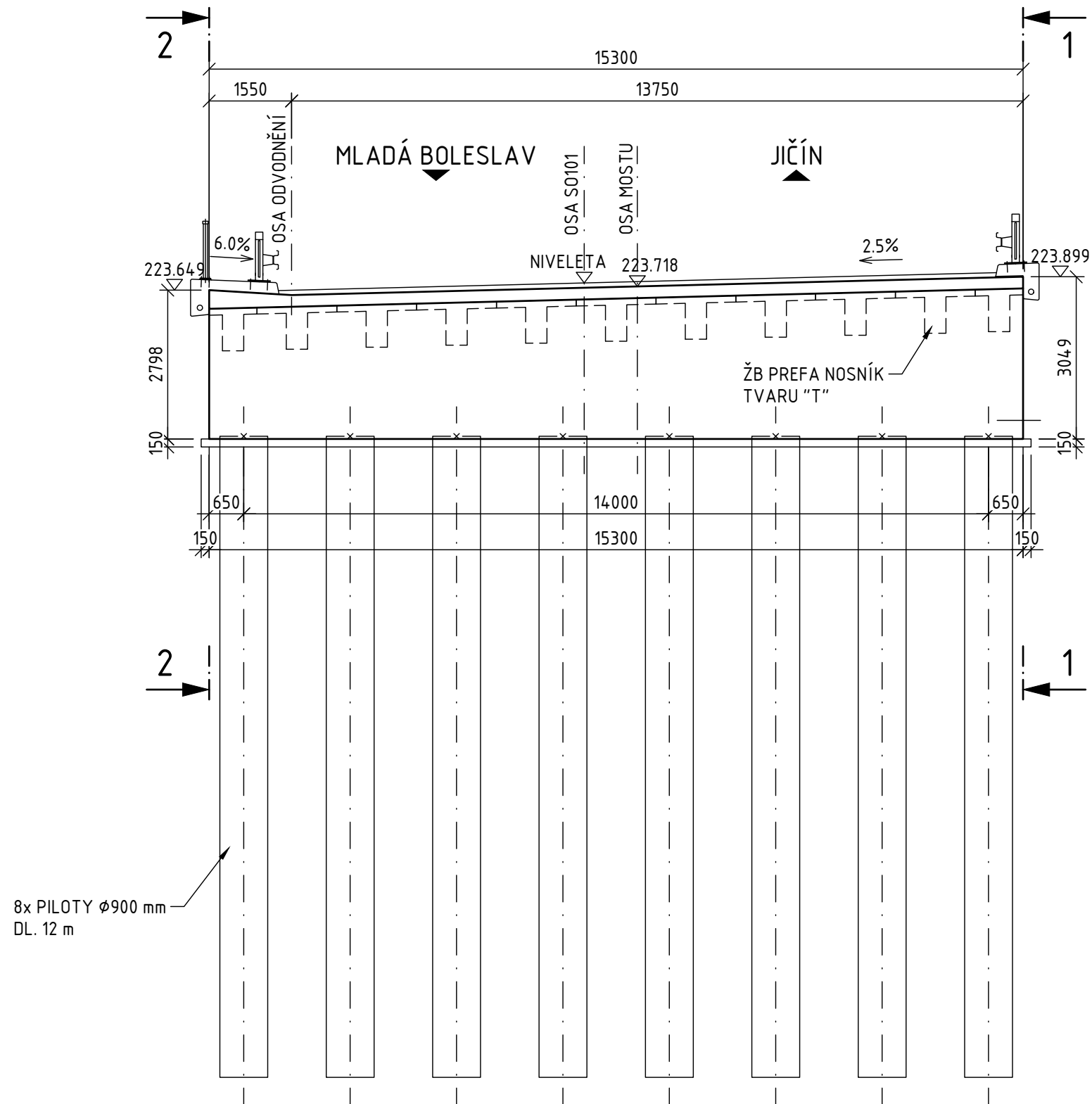
ŘEZ B-B 1:100
