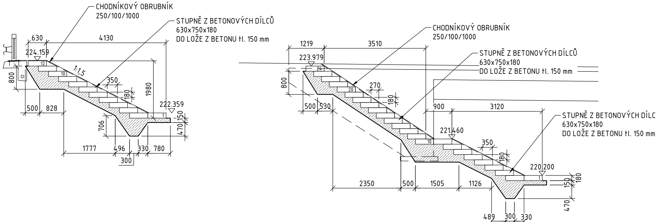
SCHODIŠTĚ 1 - PODÉLNÝ ŘEZ 1:75
