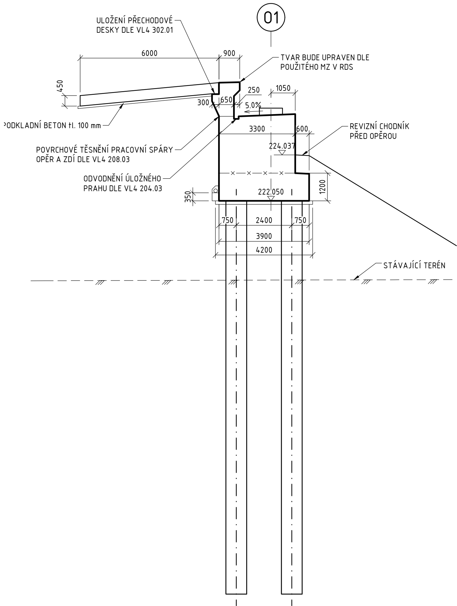
ŘEZ B-B 1:100, 01
