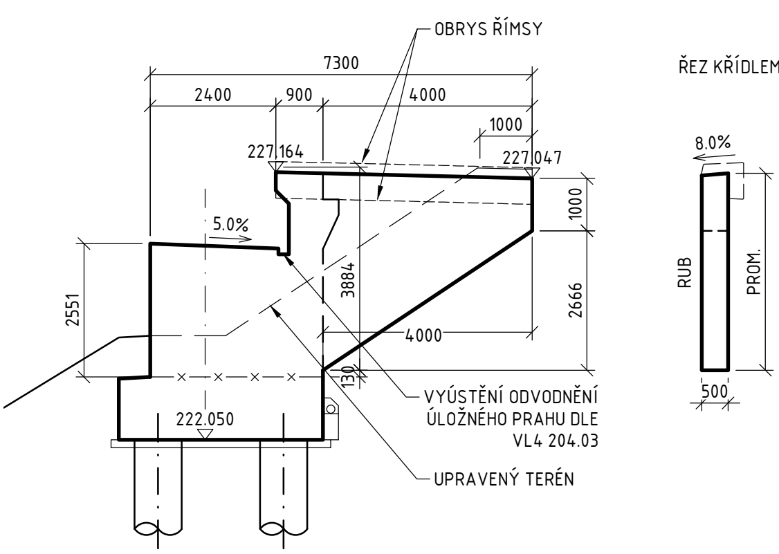
POHLED 1 1 : 100, 01
