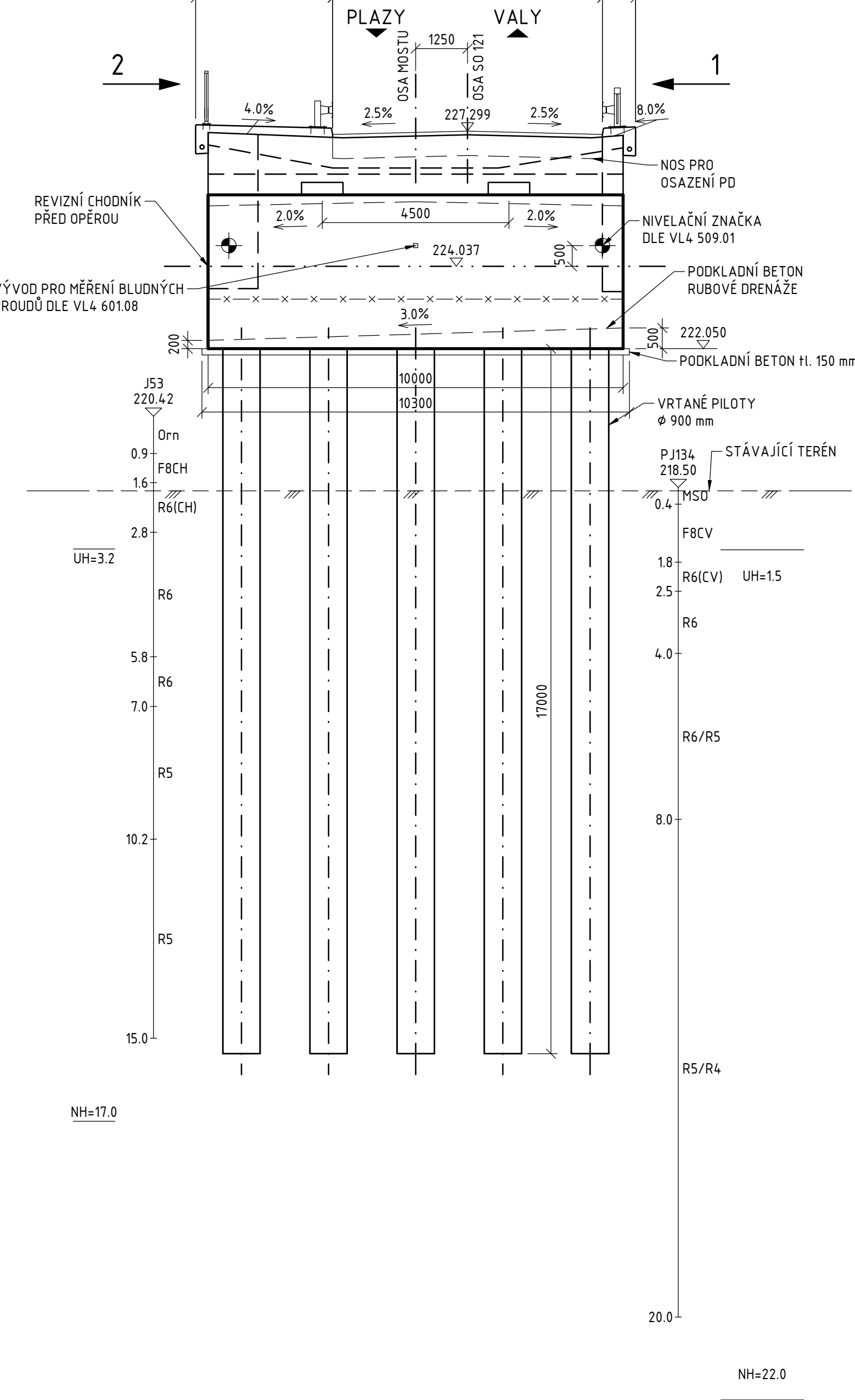
OPĚRA 01 ŘEZ A-A 1:100
