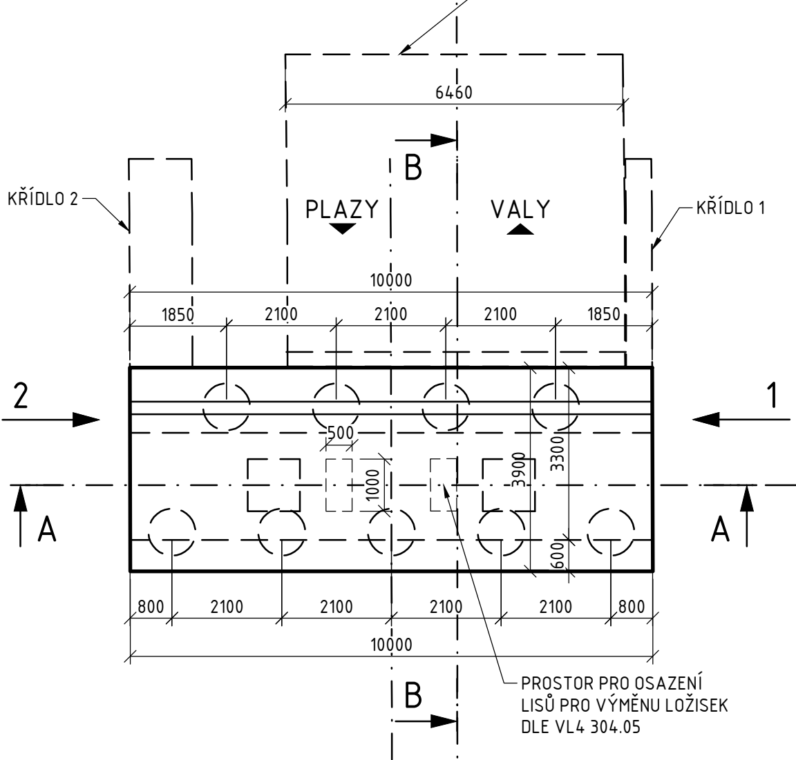
PŮDORYS ZÁKLADU 1 : 100
