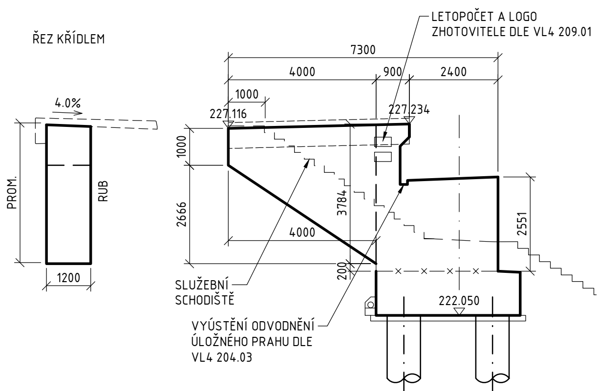
POHLED 2 1 : 100, 01
