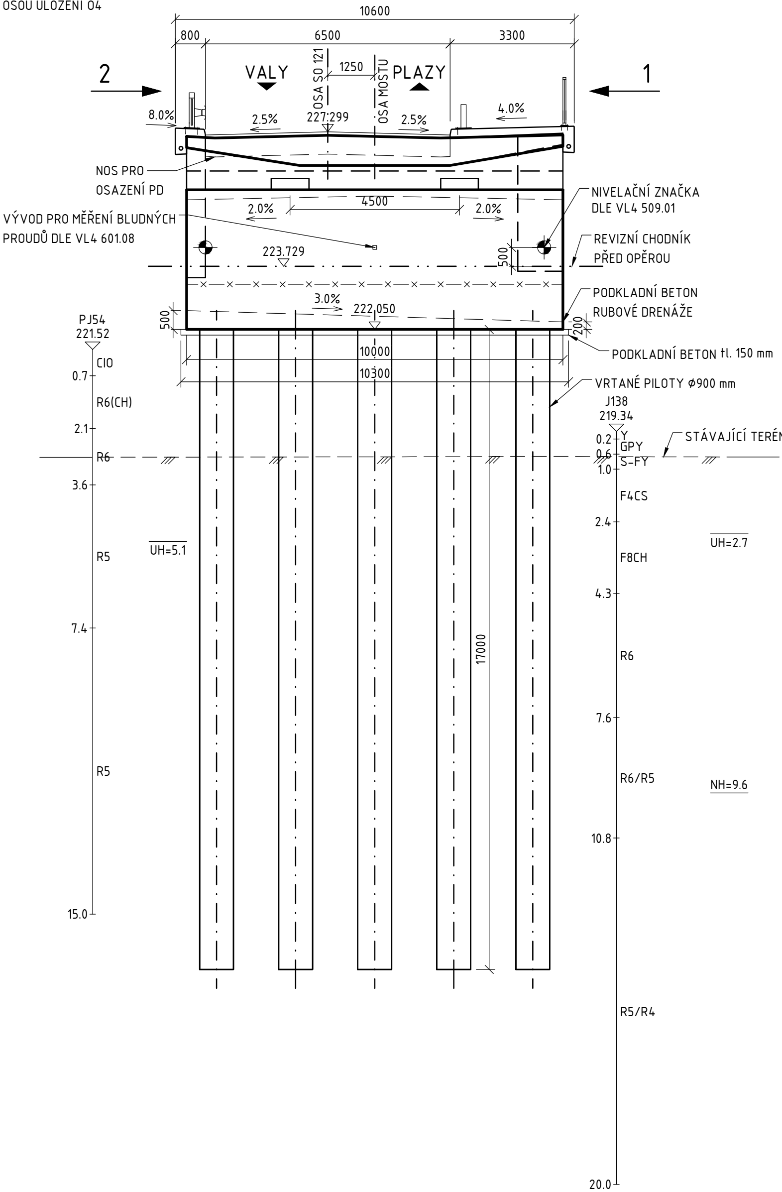
OPĚRA 04 ŘEZ A-A 1:100 OSOÚ ULOŽENÍ 04
