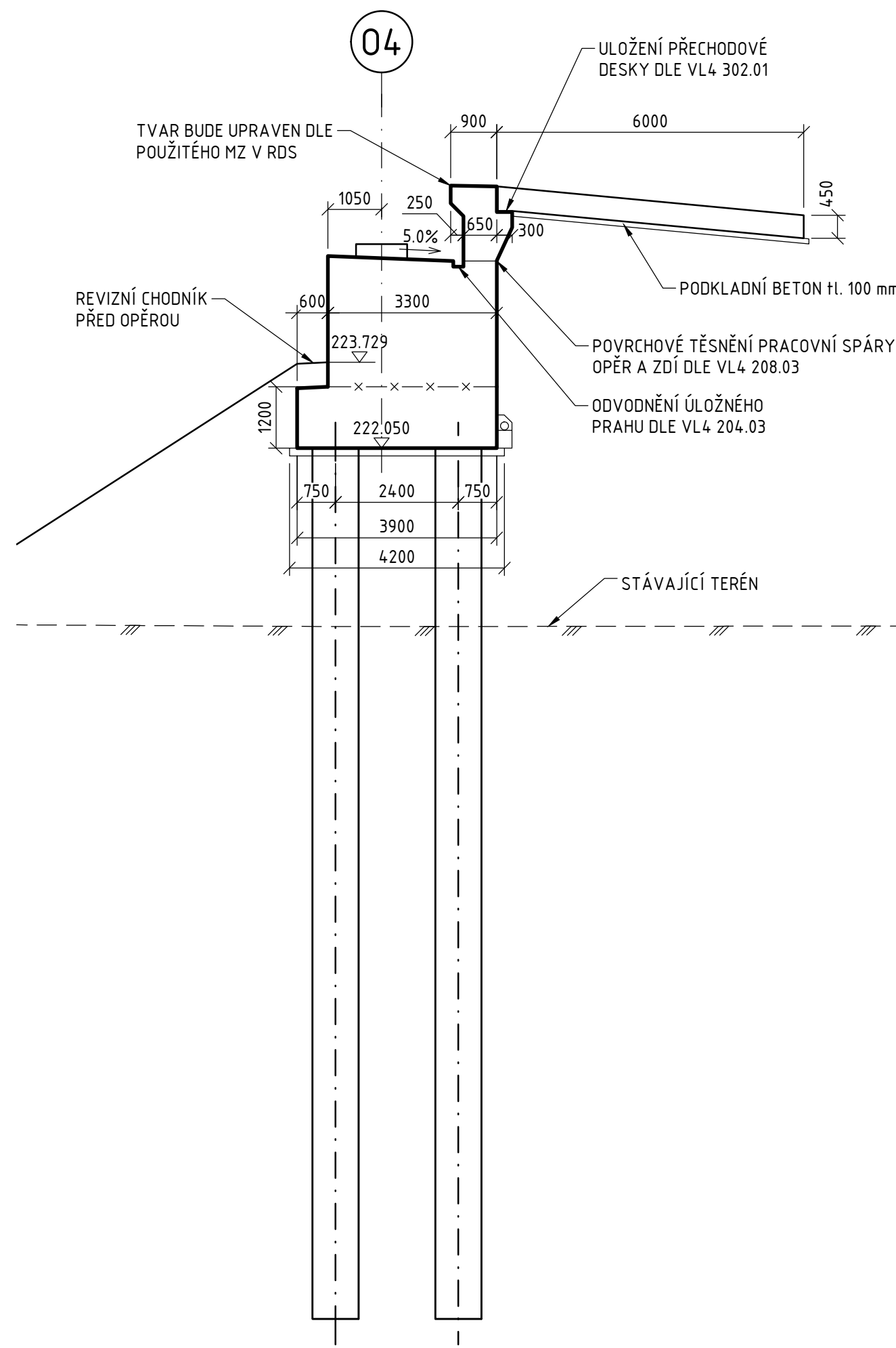
ŘEZ B-B 1:100, 04
