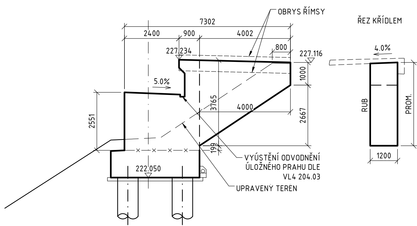
POHLED 1 1:100, 04
