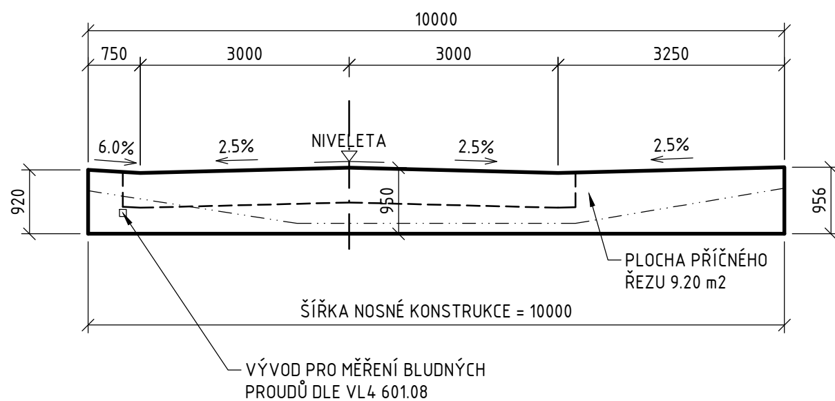
TVAR PŘÍČNÍKU V MÍSTĚ 04 1:75
