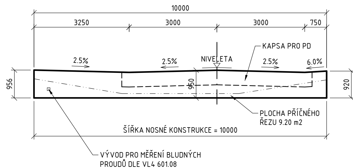
TVAR PŘÍČNÍKU V MÍSTĚ 01 1:75
