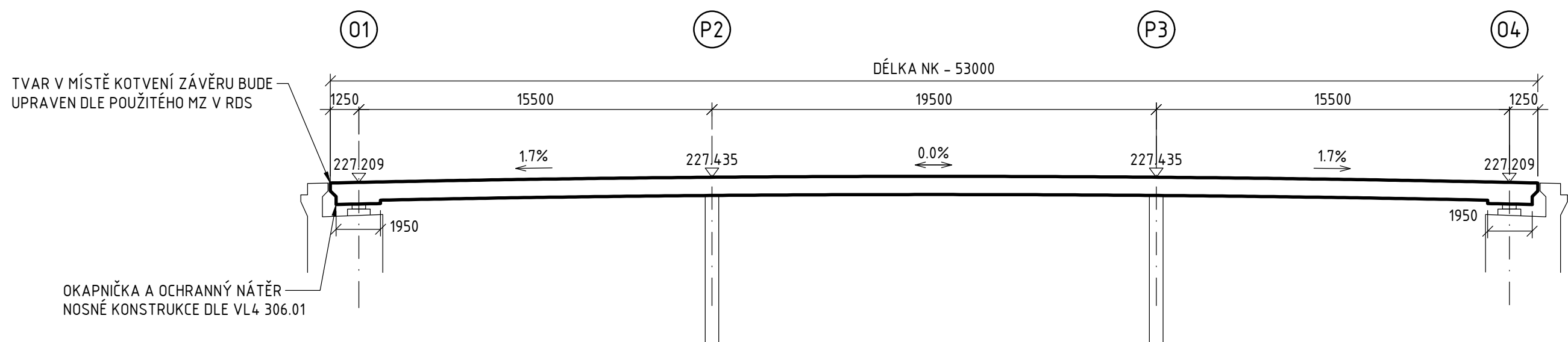
PODÉLNÝ ŘEZ 1:200
