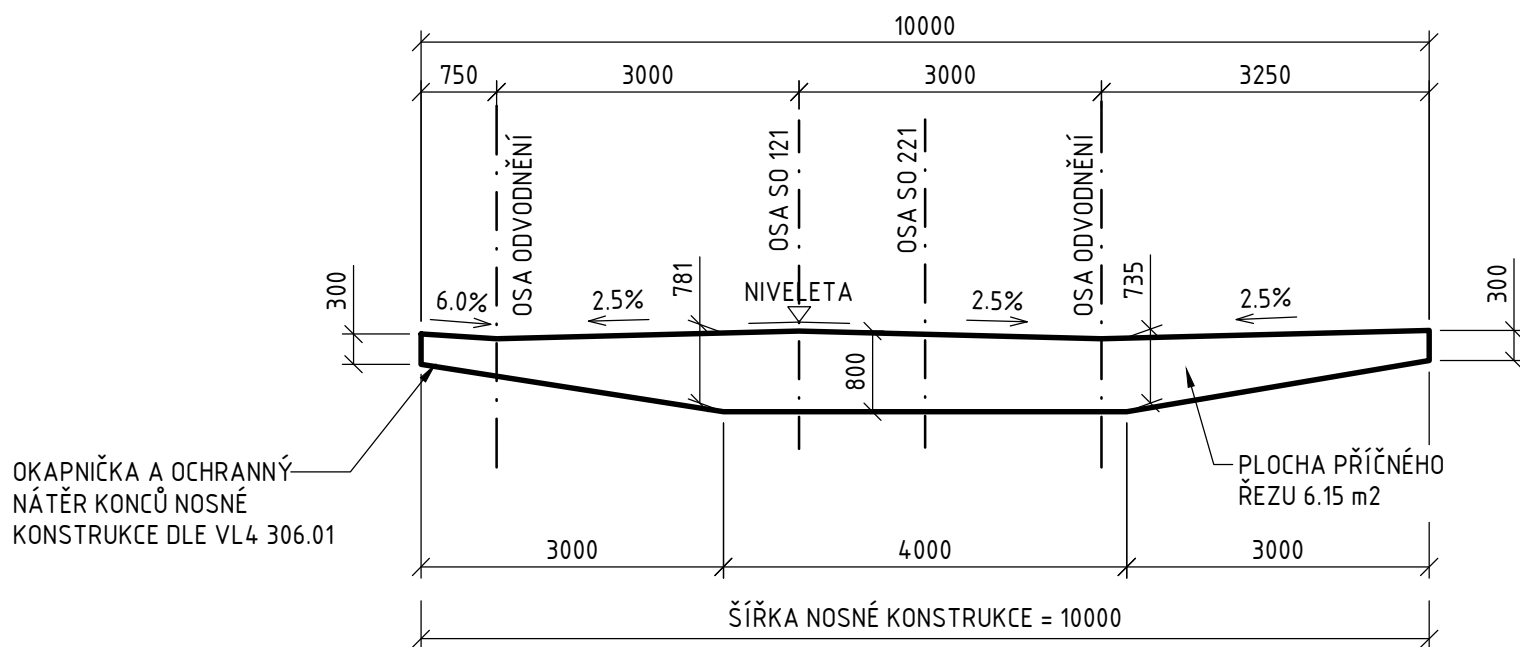
PŘÍČNÝ ŘEZ NK 1:75
